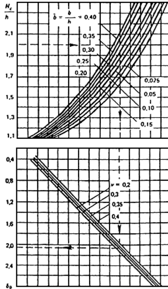
Номограмма для определения значений \delta_0
