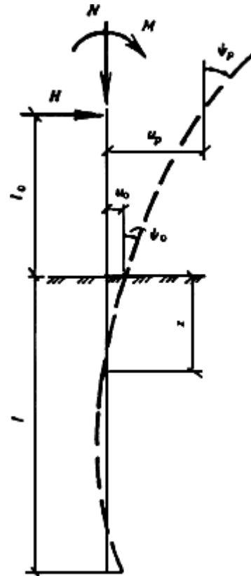
Схема нагрузок на сваю
