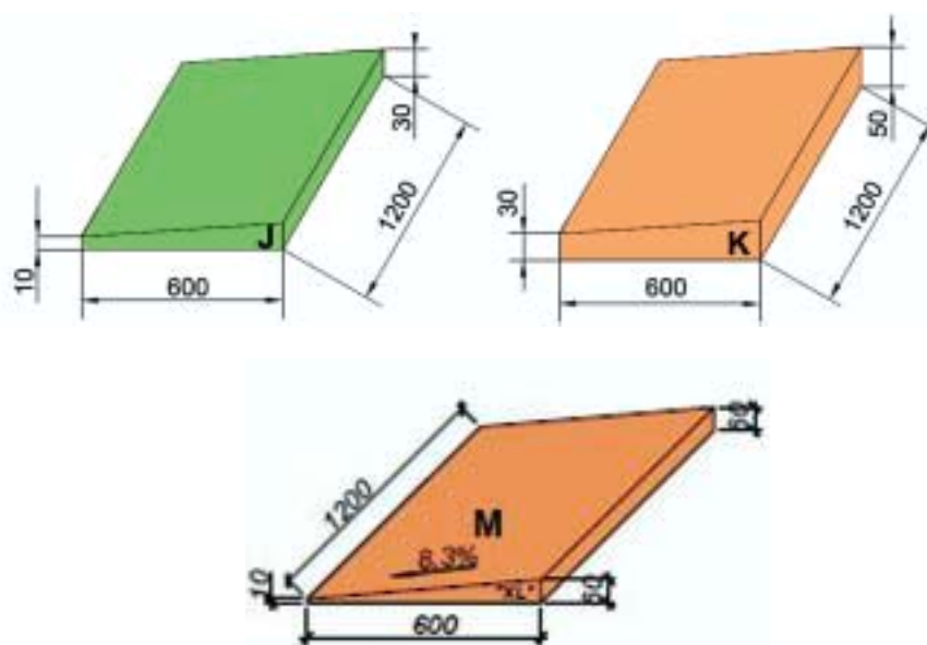
Рисунок Д.3 — Набор плит XPS ТЕХНИКОЛЬ CARBON PROF SLOPE и плит PIR SLOPE 3,4% и 8,3%
