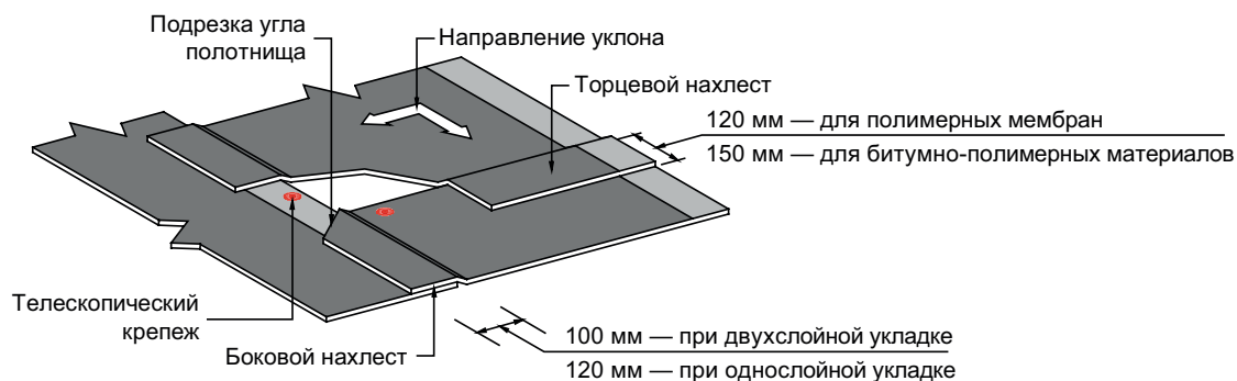
Рисунок Ж.7 — Нахлесты полотнищ рулонных материалов при механическом креплении
