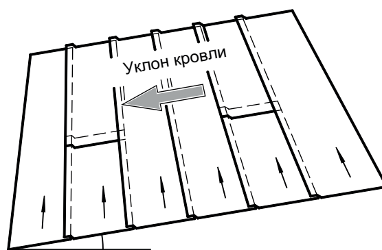
Рисунок Ж.2—Укладка материала на скате крыши перпендикулярно уклону
