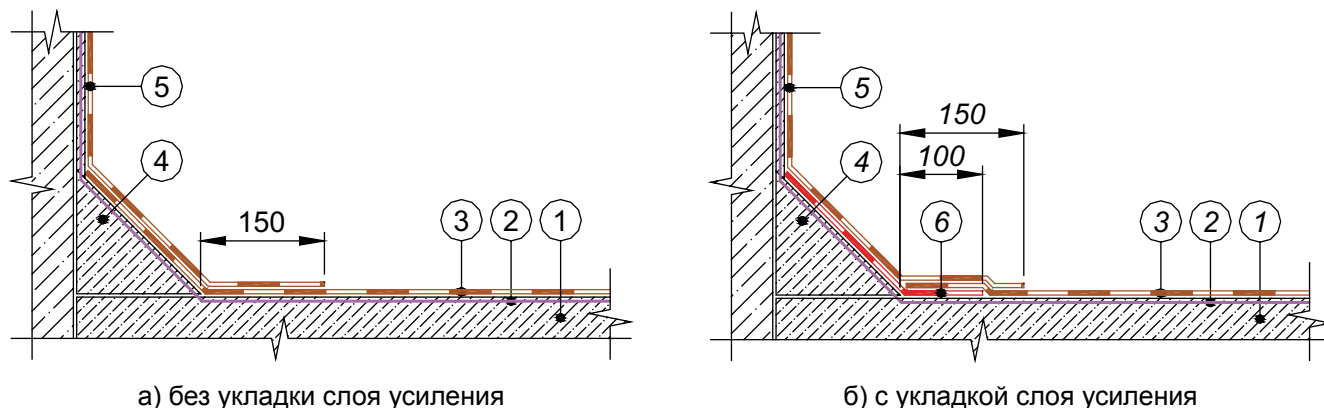
Рисунок М.6 — Варианты раскладки кровельного материала на переходном бортике при однослойной укладке
