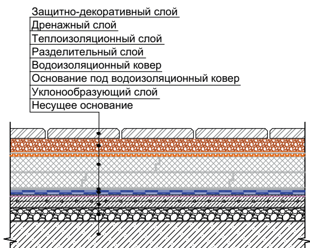
Рисунок 4.3 — Конструкция эксплуатируемой крыши под пешеходную нагрузку
