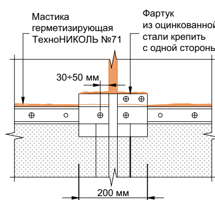
Рисунок М.12 — Краевая рейка на стене из бетонных плит
