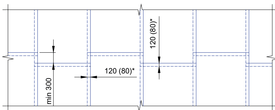
а) со смещением торцевых нахлестов
