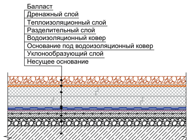
Рисунок 4.2 — Конструкция инверсионной крыши
