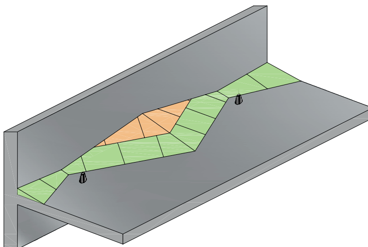
Рисунок Д.12 — Схема раскладки плит ТЕХНОРУФ Н30-КЛИН 4,2% при устройстве контруклона в парапетной зоне
