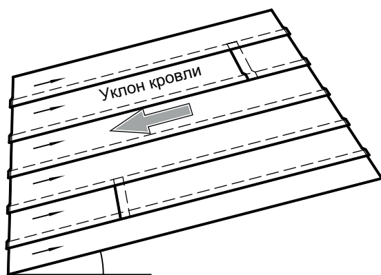
Рисунок Ж.1—Укладка материала на скате крыши параллельно уклону
