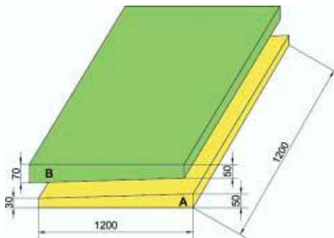
Рисунок Д.7 — Набор плит ТЕХНОРУФ Н30 КЛИН 1,7%
