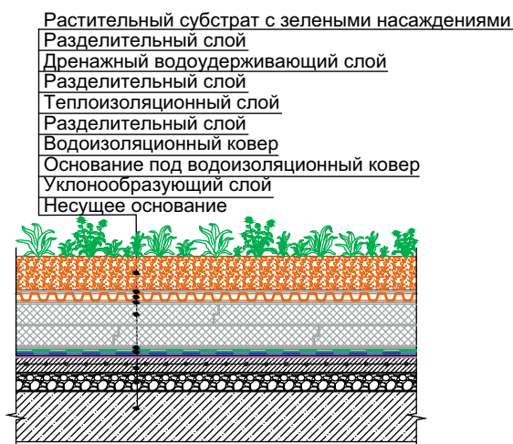
Рисунок 4.5 — Конструкция зеленой крыши
