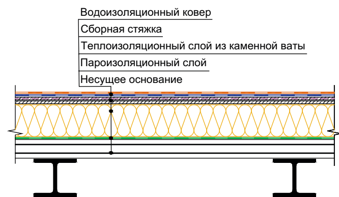
Рисунок 7.1 — Крыша с теплоизоляционным слоем из каменной ваты
