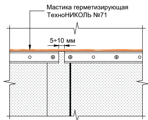
Рисунок М.9 — Зазор между краями соседних реек
