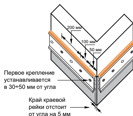
Рисунок М.10 — Установка краевой рейки на углу
