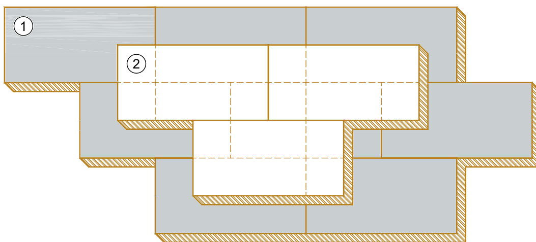
Рисунок Г.2 — Смещение плит верхнего и нижнего слоев при укладке
