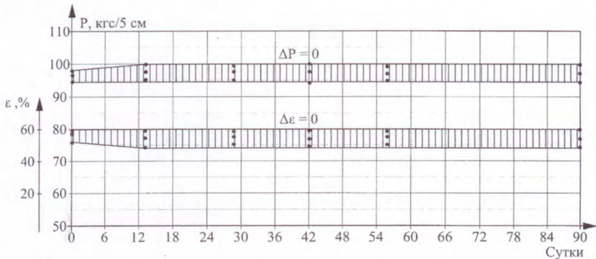
Рис. 1. Изменение прочности (1) и относительного удлинения (2) образцов рулонного материала "Техноэласт ЭПП" при воздействии 15-% раствора NaOH
