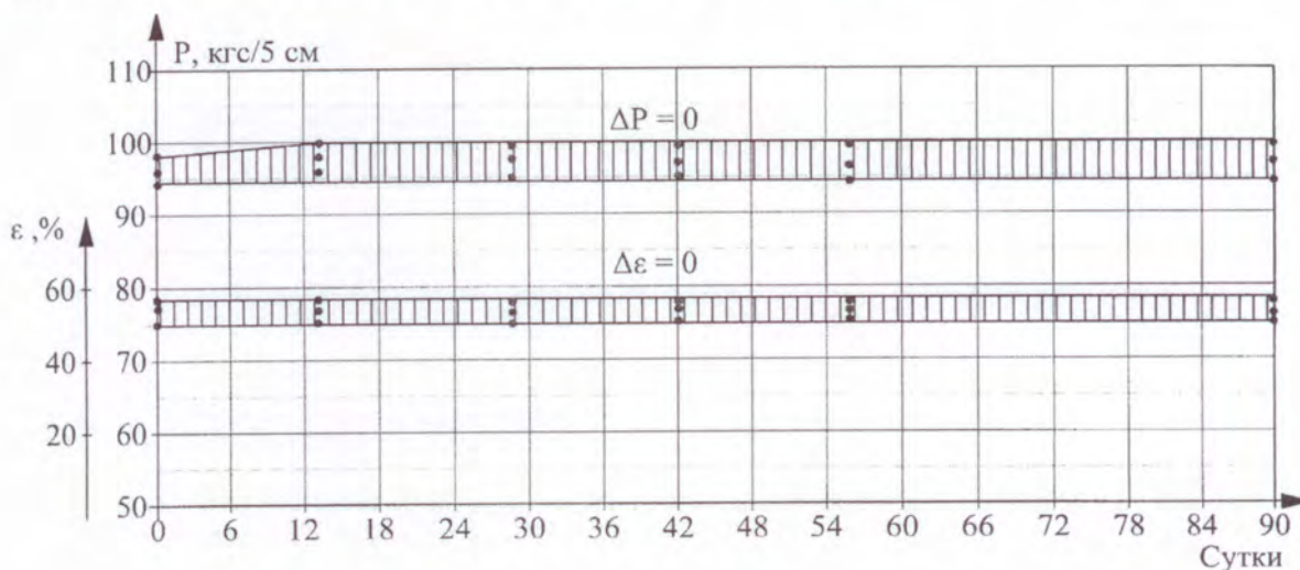
Рис. 3. Изменение прочности (1) и относительного удлинения (2) образцов материала "Техноэласт ЭПП" при воздействии насыщенного раствора NaCl
