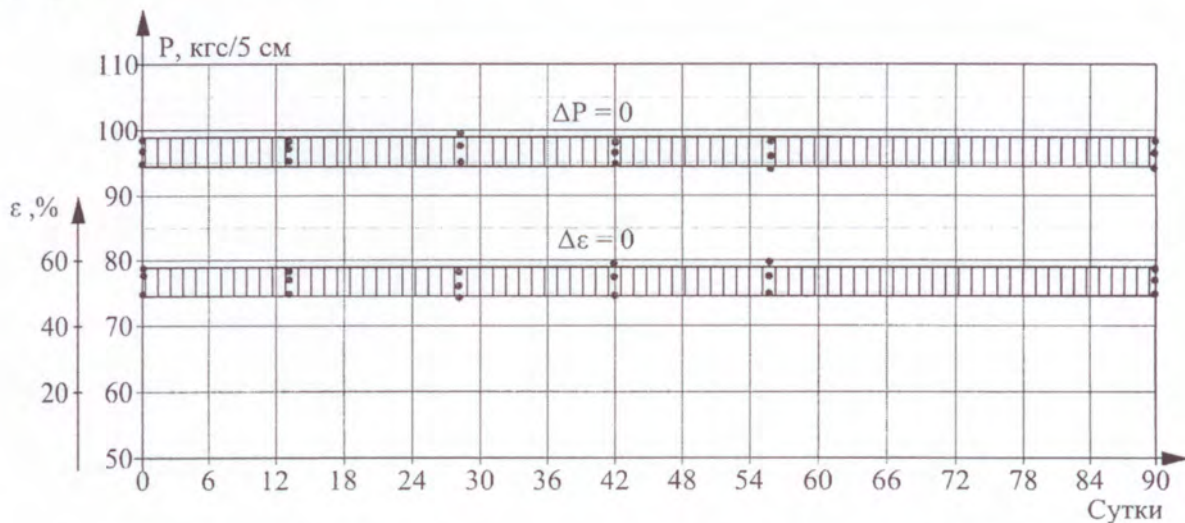
Рис. 2. Изменение прочности (1) и относительного удлинения (2) образцов рулонного материала "Техноэласт ЭПП" при воздействии 15-% раствора H 2 SO 4
