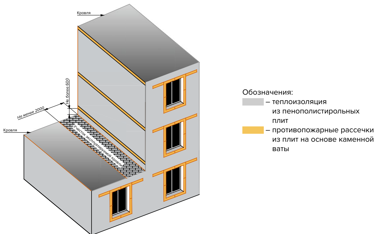
Рисунок 10 – Примыкание СФТК к участку эксплуатируемой кровли.
