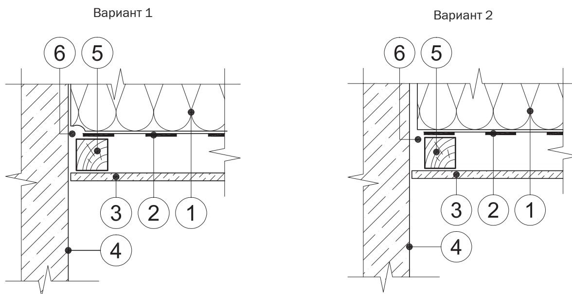
1 — теплоизоляционный слой; 2 — пароизоляционный слой; 3 — внутренняя отделка; 4 — стена; 5 — деревянный брус; 6 — деформационная складка
