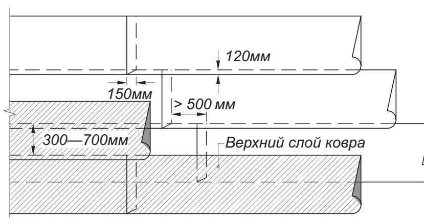
Рисунок Л.2 — Смещение полотнищ гидроизоляционных материалов в смежных слоях
