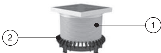
1 — водосливный трап 2 — дренажное кольцо Д2
