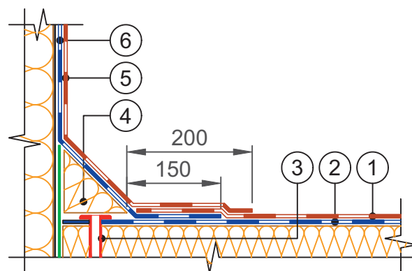
1 — верхний слой водоизоляционного ковра; 2 — нижний слой водоизоляционного ковра; 3 — телескопический крепежный элемент ТЕХНОНИКОЛЬ; 4 — ТЕХНОРУФ В 60 ГАЛТЕЛЬ; 5 — верхний слой водоизоляционного ковра на вертикальной поверхности; 6 — нижний слой водоизоляционного ковра на вертикальной поверхности
