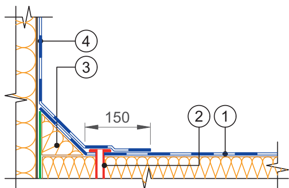
1 — кровельный ковер; 2 — телескопический крепежный элемент ТЕХНОНИКОЛЬ; 3 — ТЕХНОРУФ В 60 ГАЛТЕЛЬ; 4 — кровельный ковер на вертикальной поверхности
