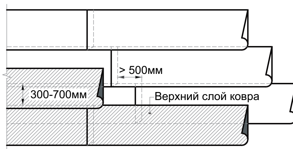
Рисунок Е.4 — Смещение полотнищ кровельного материала в смежных слоях
