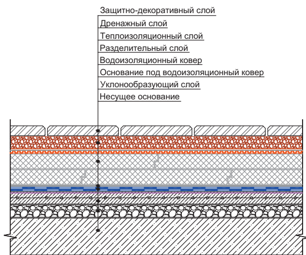
Рисунок 4.3 — Конструкция инверсионной эксплуатируемой крыши
