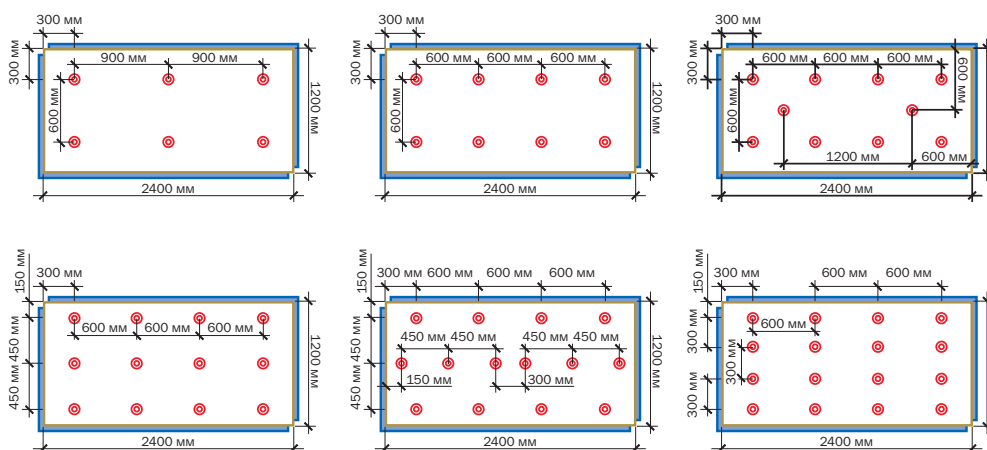
Рисунок 7.5 — Схема крепления теплоизоляционных плит из пенополиизоцианурата при индукционном способе крепления полимерной мембраны
