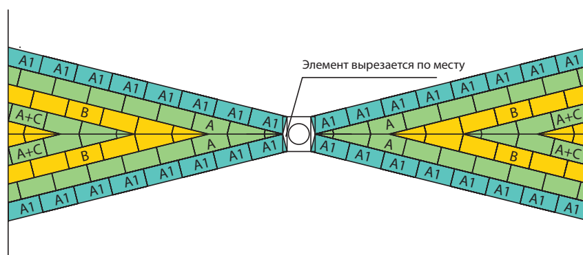
Рисунок Д.17 — Схема раскладки плит ТЕХНОРУФ Н30 КЛИН 4,2 % при создании уклонообразующего слоя в ендове
