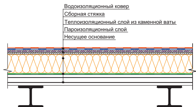
Рисунок 7.1 — Крыша с теплоизоляционным слоем из каменной ваты
