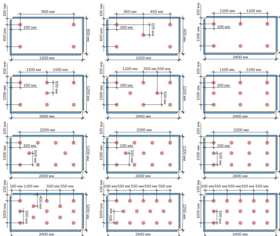
Рисунок 7.4 — Схема крепления теплоизоляционных плит из пенополиизоцианурата
