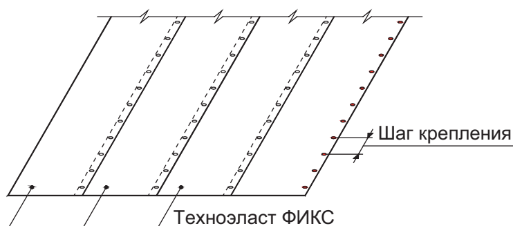
Рисунок Е.11 — Стандартная схема установки крепежа
