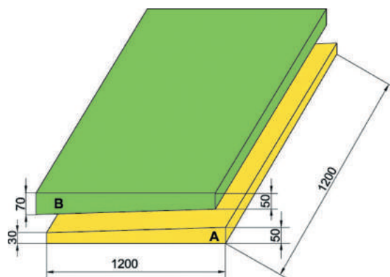
Рисунок Д.13 — Набор плит ТЕХНОРУФ Н30 КЛИН 1,7%
