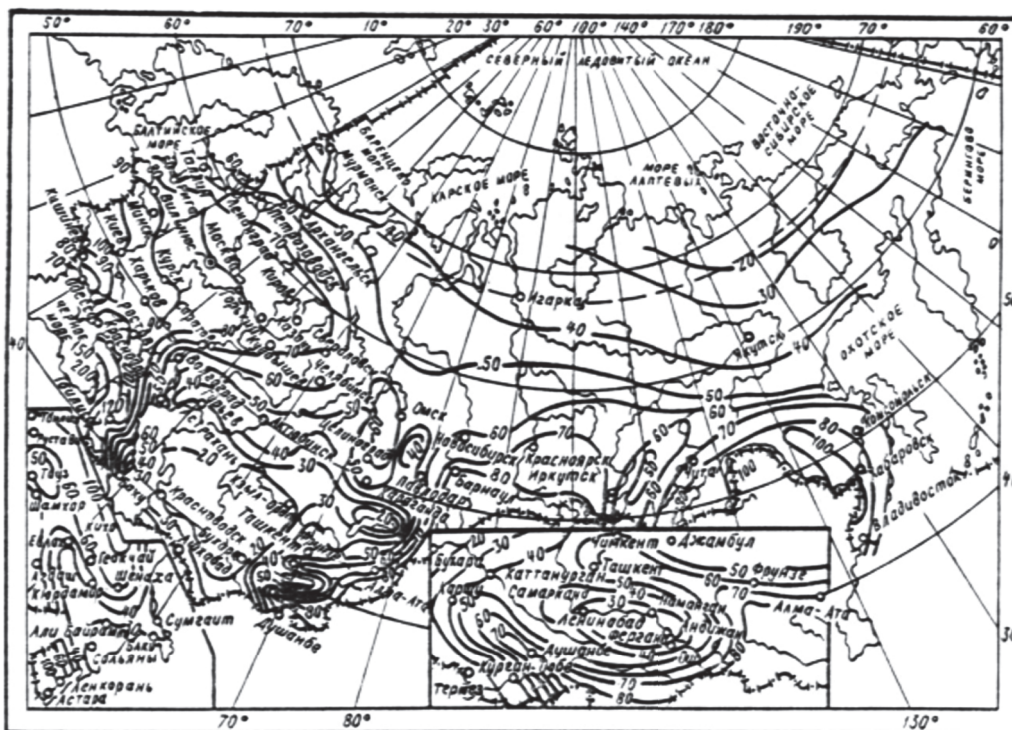
Рисунок И.1 — Значения величин интенсивности дождя q_{20}
