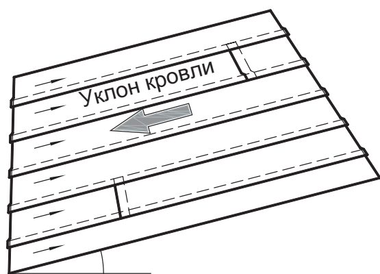
Рисунок Е.2 — Укладка материала на скате крыши параллельно уклону
