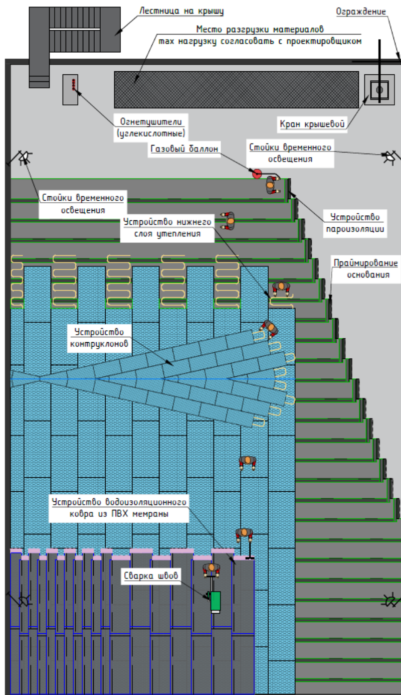
Рис. 5.1. Схема организации рабочего места
