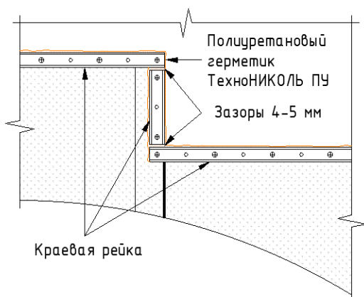
Рис. 5.28 Обрамление края кровельного ковра краевой рейкой
