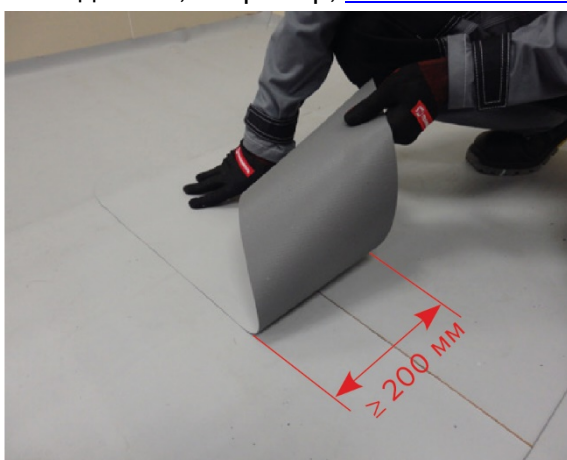
Рис. 5.14 Соединение стыков рулонов ПВХ-мембран с флисовой подложки при помощи ПВХ-мембраны без флисовой подложки
