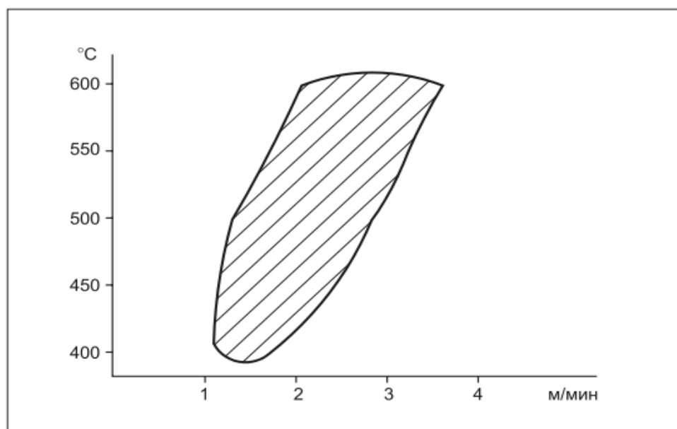
Рис. 5.16 Область сварки ПВХ мембран
