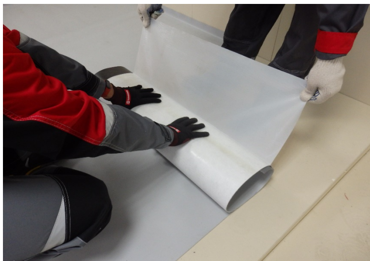
Рис. 5.13 Удаление анти-адгезионной пленки полимерной мембраны LOGICROOF V-GR FB SA
