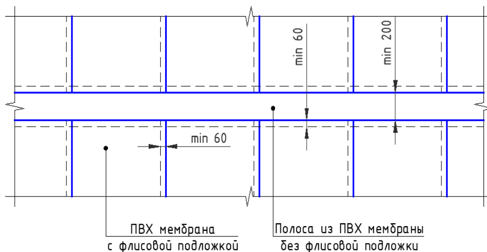
Рис. 5.9 Соединение стыков рулонов ПВХ-мембран с флисовой подложкой при помощи ПВХ-мембраны без флисовой подложки
