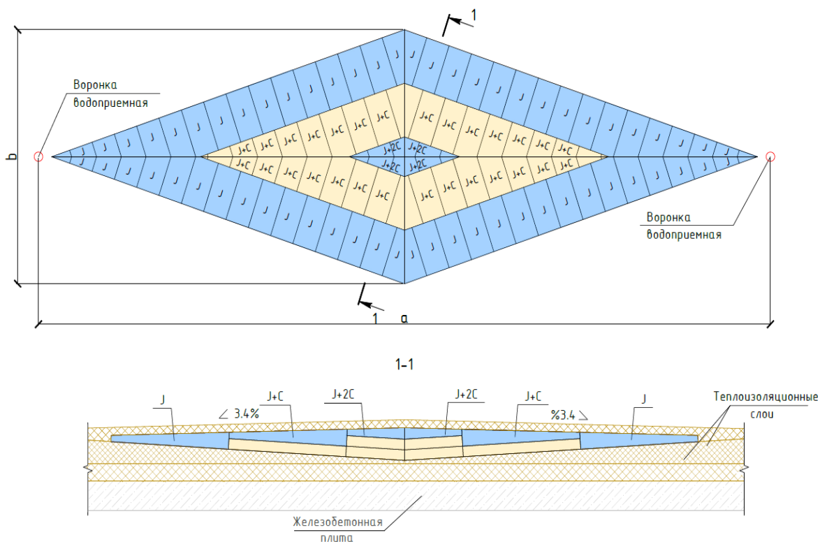
Рис. 5.6. Пример раскладки плит при создании уклона между воронками из плит LOGICPIR SLOPE с уклоном 3,4%
