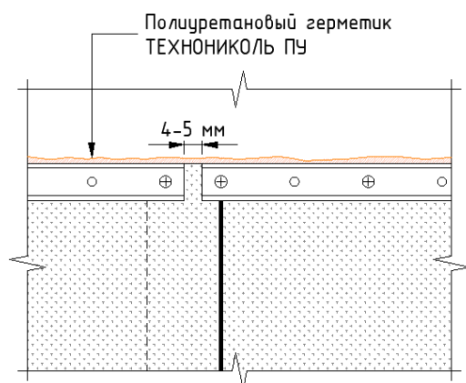
Рис. 5.26 Зазор между краями соседних реек
