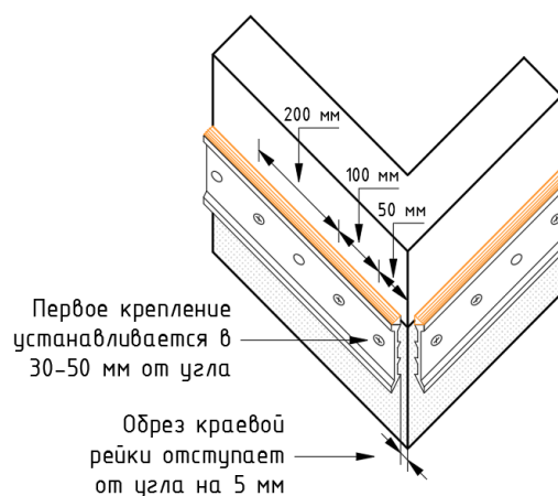
Рис. 5.27 Установка краевой рейки в угловой зоне
