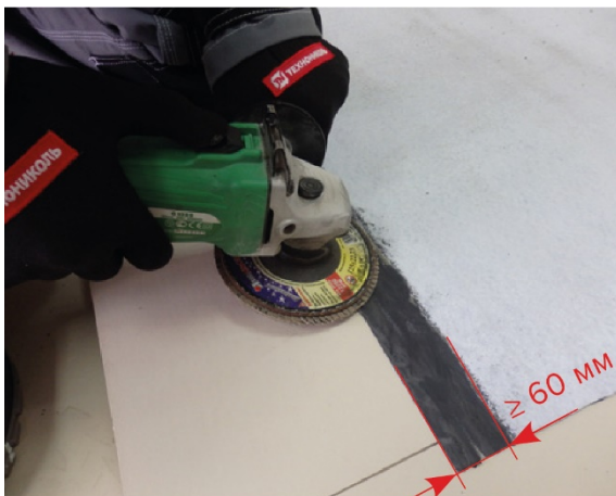
Рис. 5.15 Очистка краев полимерной мембраны от флиса и сварка стыков
