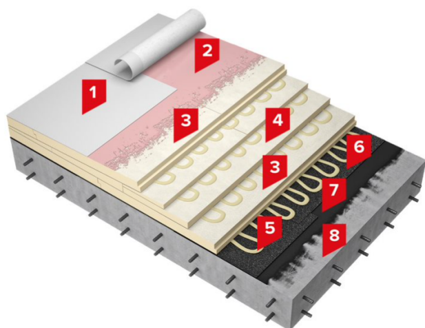
Рис. 3.1. Состав системы ТН-Кровля Эксперт PIR
