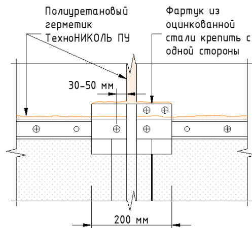
Рис. 5.29 Краевая рейка на стене из бетонных плит
