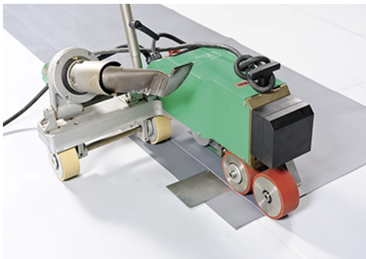
Рис. 5.20 Приварка полосы из полимерной мембраны
