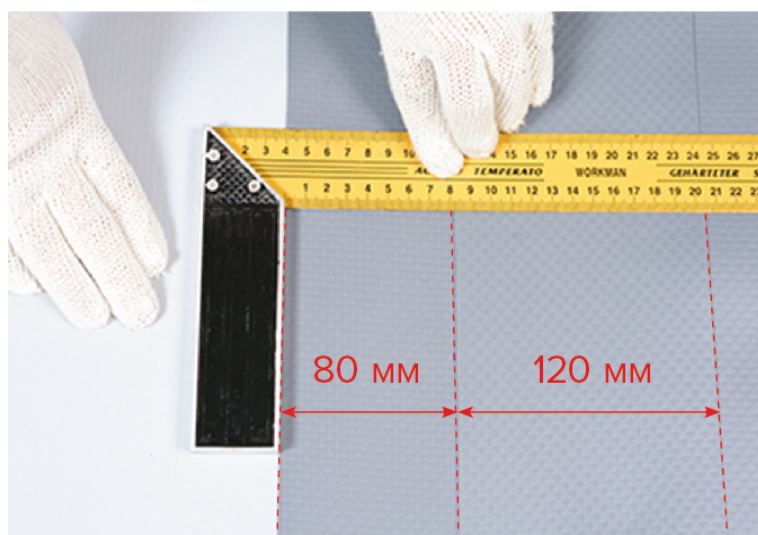
Рис. 5.18 Подбор ширины полотна полимерной мембраны для заведения на парапет
