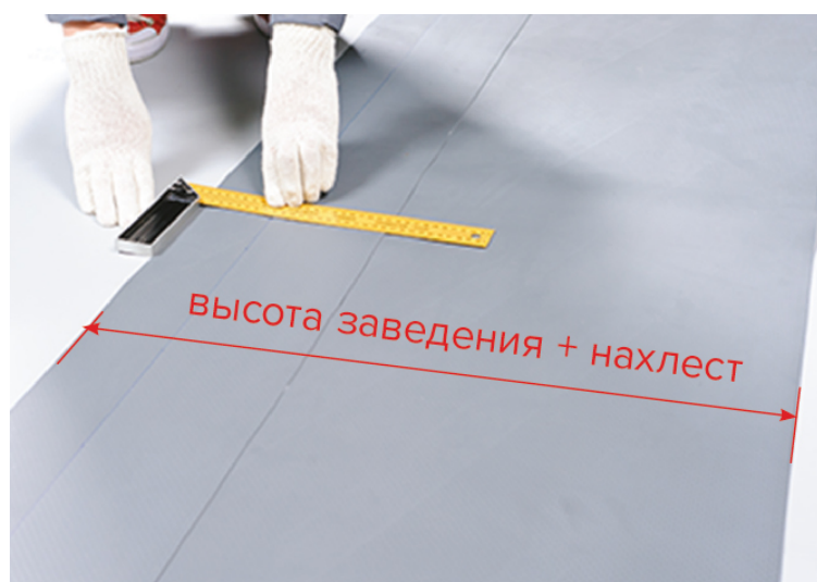
Рис. 5.17 Подготовка полотна полимерной мембраны для заведения на парапет
