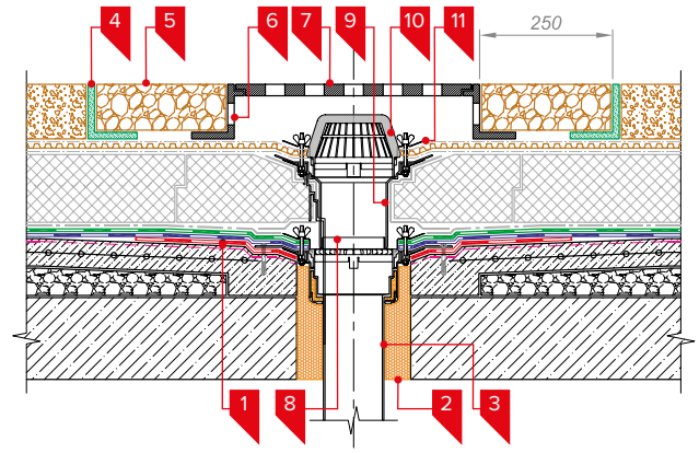
Рис. 3.53. Примыкание к воронкам в эксплуатируемых крышах
