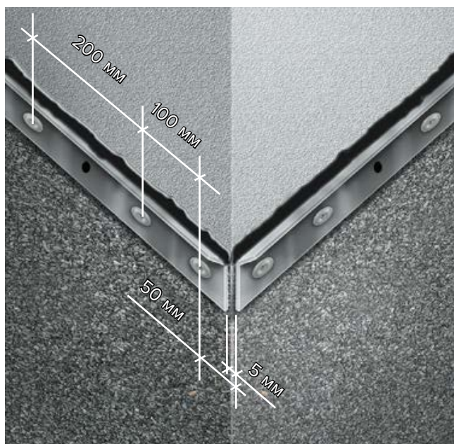
Рис. 3.22. Крепление краевой рейки
