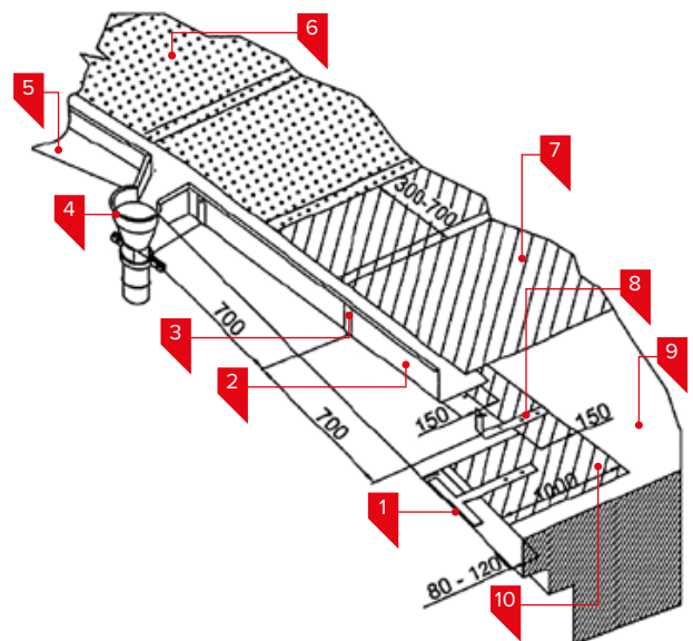
Рис. 3.54. Настенный водосточный желоб
