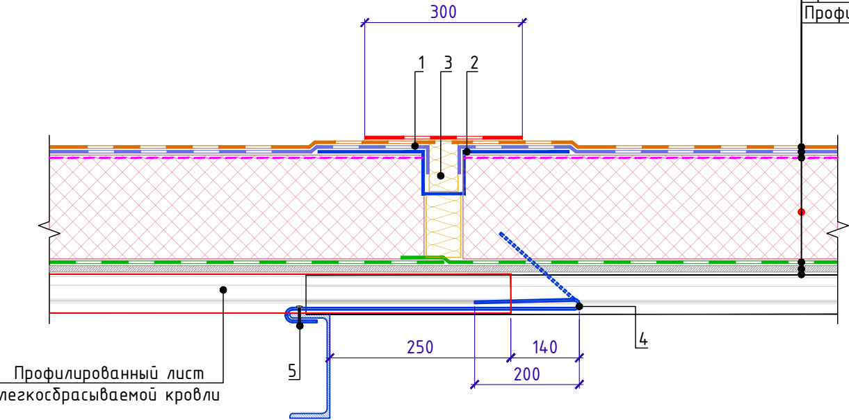
Сечение А-А
