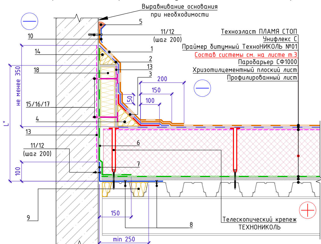
Спецификация на узел У.3.2-2025.02
