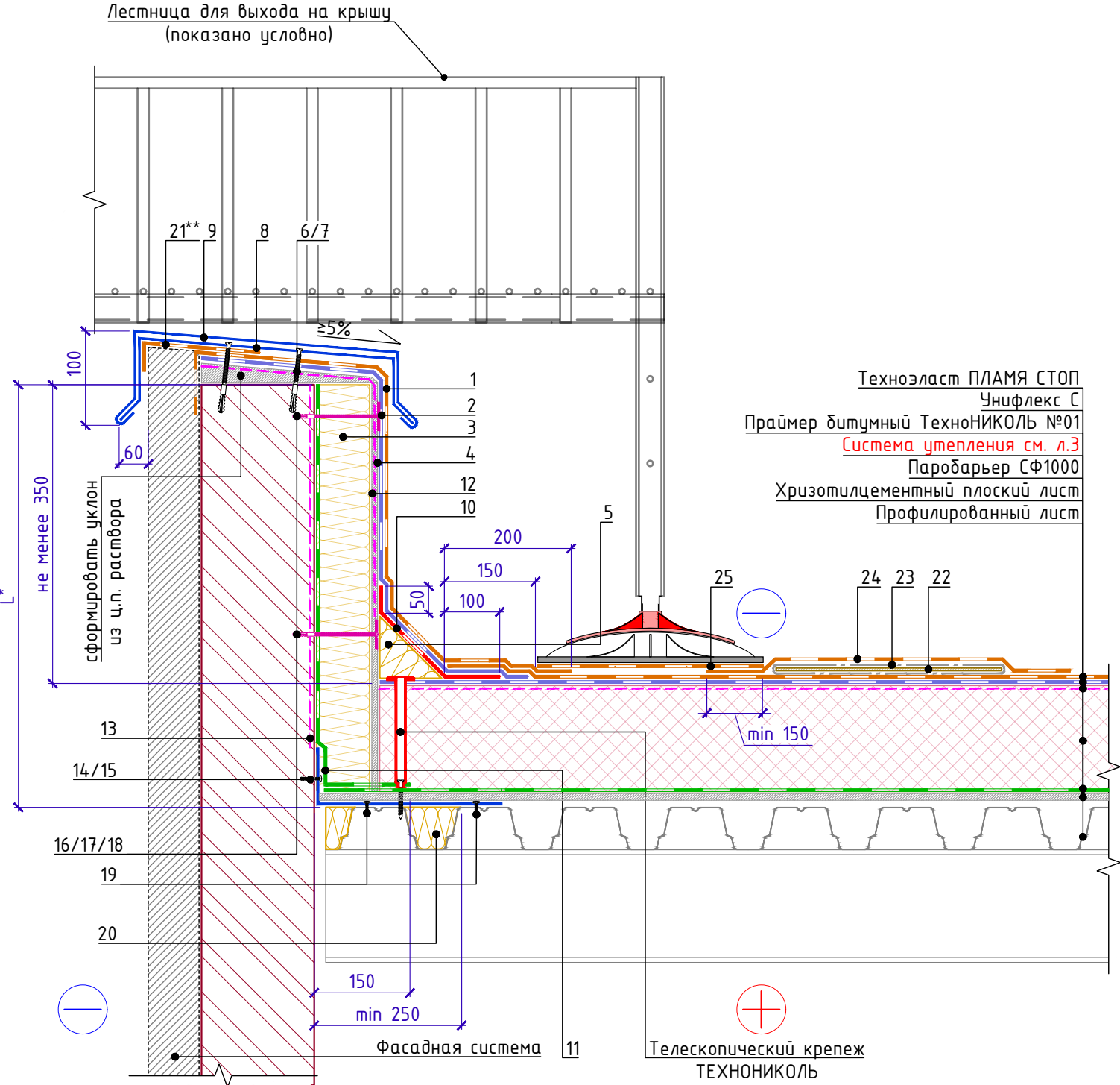
Крепежный элемент Позиция 8
