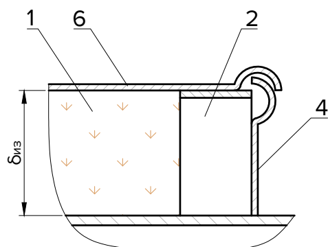
Заглушка металлическая
