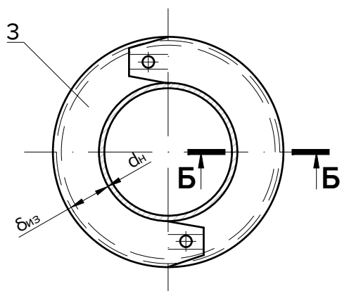
Диафрагма тип II
