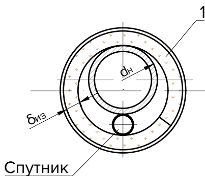
A - A со спутником
