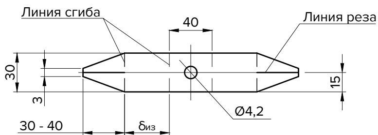
Развертка шплинта
