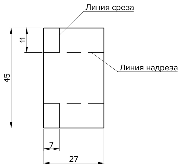
Заготовка пряжки
