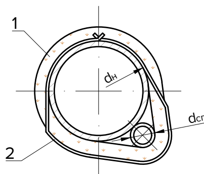
Б - Б при прокладке спутника сбоку
