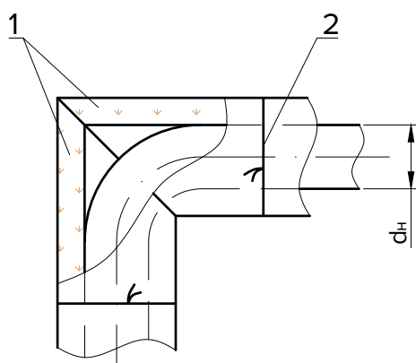
Вариант для отводов d н от 18 до 57 мм
