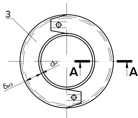
Диафрагма тип I
