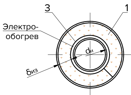
A - A с электрообогревом
