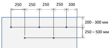
Рис. 3. Установка крепежа вдоль карнизного свеса (схематичный рисунок)
