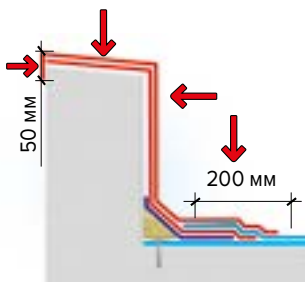
Кровля с мех. фиксацией нижнего слоя
