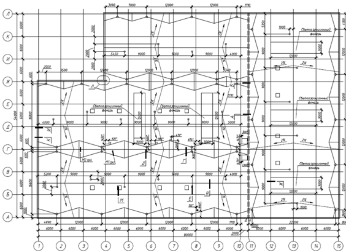
План кровли
