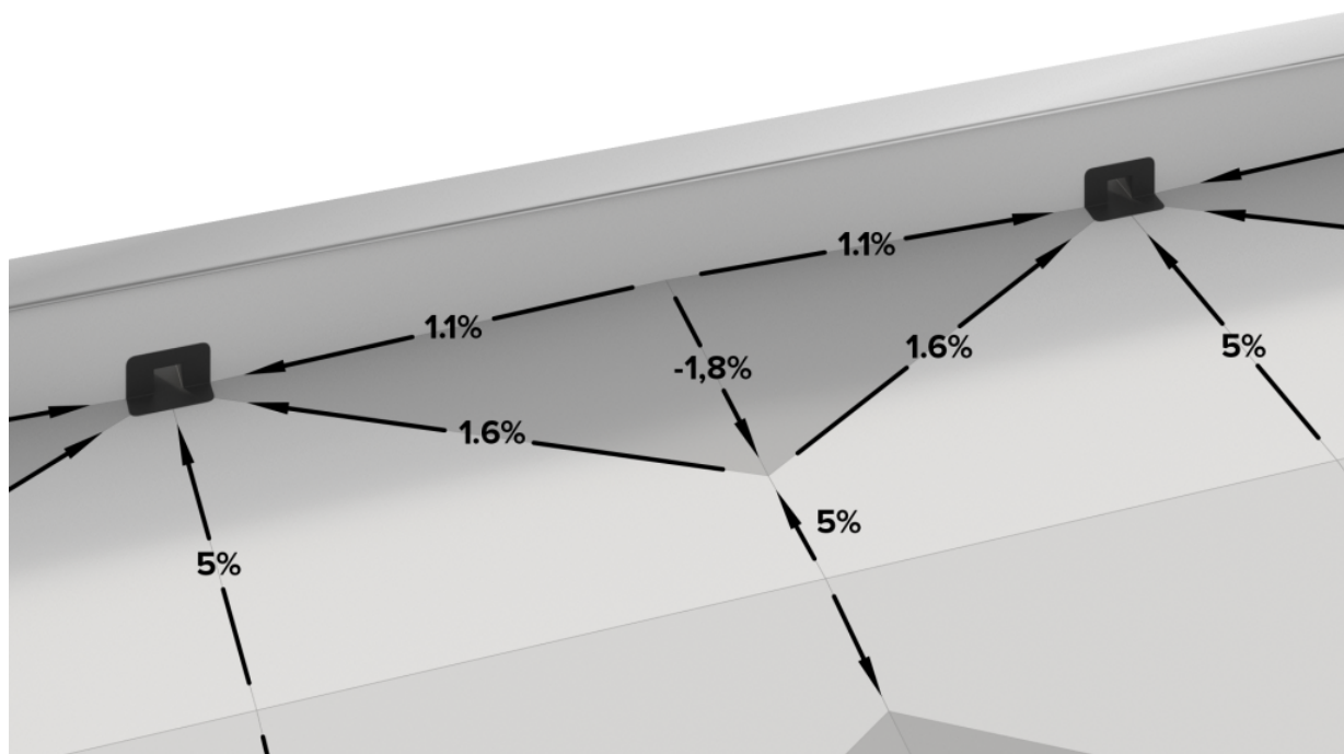
Рисунок 13. Контруклон между парапетными воронками.
