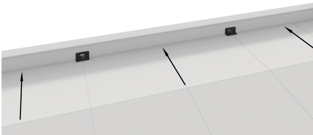
Рисунок 12. Ендова располагается у парапета, воронки находятся в парапете.
