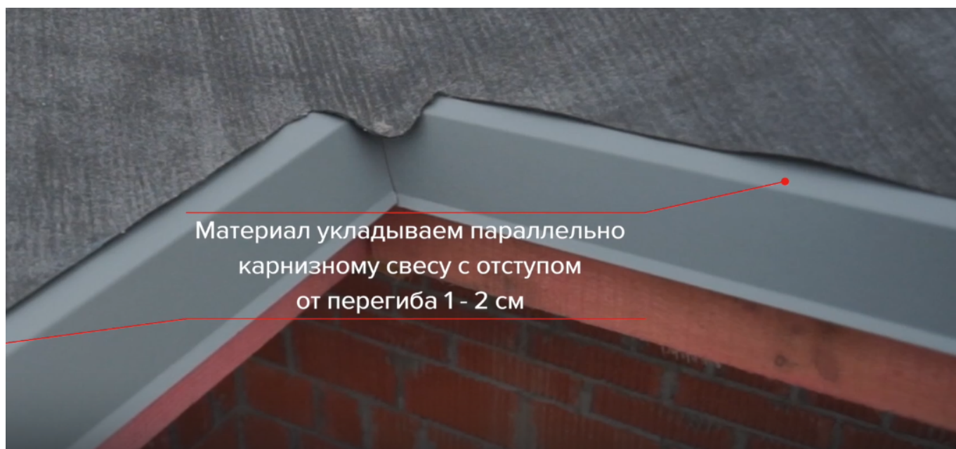
Серия 9: Монтаж гибкой черепицы ТЕХНОНИКОЛЬ SHINGLAS
