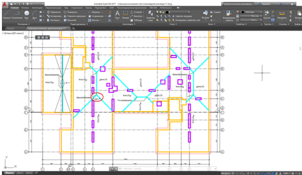
Рисунок 15. Формирование основного уклона.
