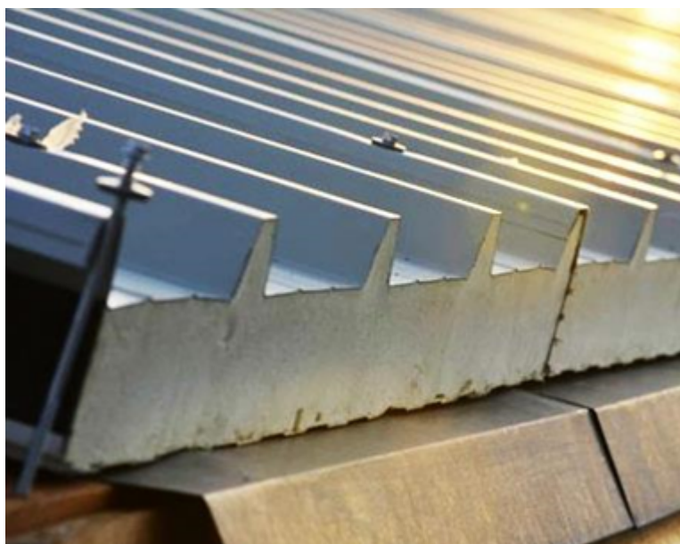
Комплексные сэндвич панели
