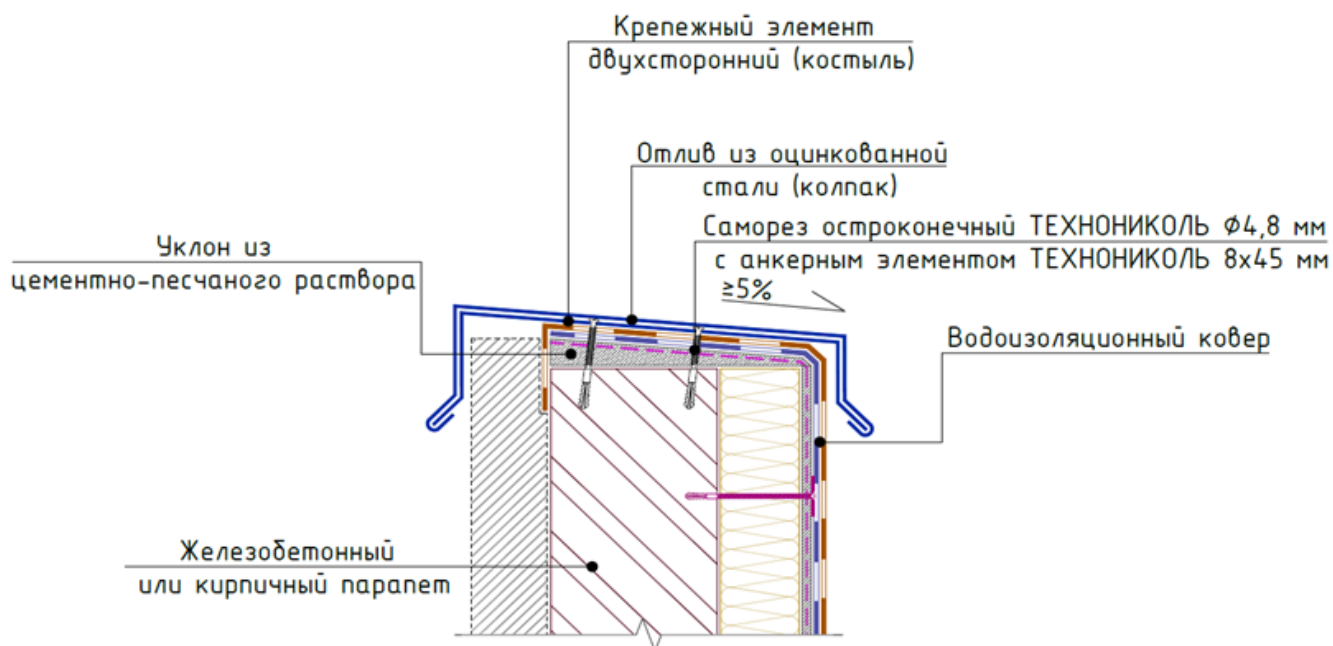
Рисунок 3. Крепление отлива из оцинкованной стали к верхней части парапета
