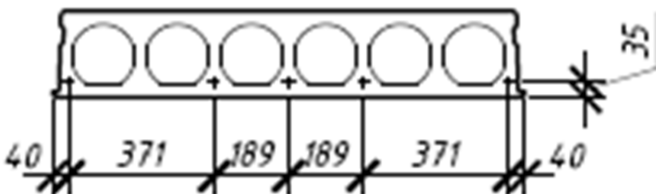
Рисунок 3. Расчетное сечение многопустотной плиты
