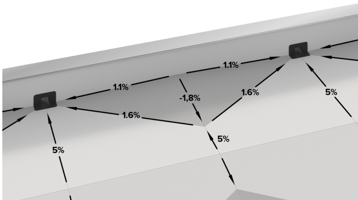
Рисунок 13. Контруклон между парапетными воронками.
