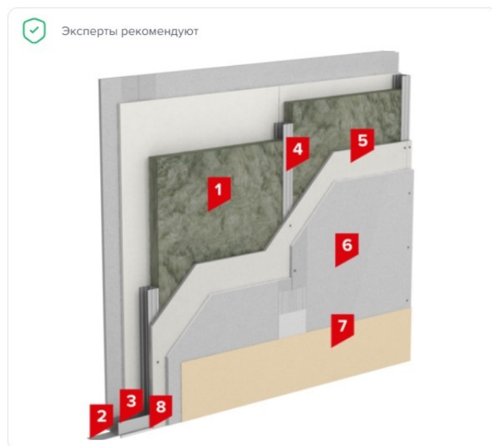
Рис. 1. Устройство каркасной звукоизоляционной перегородки для зонирования квартир, офисов, гостиничных номеров.
