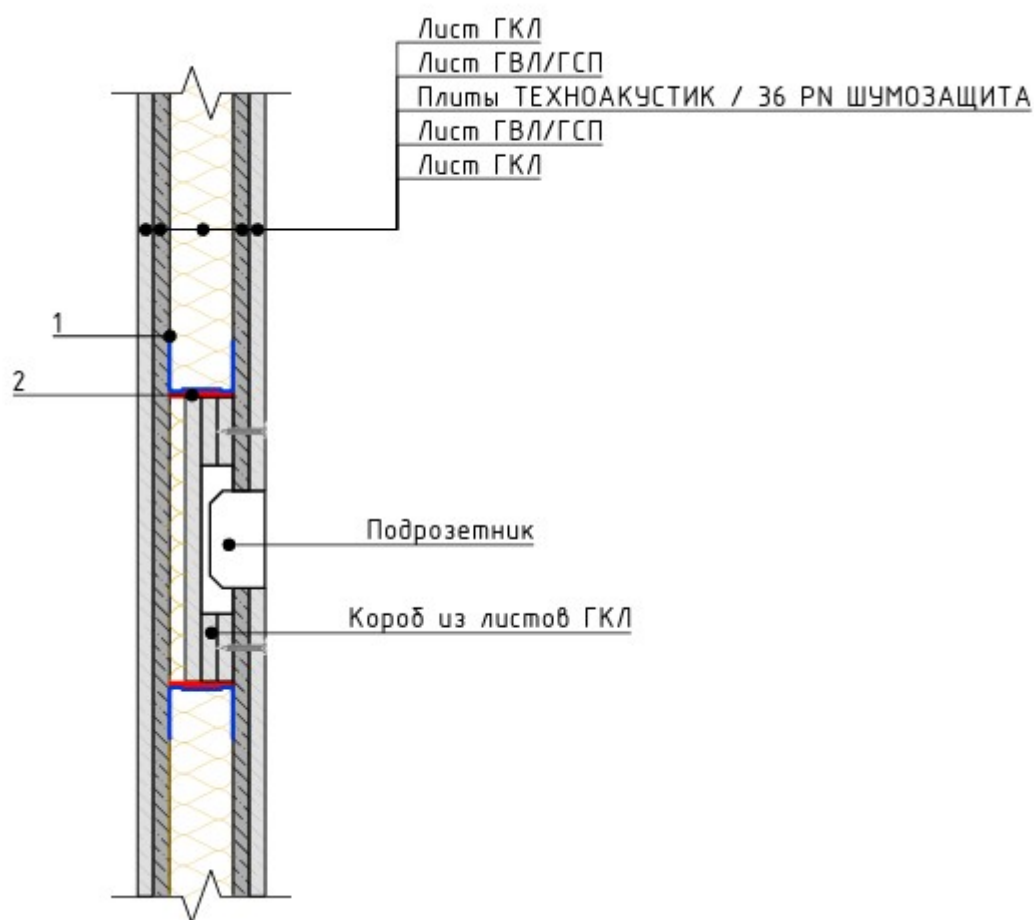
Рис. 3. Установка звукоизоляционных коробов для подрозетников в каркасную стену между комнатами. Взято из Альбома технических решений по устройству внутренних звукоизоляционных каркасных перегородок , узел У.2.15.
