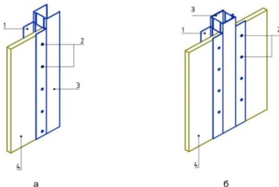
а – Схема установки закладных деталей длиной до 600 мм; б – схема установки закладных деталей длиной более 600 мм 1 – профиль направляющий ПН, 2 – саморез, 3 – профиль стоечный ПС, 4 – закладная из фанеры
