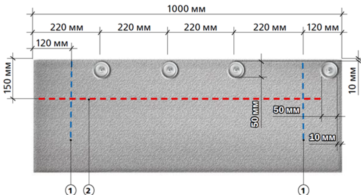
1 — Линия краевого нахлеста; 2 — Линия торцевого нахлеста
