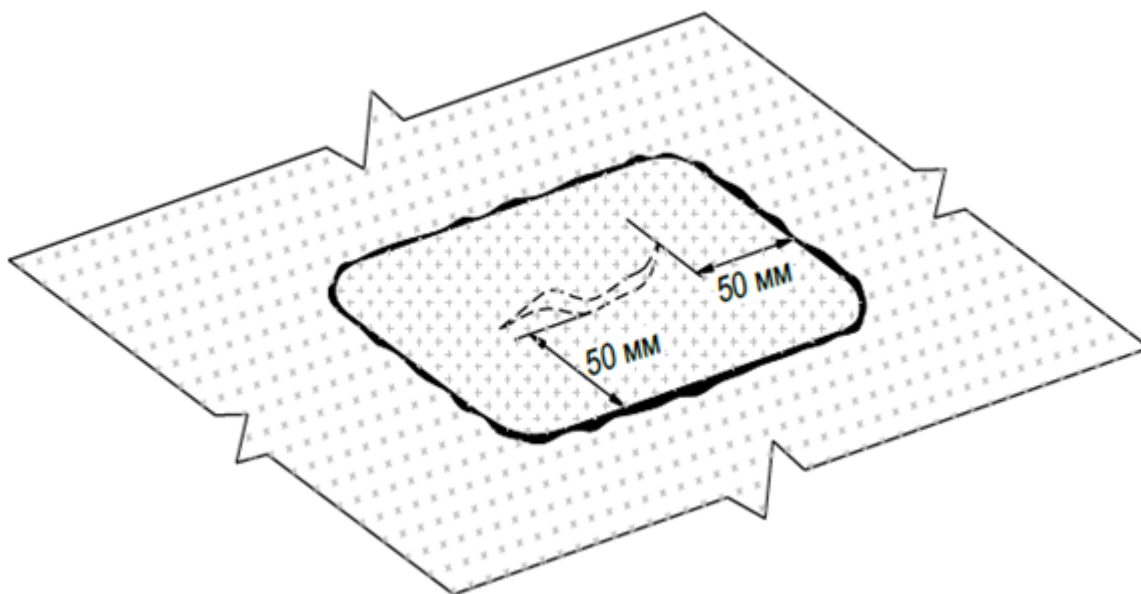
Рисунок 1. Требования к размеру заплатки для ремонта кровель из полимерных мембран ТЕХНОНИКОЛЬ
