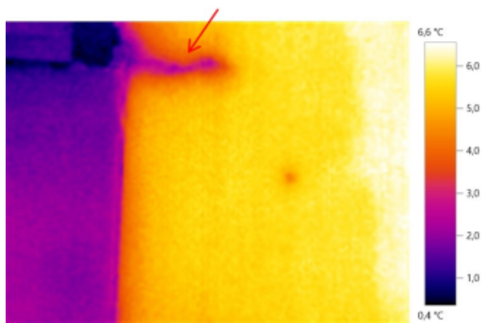
Пример №4. Вид на фасаде подобного дефекта.
