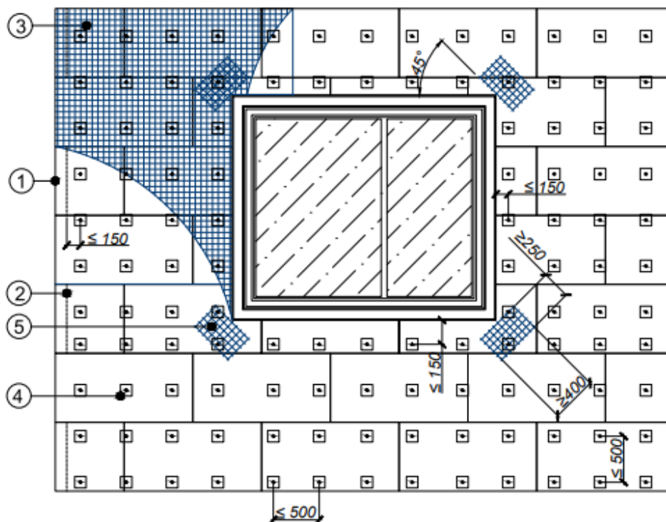
Рисунок 4 – Схемы усиления проемов
