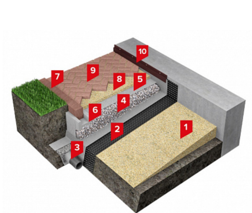
Рис. 3. Пример конструкции мягкой неутепленной отмостки, связанной с системой поверхностного водоотвода.
