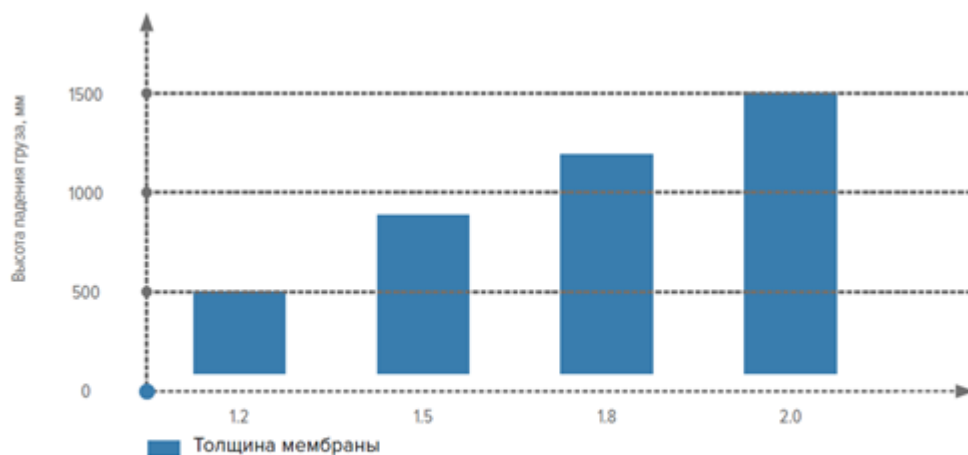
Зависимость показателя ударной прочности от толщины мембраны
