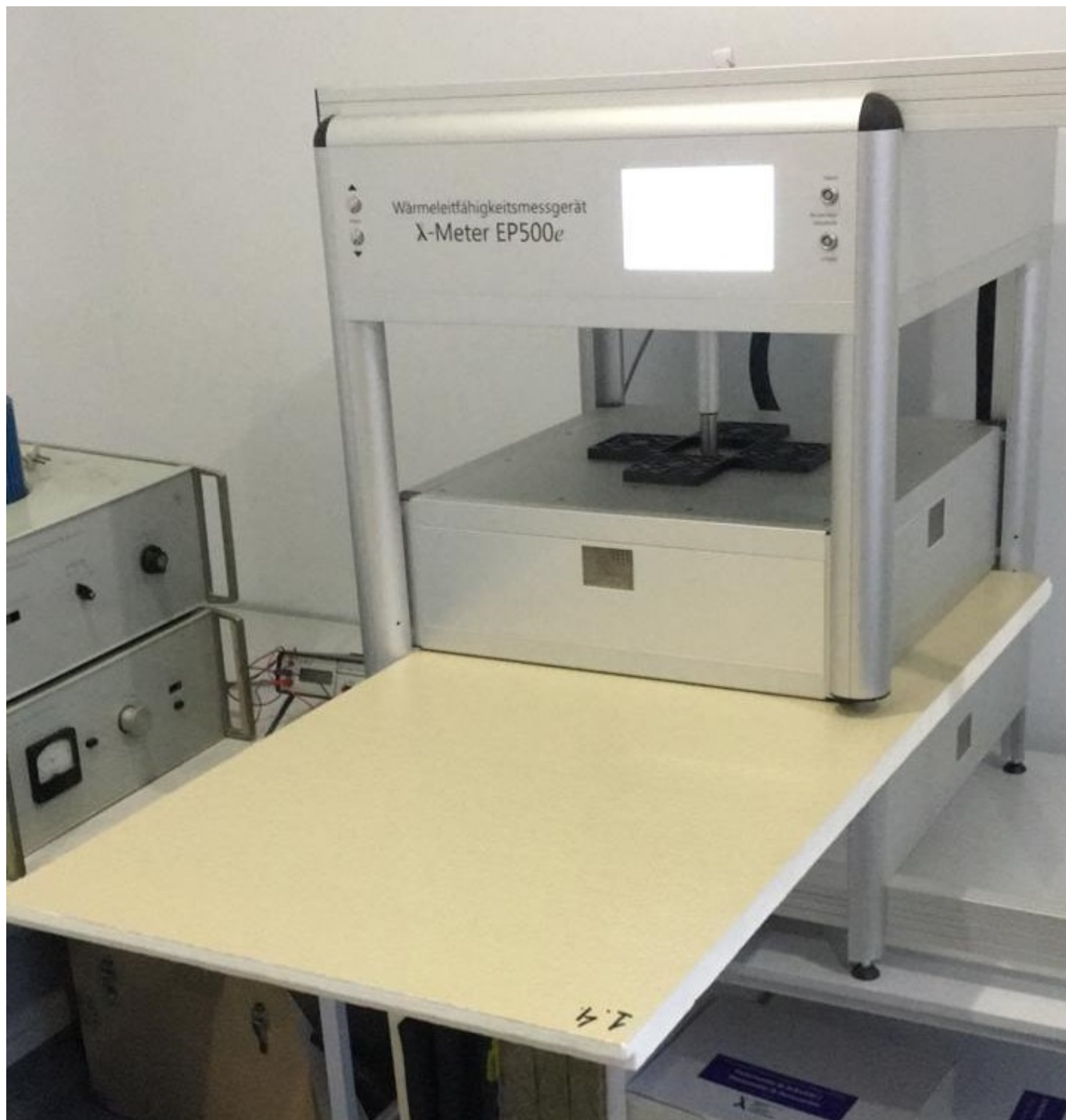
Рис. 1 Испытание цельной плиты LOGICPIR PROF Ф/Ф на приборе Lambda-Meter EP500e
