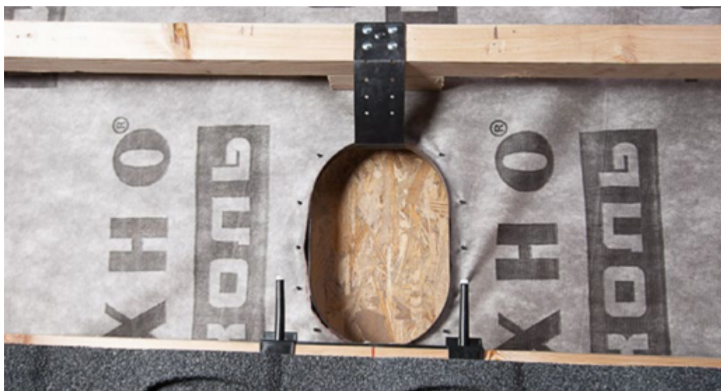
Проходной элемент (UNIVERSAL) для панели Roman
