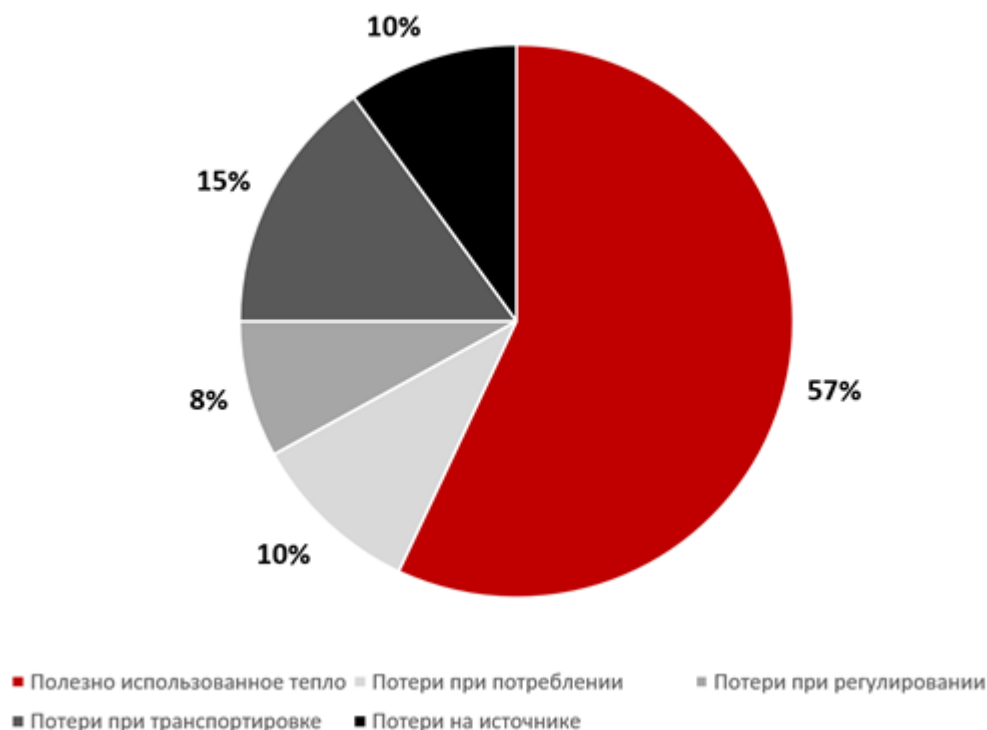
Потери тепла в централизованной системе отопления
