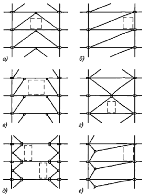
Рисунок 68 - Формы вертикальных связей многоэтажных и высотных зданий
