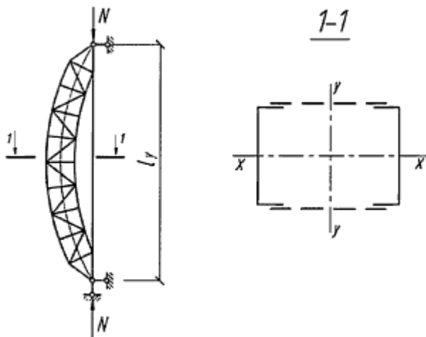
Рисунок 4 - Шарнирно опертый сквозной стержень
