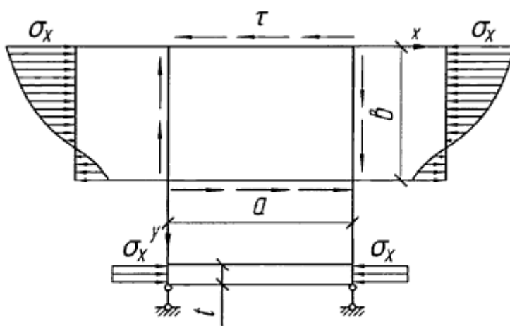
Рисунок 10 - Схема нагружения пластинки
