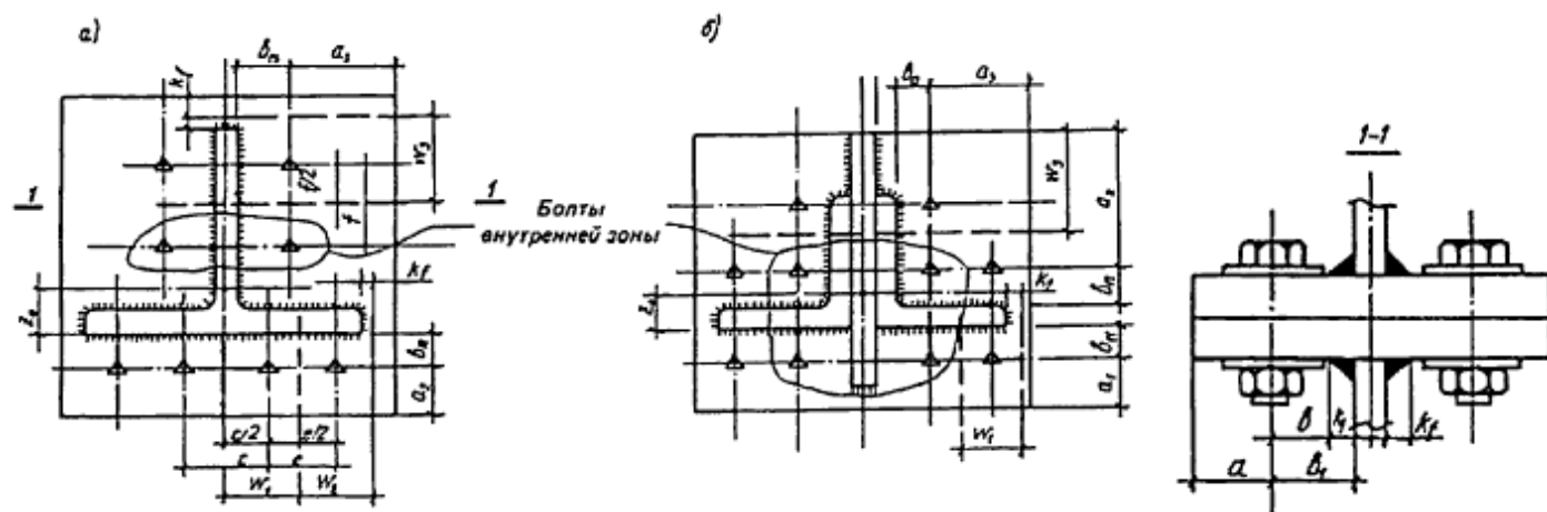
а) - из широкополочных тавров; б) - из парных равнополочных уголков
