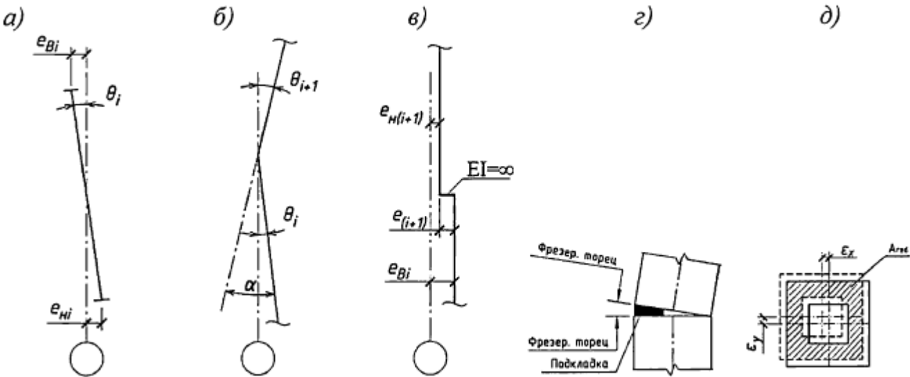
Рисунок 69 - Погрешности, возникающие при монтаже колонн многоэтажных зданий
