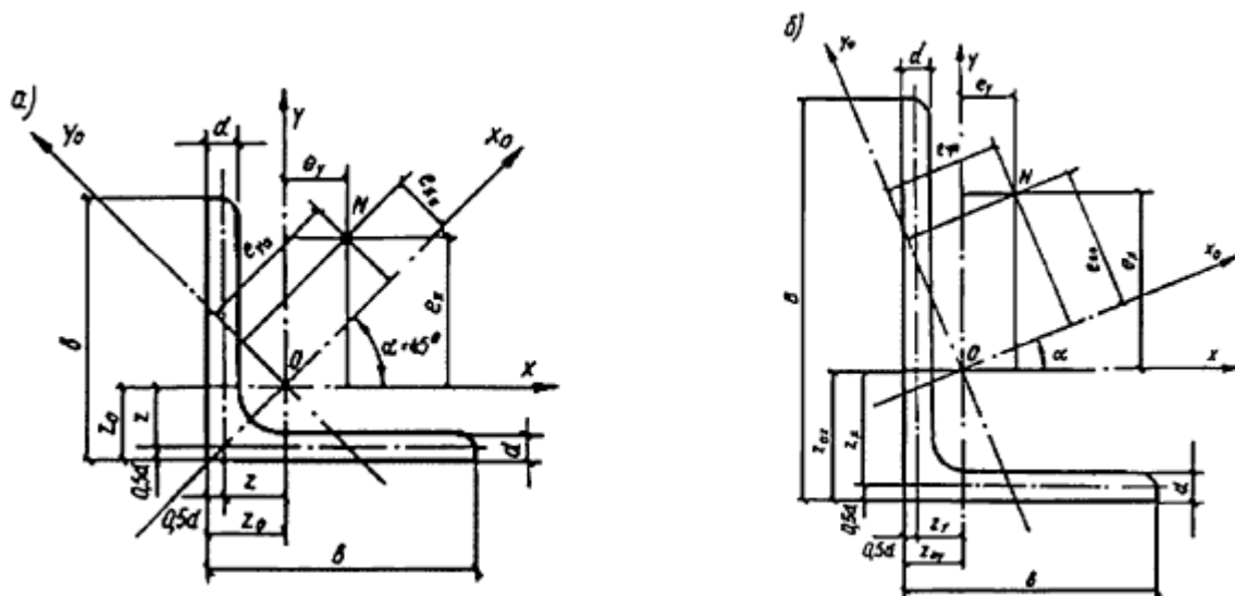
а) - равнополочного; б) - неравнополочного
