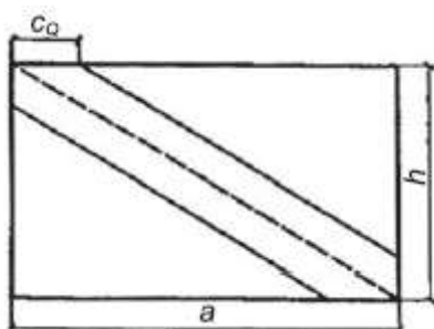
Рисунок 46 - Схема предельного состояния сечения балки при изгибе
