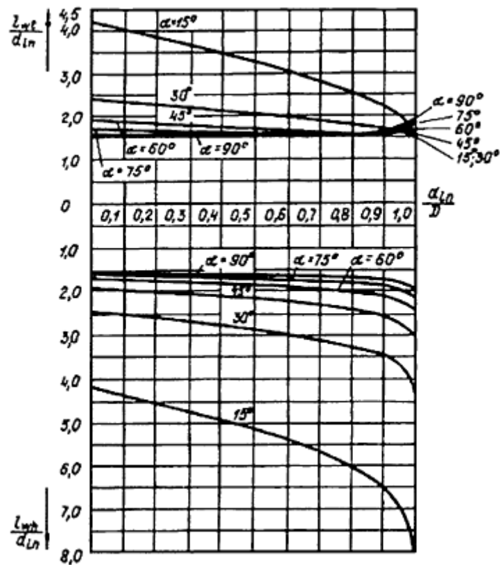
Рисунок 30 - Графики для определения полной длины "пяточного" l_{wn} и "носикового" l_{wf} участков сварного шва в соединении двух труб
