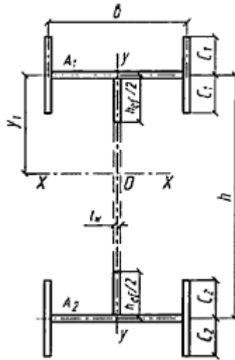
Рисунок 9 - Схема двутаврового обобщенного сечения с неустойчивой стенкой
