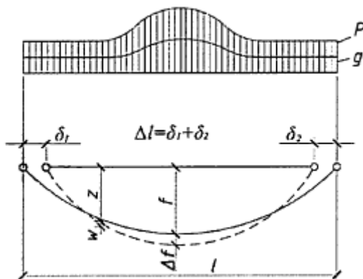
Рисунок 54 - К расчету нити на упругий провис
