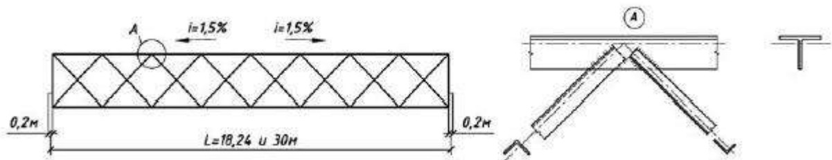
Рисунок 35 - Схема и узел фермы
