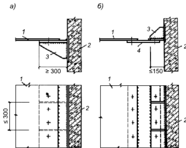
а) - внахлестку; б) - с использованием подкладного листа; 1 - мембрана; 2 - опорный контур; 3 - опорный столик; 4 - подкладка
