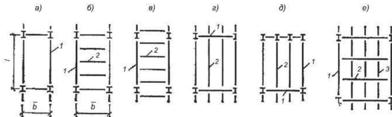
1 - главная балка, 2 - второстепенная балка (прогон), 3 - балка настила
