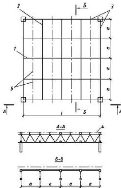
Рисунок 36 - Покрытие из перекрестных элементов
