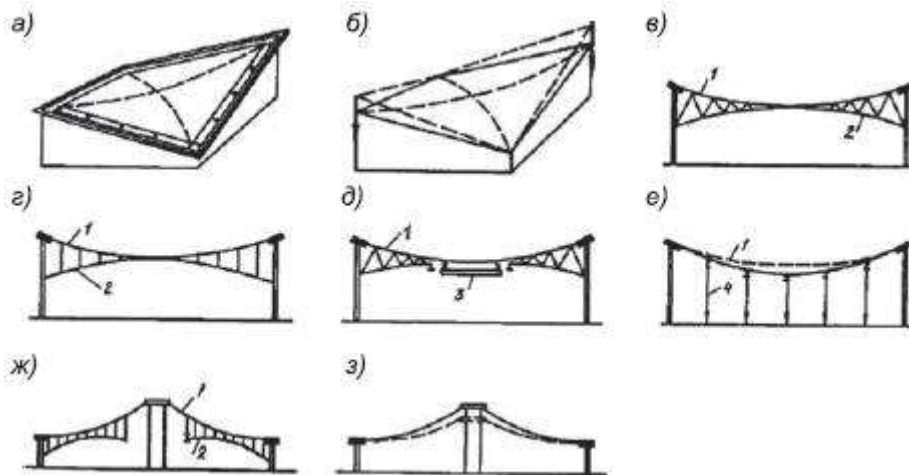
а) - притягиванием мембраны к контуру; б), в) - изменением геометрии покрытия; г), д), ж) - натяжением вантовых ферм; е) - притягиванием поперечных балок к основанию; 1 - мембрана; 2 - стабилизирующие ванты; 3 - центральный пригруз; 4 - оттяжки
