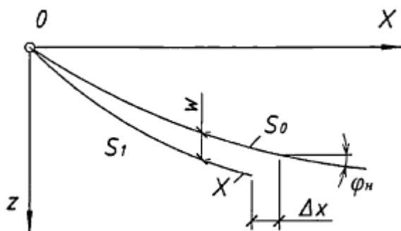
Рисунок 56 - К расчету нити на горизонтальные перемещения
