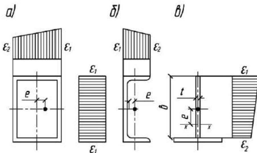
а) - трубчатое сечение; б) - швеллер; в) - тавр
