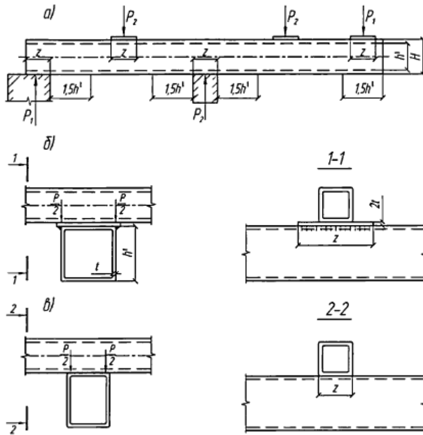
а) - схема нагрузок и реакций; б) - опирание через прокладку; в) - непосредственное опирание
