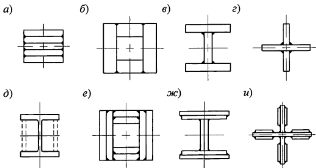
Рисунок 64 - Поперечные сечения колонн
