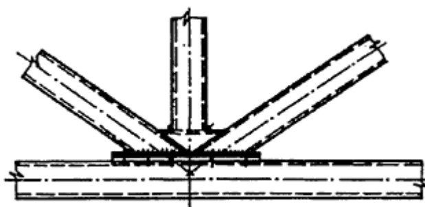
Рисунок 40 - Узел фермы с отсоединяющимся нижним поясом
