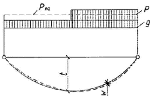
Рисунок 55 - К расчету нити на загрузку полупролета
