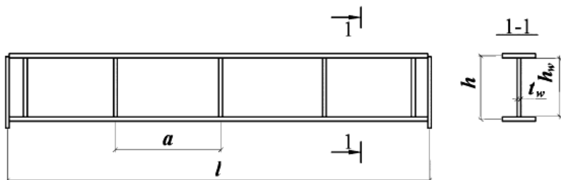
Рисунок 45 - Схема балки с гибкой стенкой
