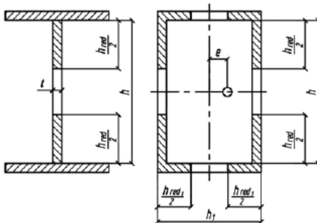
Рисунок 15 - Расчетные сечения стержней с гибкими стенками
