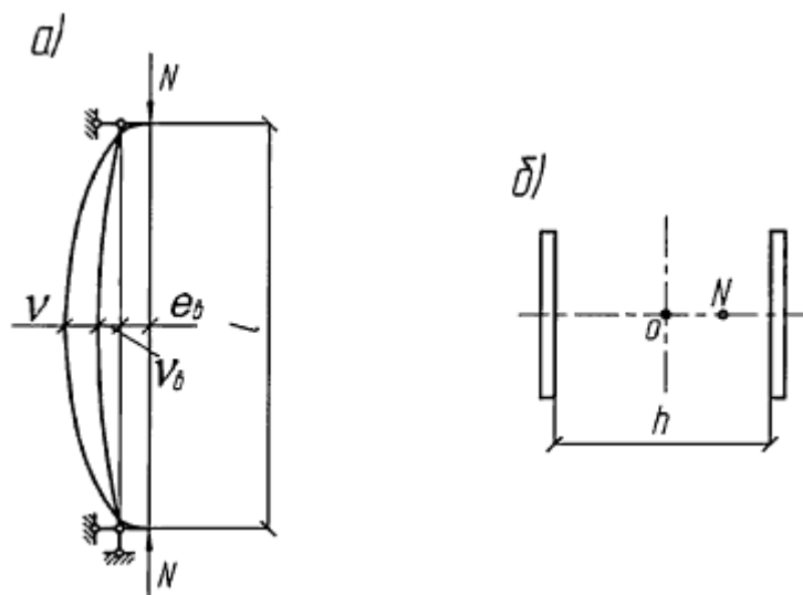
а) - изогнутая ось стержня; б) - идеализированное сечение
