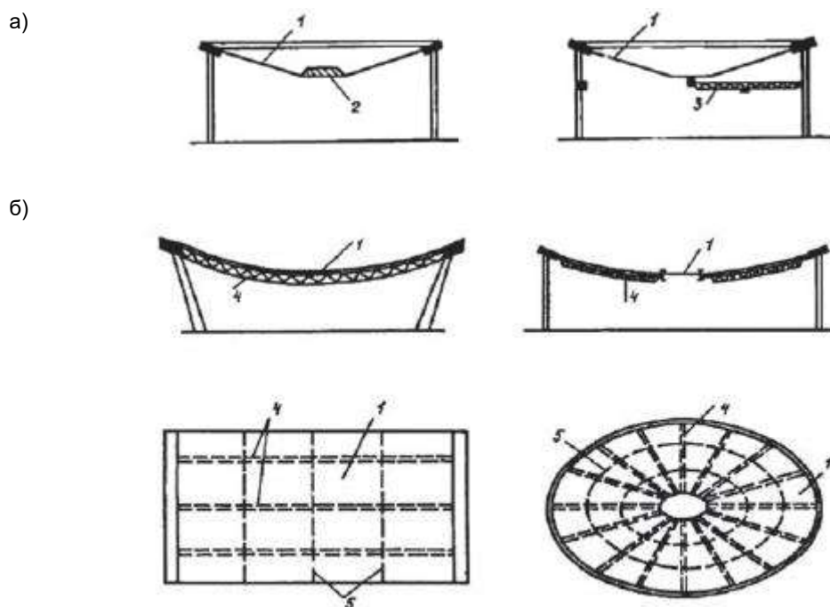
а) - пригрузом; б) - с использованием изгибно-жестких элементов; 1 - мембрана; 2 - пригруз; 3 - кольцевой кран; 4 - основные (продольные или радиальные) ребра; 5 - вспомогательные (поперечные или радиальные) ребра
