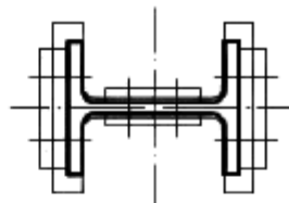
Вариант 2 – болтовой стык с накладками
