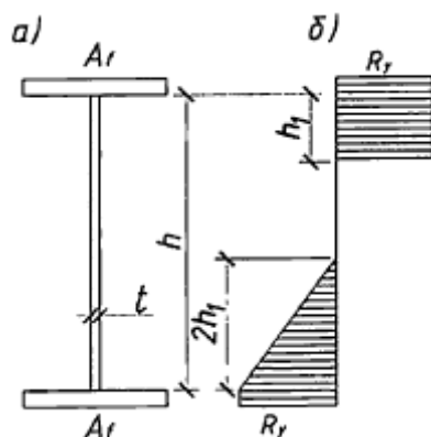
а) - сечение балки; б) - эпюра напряжений
