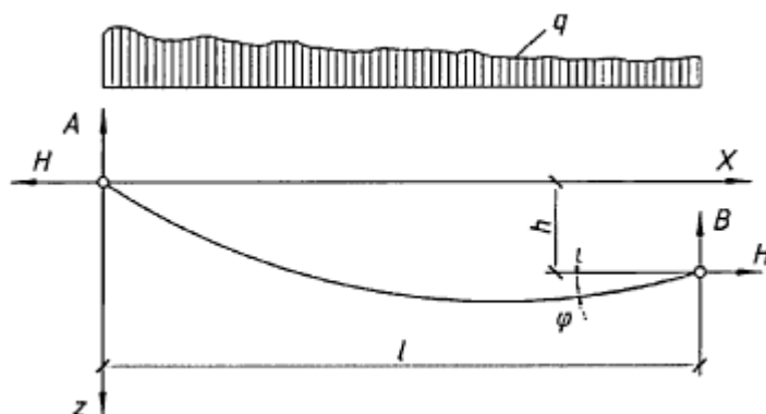
Рисунок 53 - К расчету нити на прочность Если опоры расположены на одном уровне, формула (194) приобретет вид
