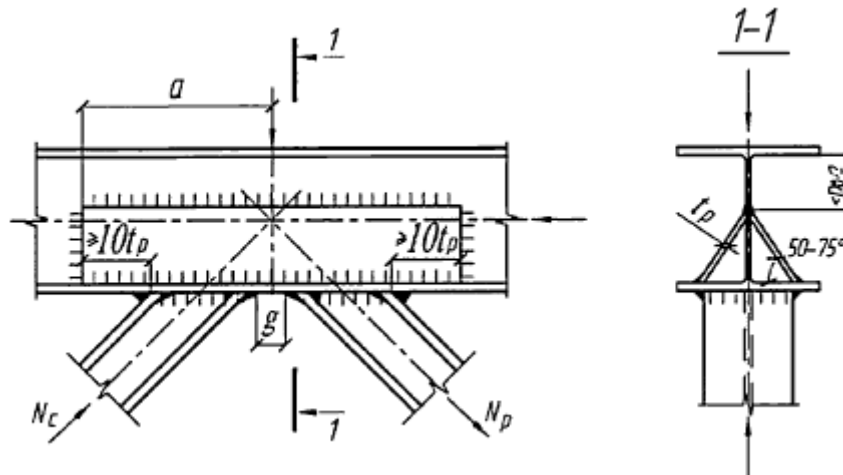
Рисунок 27 - Узел фермы, усиленный наклонными планками
