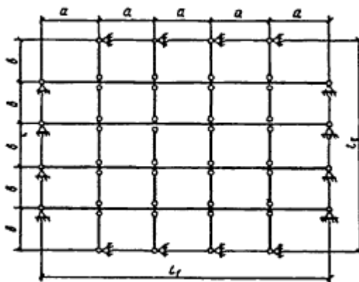
Рисунок 37 - Разбивка покрытия на главные и второстепенные балки
