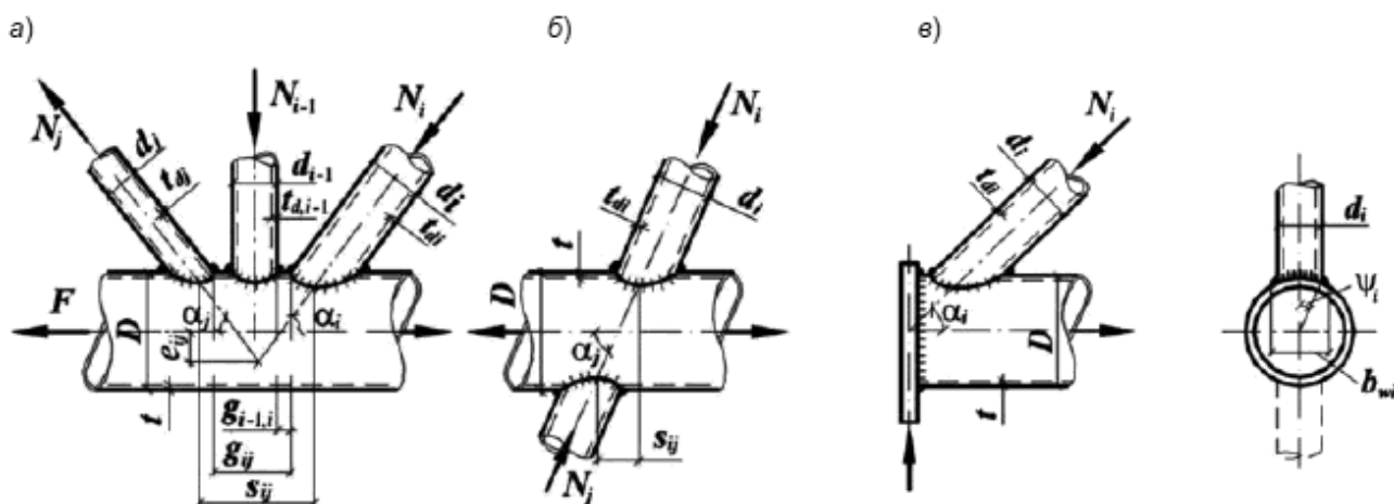
а) - К-образный; б) - Х-образный; в) - опорный
