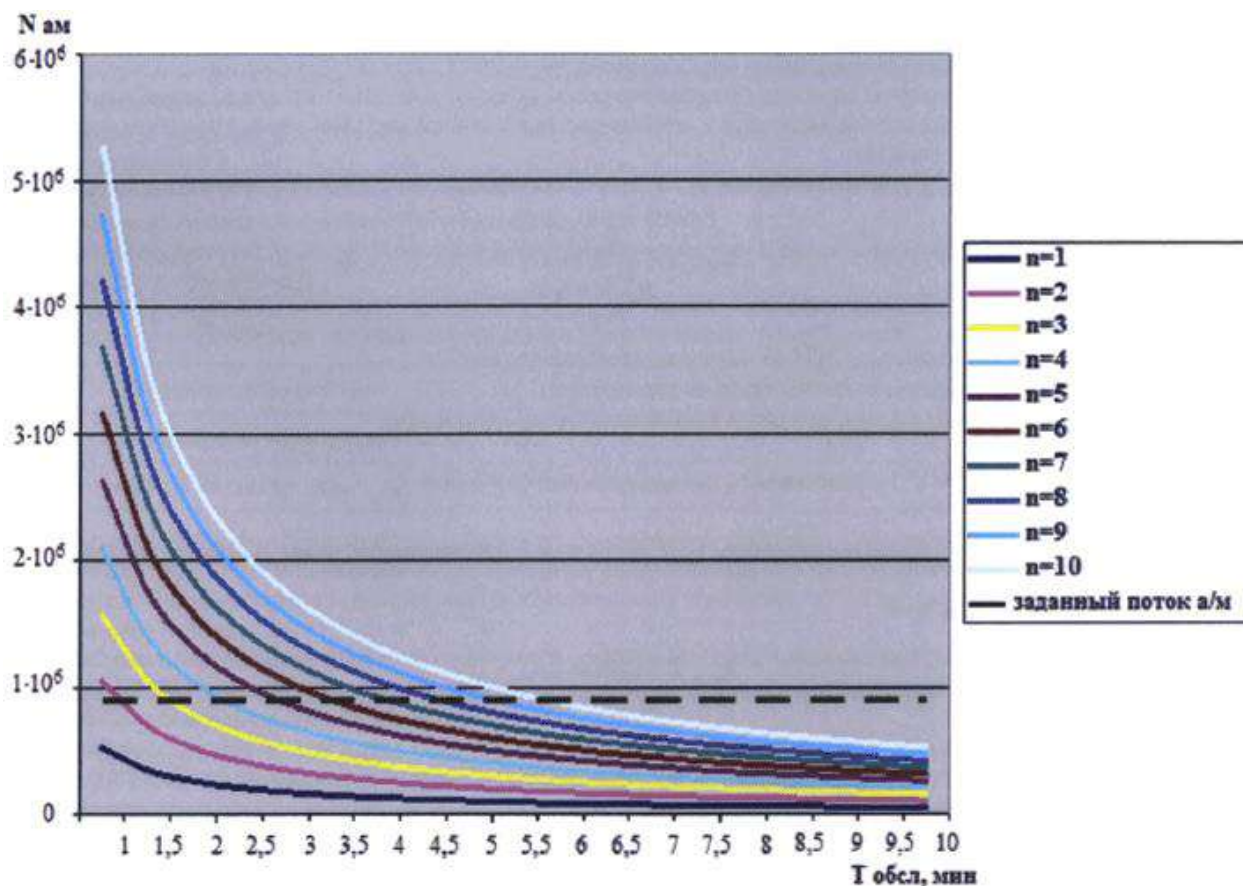
Рисунок Б.1 - Пропускная способность АВК
