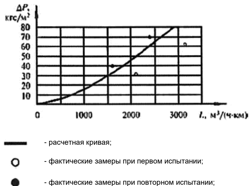
Рисунок В.3 - График характеристики герметичности отсека
