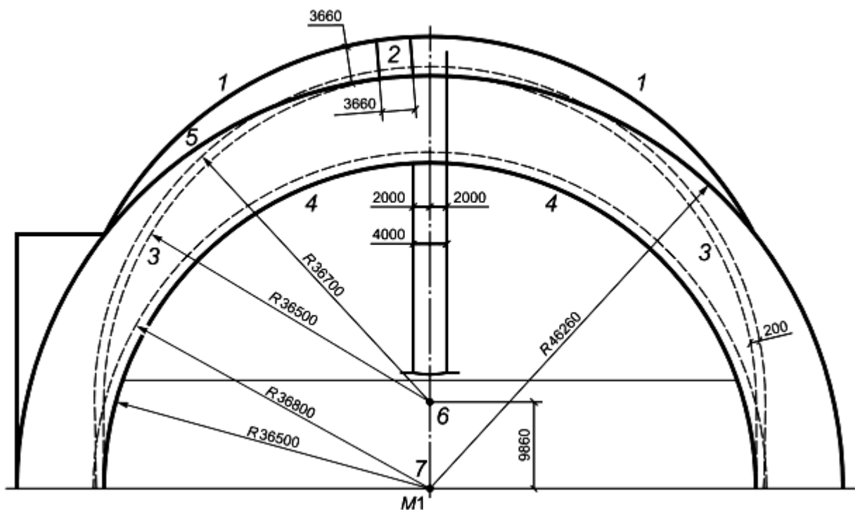
Расстояние линии бега от разметки внутреннего края дорожки - 0,20 м ( R=36,70 м). Длина линии бега на вираже при преодолении ямы с водой, расположенной вне виража дорожки, на 19,407 м больше, чем полукруглый вираж стандартной 400-метровой круговой дорожки (115,611 м). 1 - внешняя граница дорожки (вмонтированная заподлицо); 2 - яма с водой; 3 - разметка (поверхность дорожки); 4 - внутренняя граница дорожки (0,05 м высотой); 5 - внешняя граница дорожки
