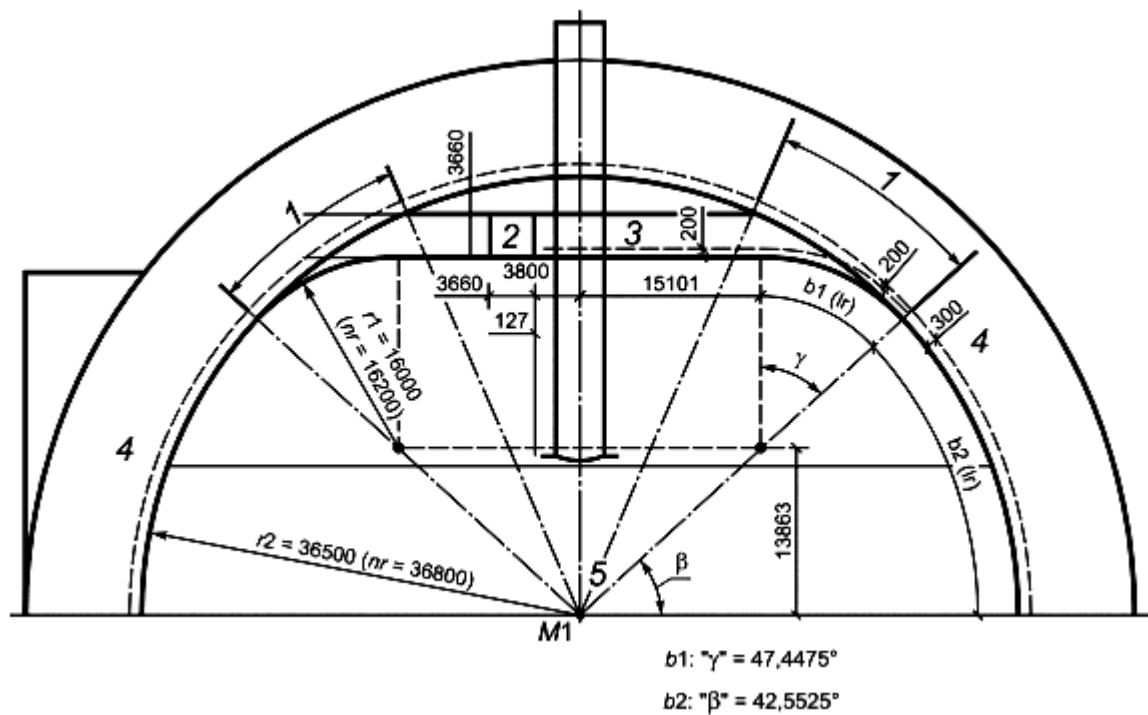
1 - переносная (нестационарная) бровка дорожки; 2 - яма с водой; 3 - прямая дорожка; 4 - расстояние между линией бега и внутренним краем дорожки; 5 - центр полуокружности Рисунок Е.6 - Яма с водой, расположенная внутри виража дорожки
