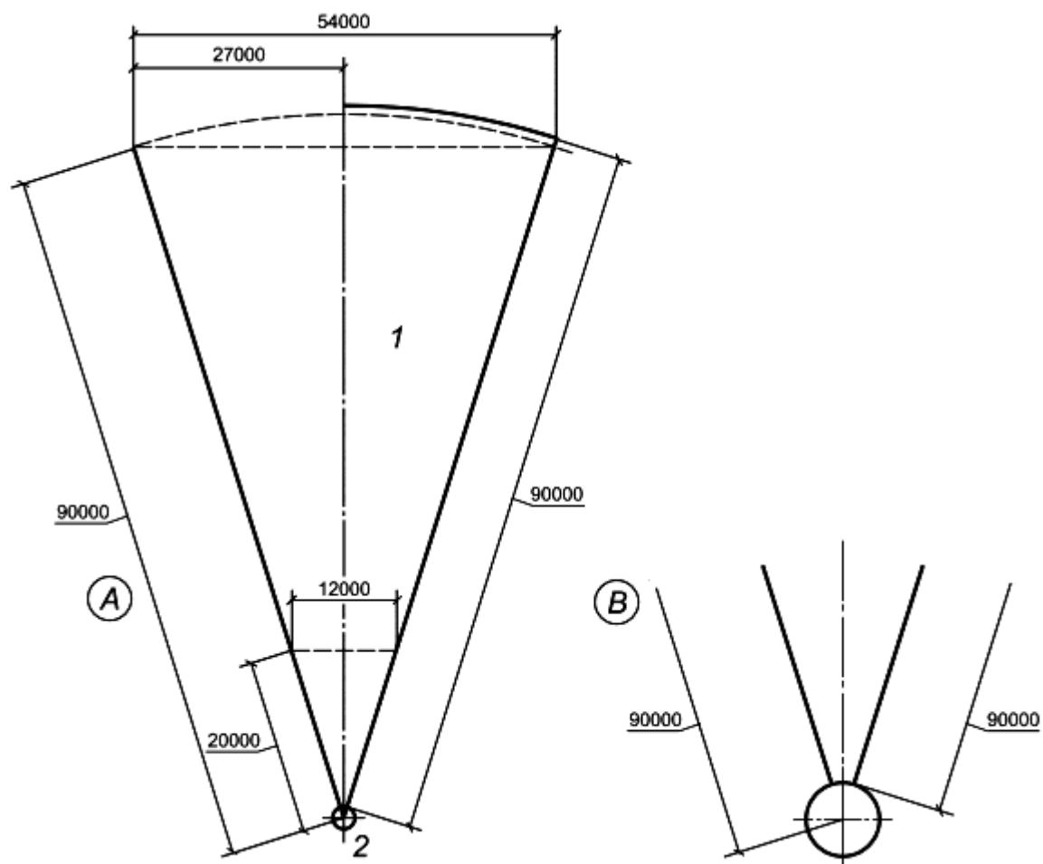
A - общая схема сектора; B - план разметки; 1 - сектор приземления; 2 - круг для метания Рисунок E.17 - Сектор для метания молота
