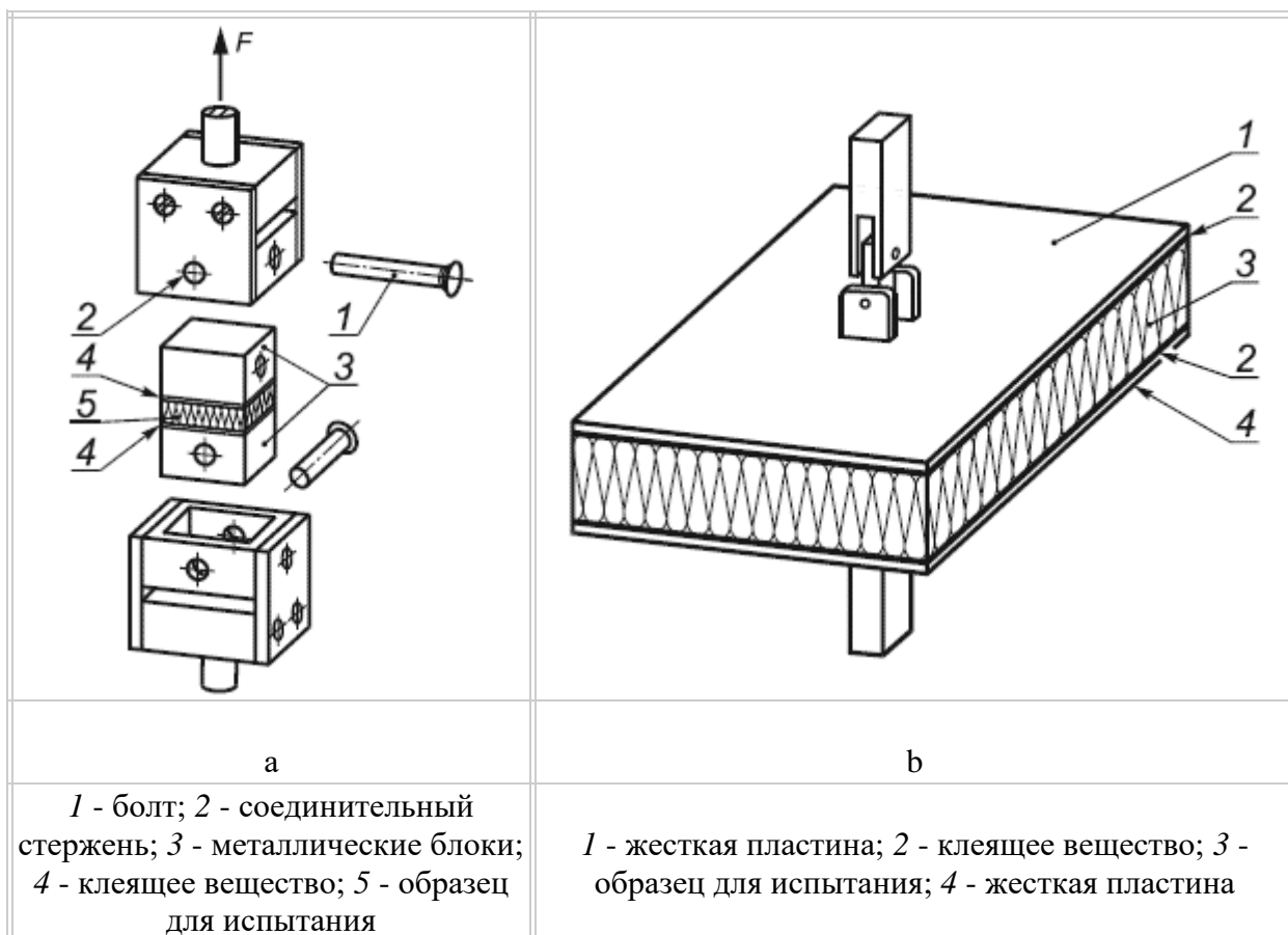
Рисунок 1 - Примеры приспособлений для крепления образца
