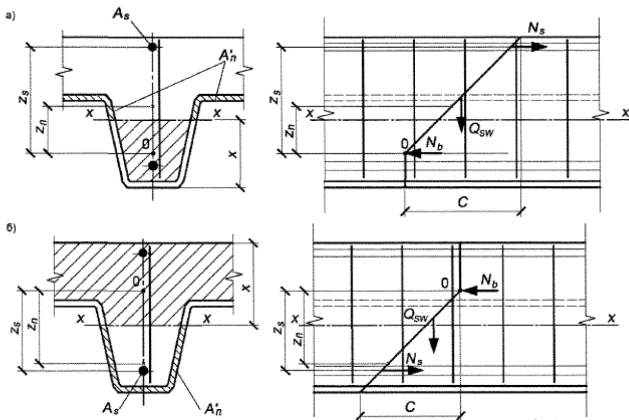
а) сжатая зона расположена внутри гофра; б) сжатая зона расположена над гофром Рисунок 6.8а - Схема усилий в наклонном сечении при расчете его прочности на действие моментов
