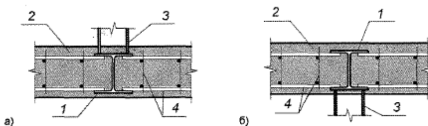
Рисунок Е.3 - Схема узла сопряжения монолитного перекрытия по профилированному настилу с поясами ферм
