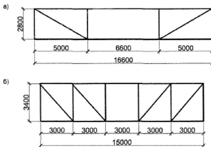
Рисунок Е.2 - Примеры габаритных размеров схем ферм для зданий различного функционального назначения
