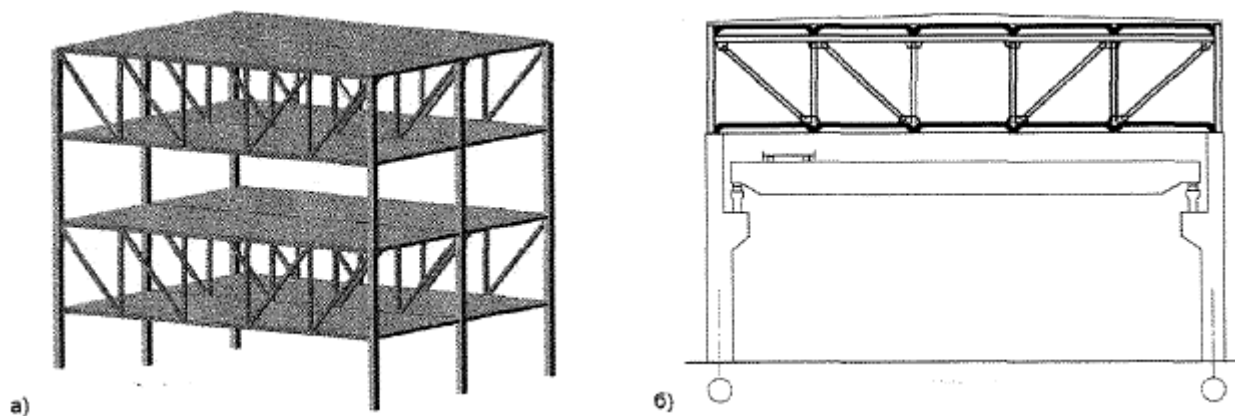
Рисунок Е.1 - Пространственно-армированные сталежелезобетонные блок-секции
