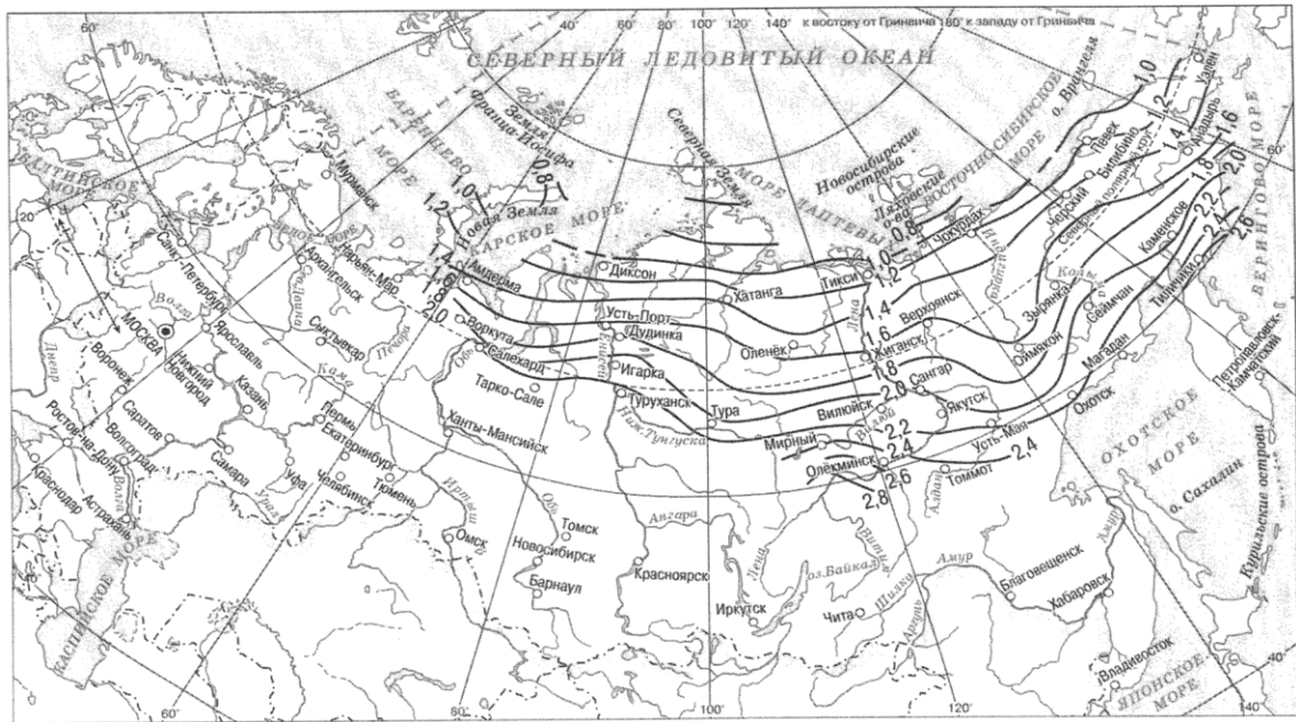
Рисунок Г.2 - Глубины оттаивания глинистых грунтов
