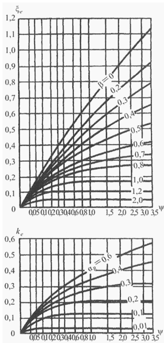
Рисунок К.2 - Графики для определения коэффициентов \xi_e и k_e
