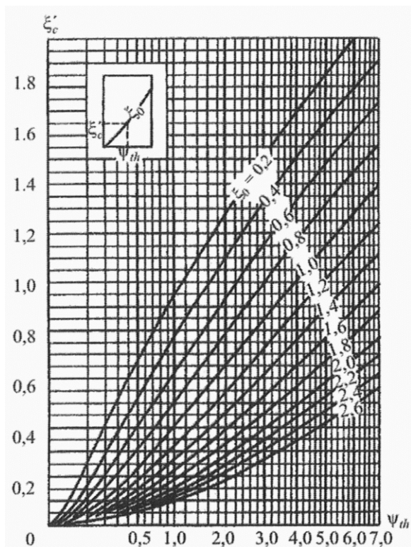
Рисунок К.5 - Графики для определения коэффициента \xi'_c
