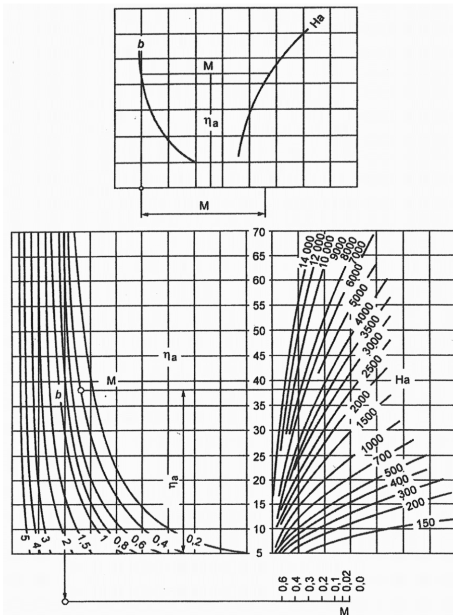
Рисунок Р.1 - Номограмма для расчета радиуса охлаждения
