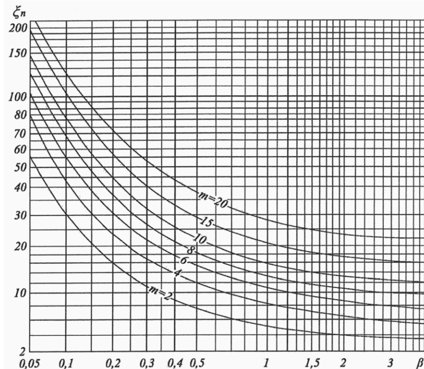
Рисунок Н.3 - Номограмма для определения оттаивания многолетнемерзлых грунтов вокруг холодного трубопровода
