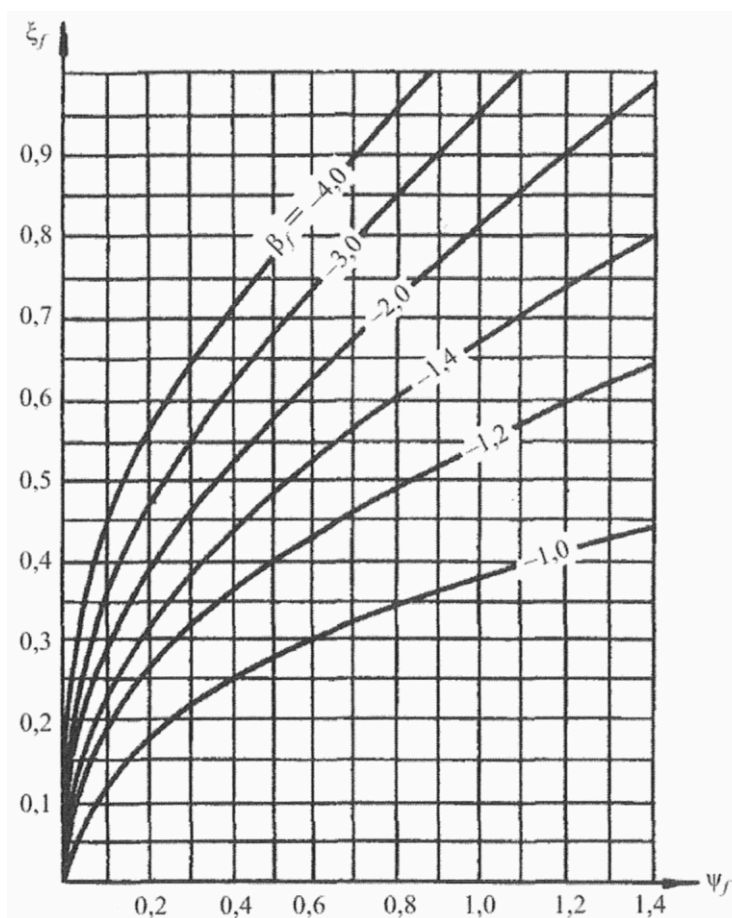
Рисунок Е.1 - Графики для определения коэффициента \beta_f
