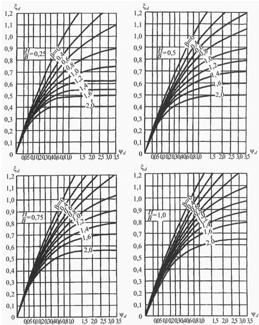
Рисунок К.4 - Графики для определения коэффициента \xi_d
