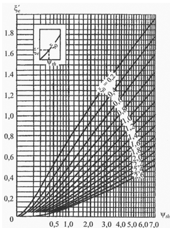
Рисунок К.6 - Графики для определения коэффициента \xi'_c
