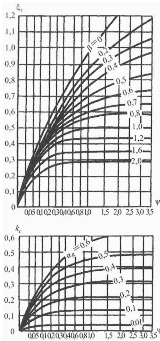
Рисунок К.1 - Графики для определения коэффициентов \xi_c и k_c
