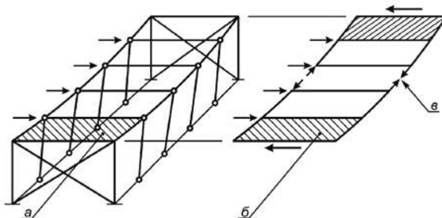
а - настил; б - зона сдвига в настиле; в - усилия в поясах краевых элементов
