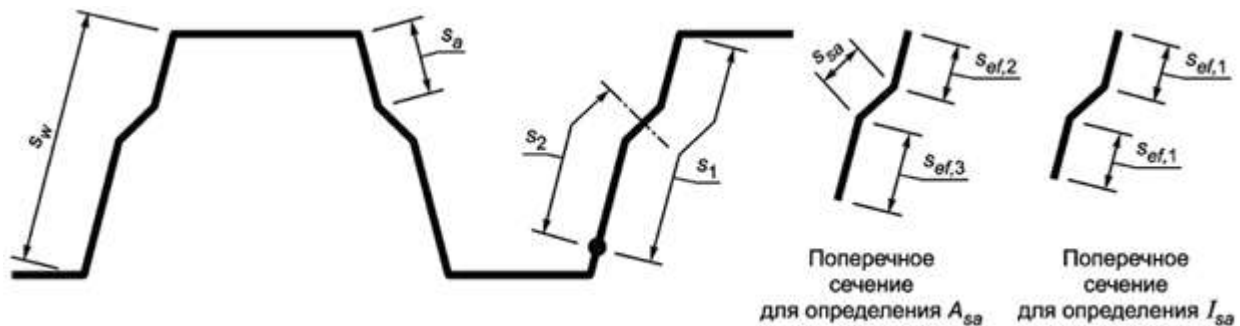
Рисунок 7.12 - Элементы жесткости стенок трапецевидных гофрированных листов
