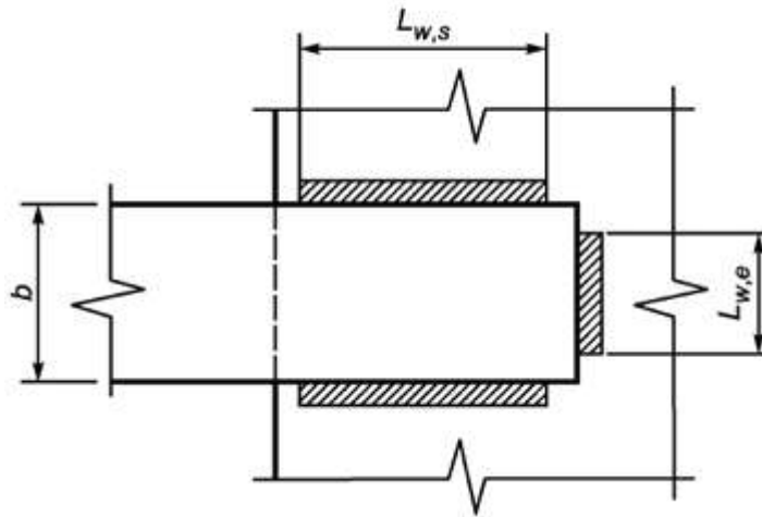
Рисунок 11.3 - Соединение с угловыми швами
