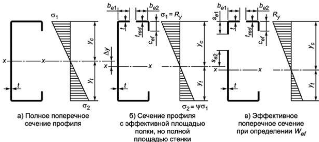
Рисунок 8.6 - Эффективное поперечное сечение (при \sigma_{com} = R_y ) для определения предельного изгибающего момента
