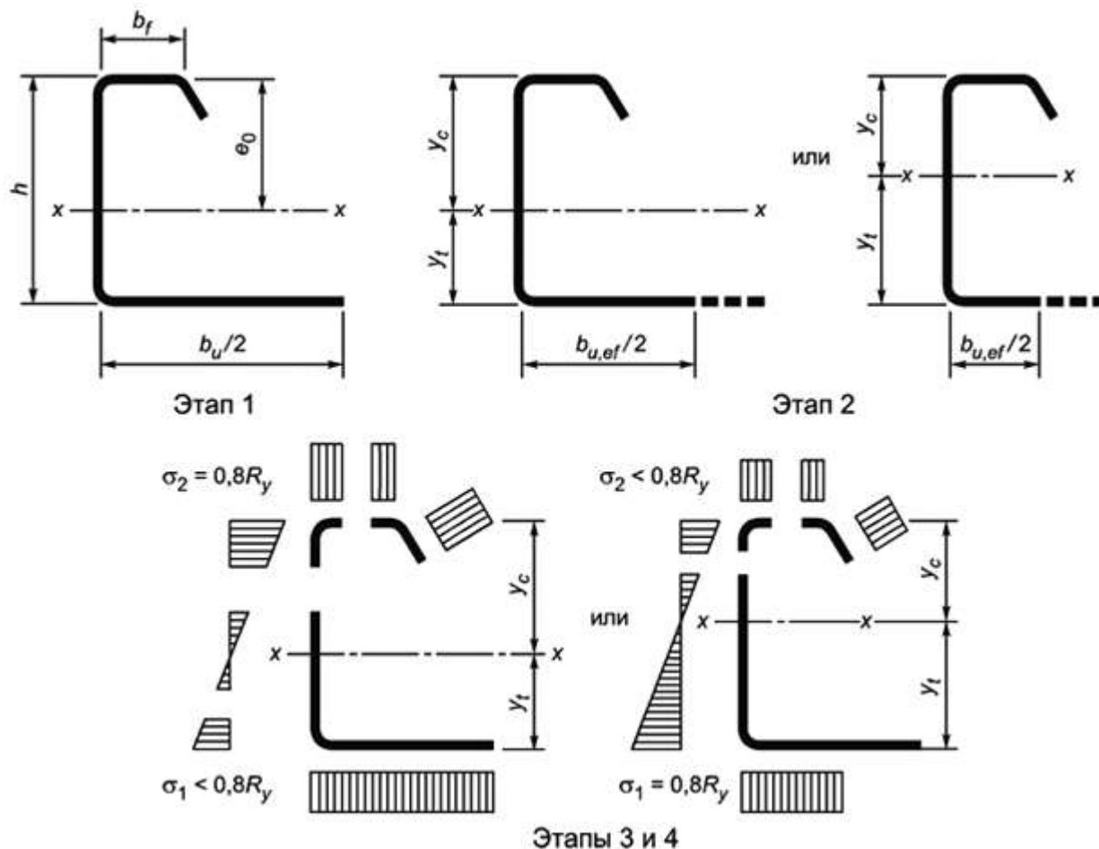
Рисунок 9.3 - Определение предельного момента при растянутой широкой полке
