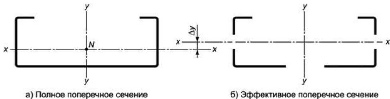
Рисунок 8.1 - Эффективное поперечное сечение при сжатии
