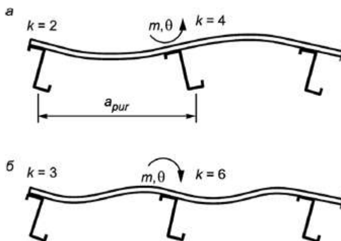
Рисунок Б.3 - К определению C_{D,C}
