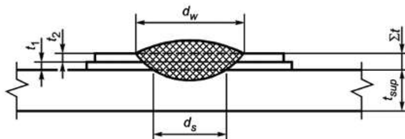
б) Присоединение двух листов ( \sum t = t_1 + t_2 )
