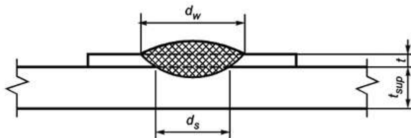
а) Присоединение одного листа ( \sum t = t )
