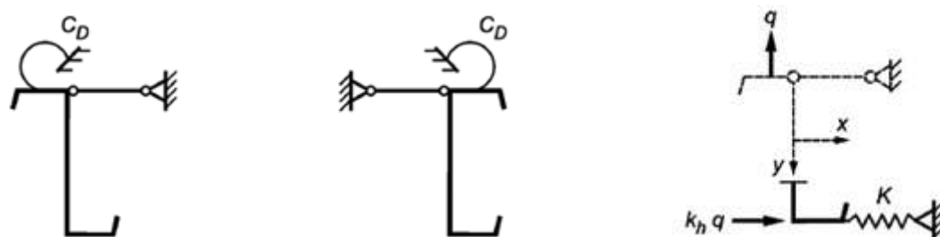
а) Модель прогона с раскреплением верхней полки угловой связью с жесткостью C_D , обеспечиваемой настилом б) Замена угловой связи с жесткостью C_D линейной связью с жесткостью K
