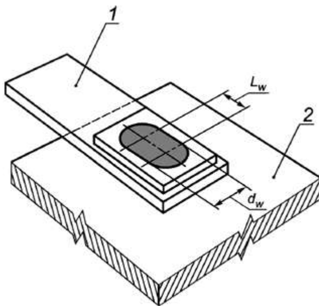
1 - присоединяемый элемент или лист; 2 - несущий элемент
