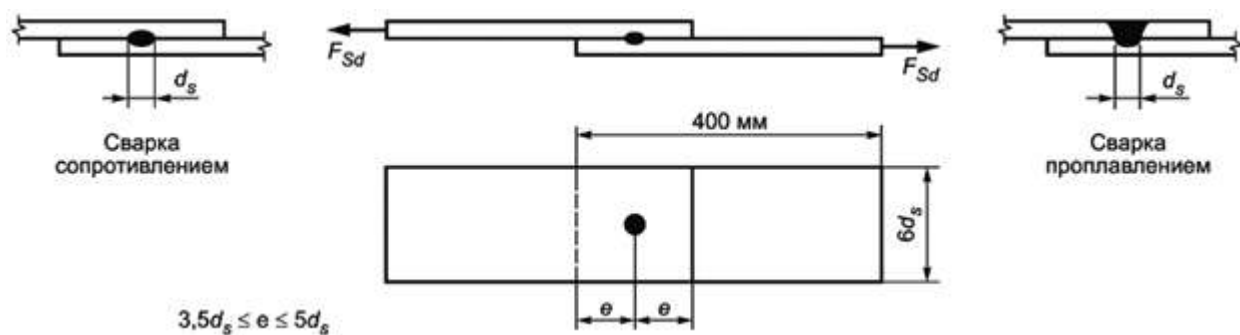
Рисунок 11.2 - Образцы для испытаний на срез сварных точек
