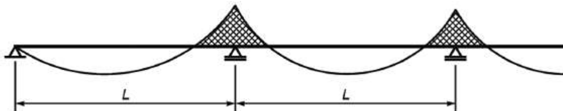
Рисунок Б.5 - Изменение сжимающих напряжений в свободной полке при действии прижимной (направленной вниз) нагрузки
