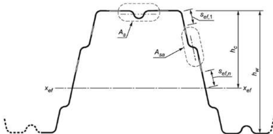
Рисунок 7.13 - Трапецевидный гофрированный лист с промежуточными элементами жесткости на полках и стенках
