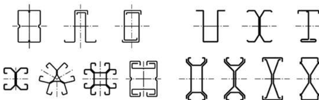
Рисунок 5.2 - Открытые и замкнутые составные сечения элементов конструкций из стальных тонкостенных холодногнутых оцинкованных профилей
