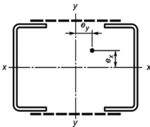
Рисунок 8.8 - Сечение сквозного стержня, подверженного сжатию и изгибу в обеих главных плоскостях
