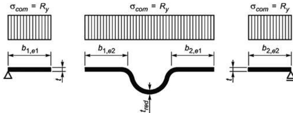
Рисунок В.11 - Четвертый этап. Окончательное эффективное поперечное сечение сжатой
