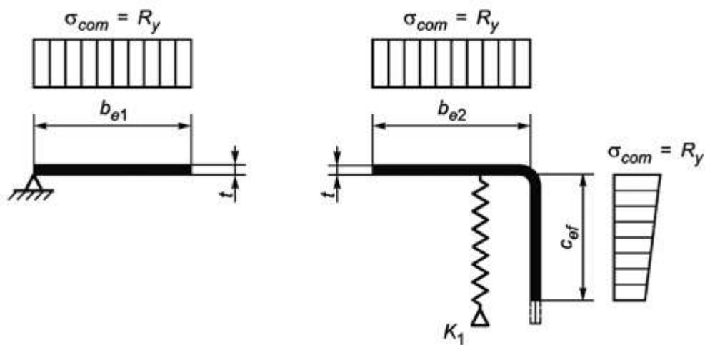
Рисунок В.2 - Первый этап. Начальное эффективное поперечное сечение сжатой полки с элементом жесткости при K = \infty и нормальных напряжениях \sigma_{com} = R_y
