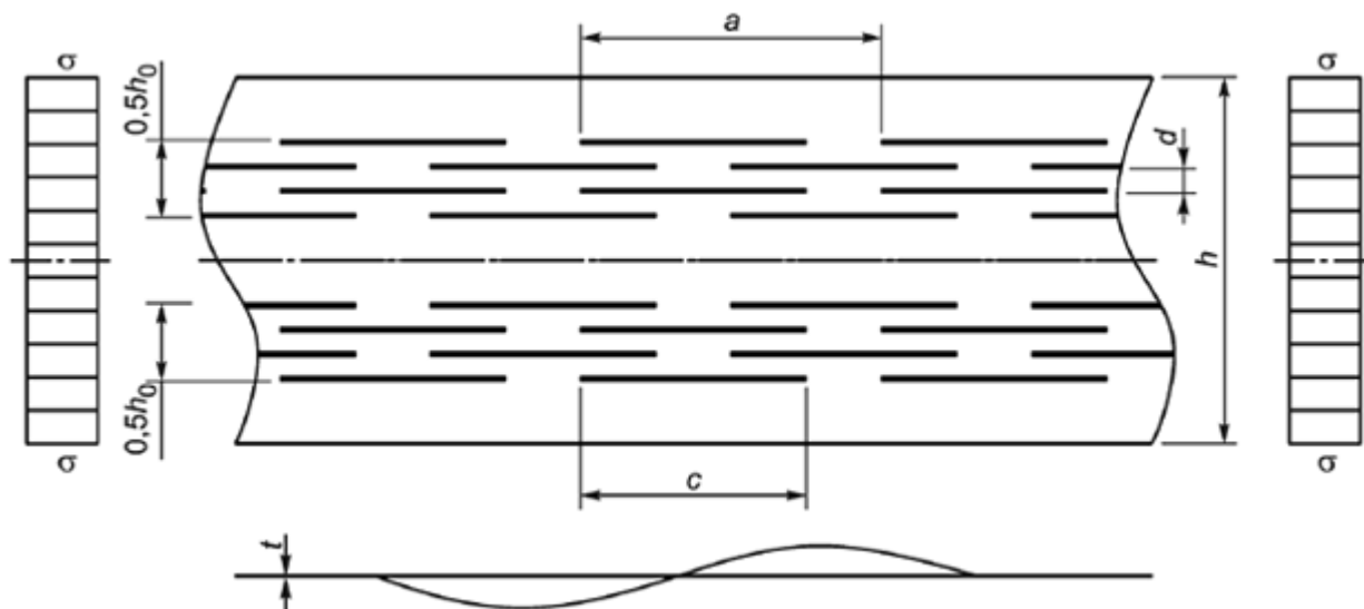
б) Пластина с двумя одинаковыми рядами перфорации
