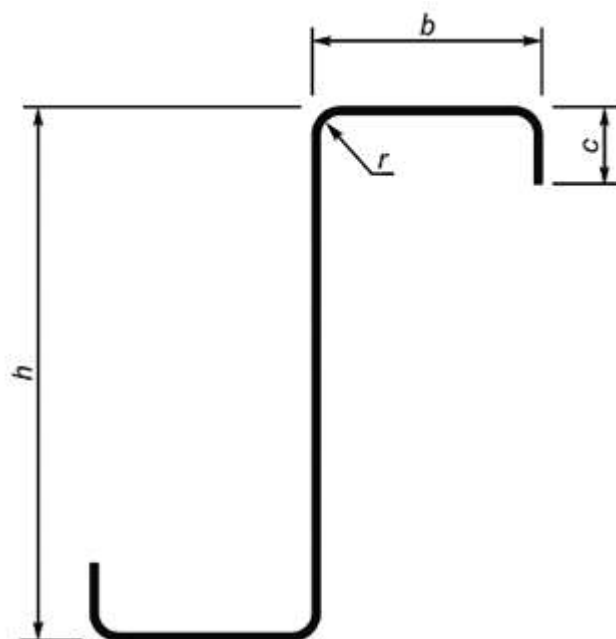
Рисунок 7.1 - Пример обозначения размеров S-образного сечения
