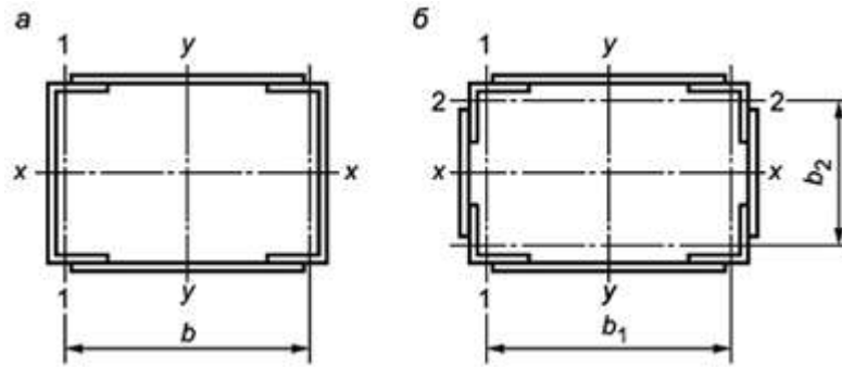
а - стержень с двумя ветвями; б - стержень с четырьмя ветвями
