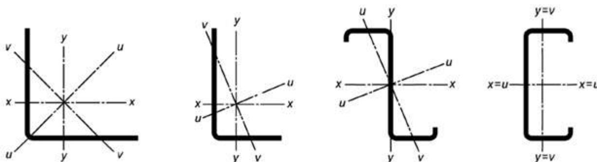
Рисунок 7.2 - Обозначения осей
