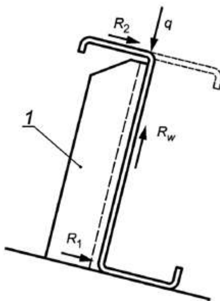
1 - опорный элемент
