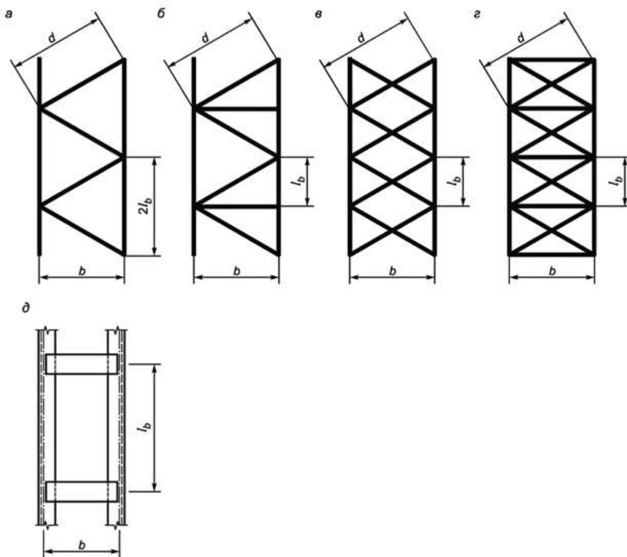
а - треугольная решетка; б - треугольная решетка с распорками; в - крестовая решетка; г - крестовая решетка с распорками; д - сквозной стержень с планками
