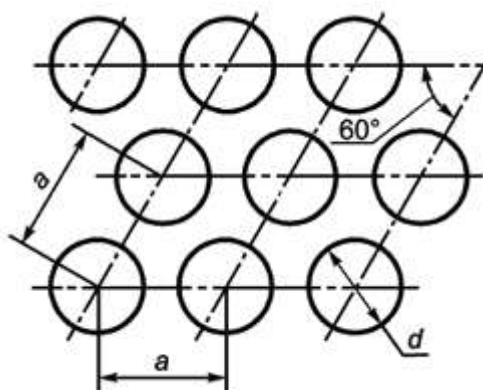
Рисунок 7.14 - Схема расположения отверстий в перфорированной пластине
