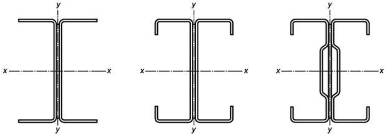
Рисунок 8.7 - Сечения сплошных стержневых колонн и стоек
