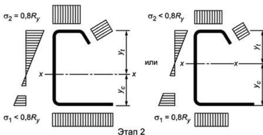
Рисунок 9.2, лист 2
