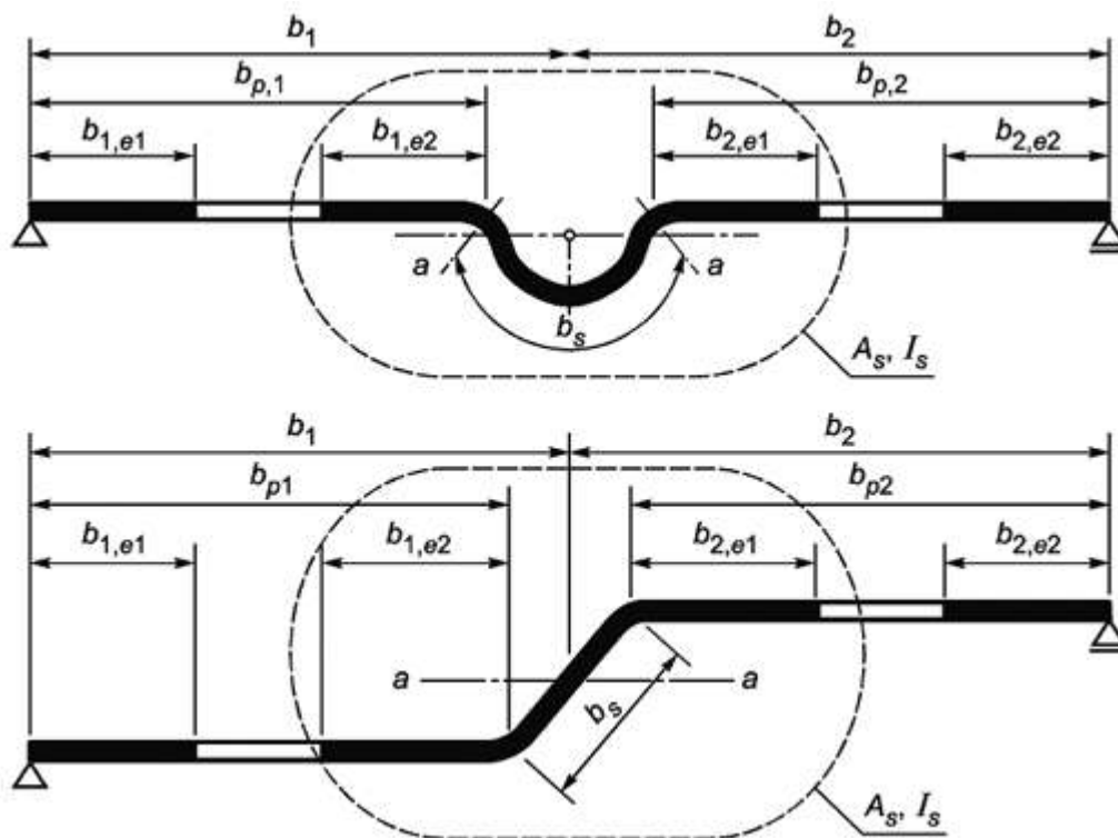
Рисунок 7.9 - Промежуточные элементы жесткости
