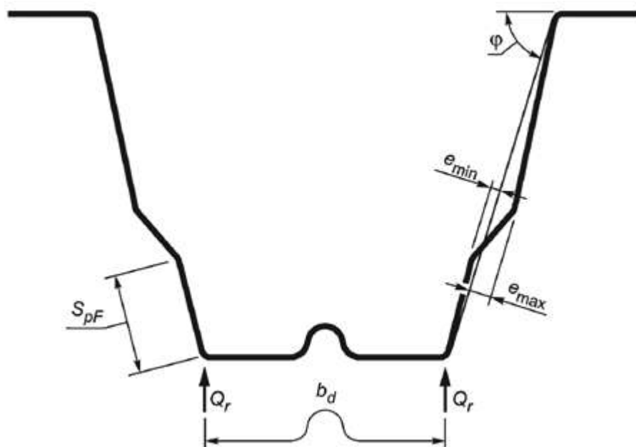
Рисунок 8.12 - Стенка с продольными элементами жесткости
