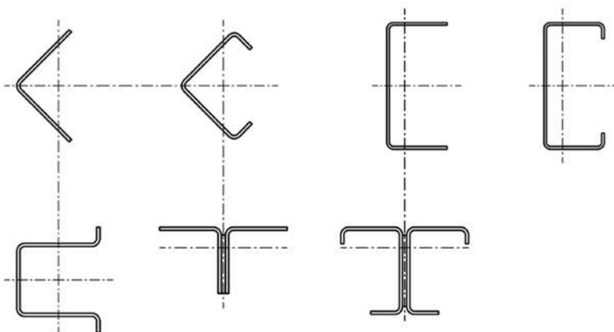
Рисунок 8.2 - Поперечные сечения, предрасположенные к изгибно-крутильной форме потери устойчивости
