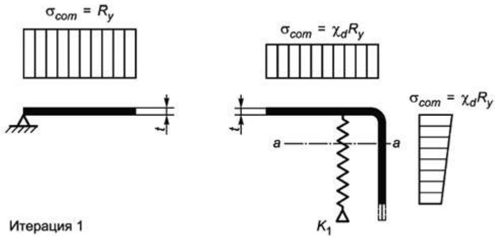
Рисунок В.4 - Второй этап. Сниженная прочность \chi_d R_y для начального расчетного сечения элемента жесткости с площадью A_s
