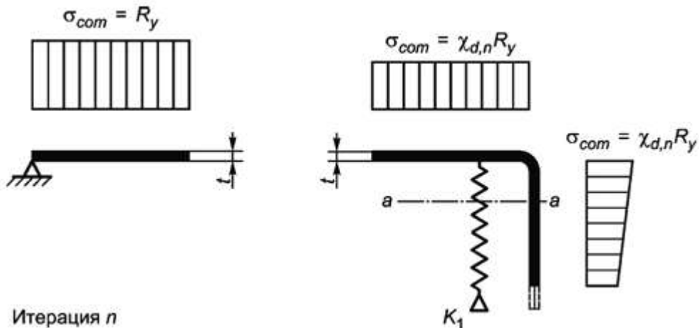
Рисунок В.5 - Третий этап. Сниженная прочность \chi_{d,n} R_y для уточненного расчетного сечения элемента жесткости с площадью A_{s,n} в итерации n
