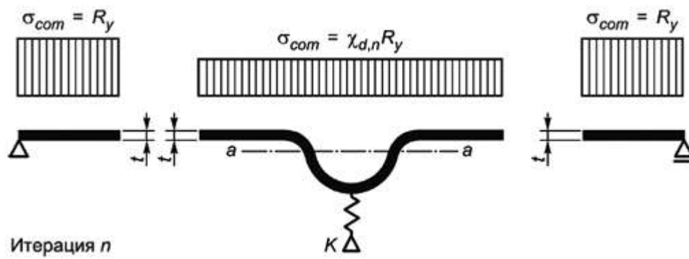
Рисунок В.10 - Третий этап. Сниженная прочность \chi_{d,n} R_y для уточненного расчетного сечения элемента жесткости с площадью A_{s,n} в итерации n
