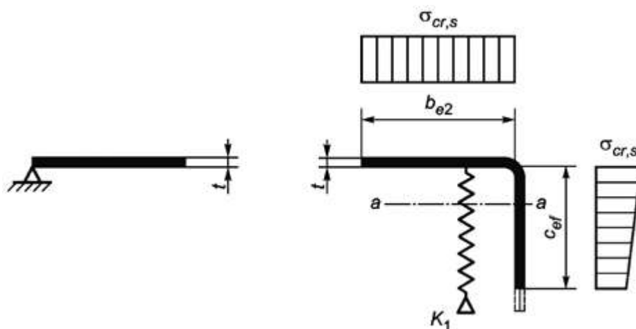
Рисунок В.3 - Второй этап. Критические напряжения потери устойчивости \sigma_{cr,s} краевого элемента жесткости, полученного на первом этапе
