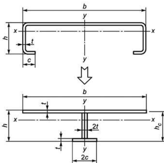
Рисунок Д.1 - Условное представление сечения с одной осью симметрии в виде двутавра для определения параметра y_j
