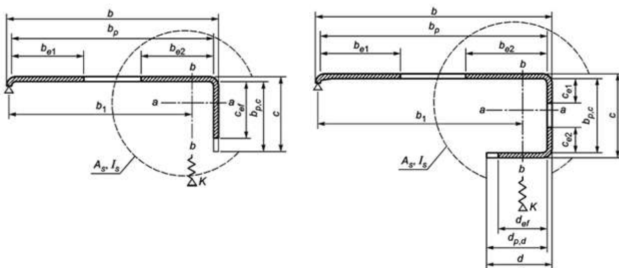
Рисунок 7.7, лист 2
