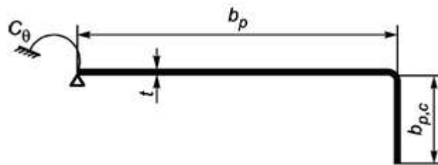
Рисунок В.1 - Сечение сжатой полки с краевыми условиями
