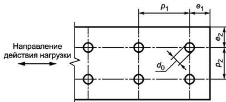
Рисунок 11.1 - Расположение метизов в соединении
