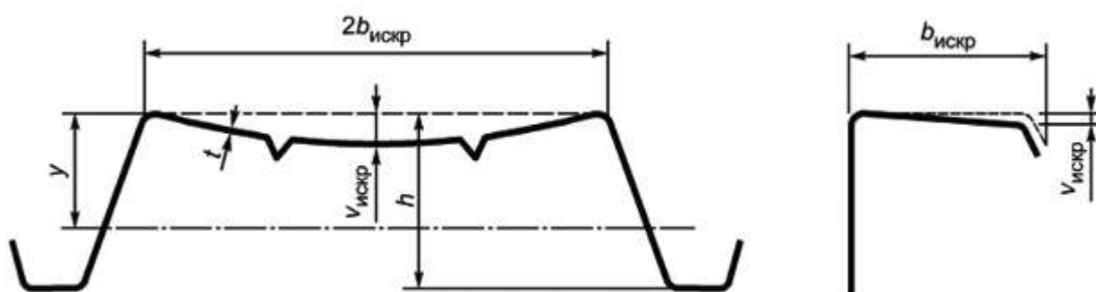
Рисунок 7.5 - Пример кривизны полки профиля, прямолинейного до приложения нагрузки
