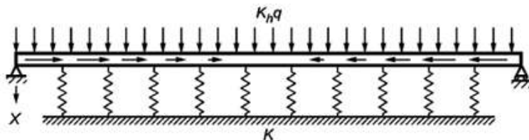
Рисунок Б.1 - Моделирование прогонов, раскрепленных настилом
