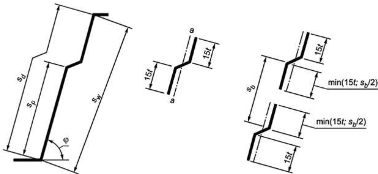
Рисунок 8.9 - Стенка с продольными элементами жесткости
