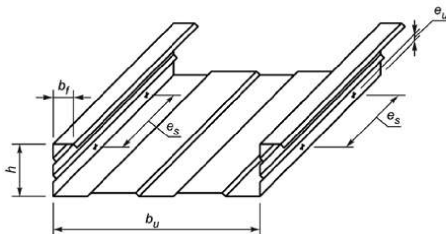
Рисунок Б.10 - Расположение метизов в продольном стыке
