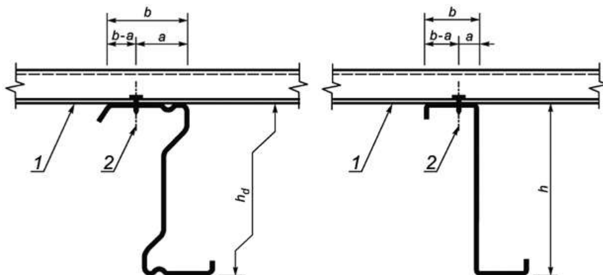
Рисунок Б.2 - Прогон и прикрепленный настил
