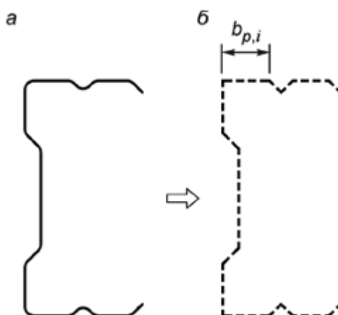
а - действительное поперечное сечение; б - идеализированное поперечное сечение
