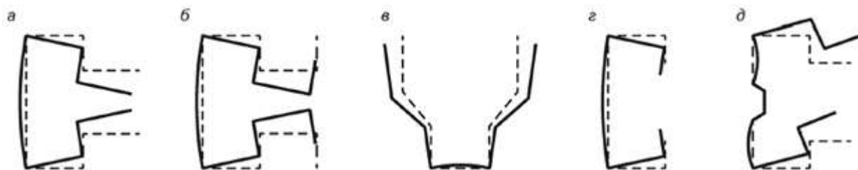
Рисунок 7.6 - Примеры потери устойчивости формы сечения
