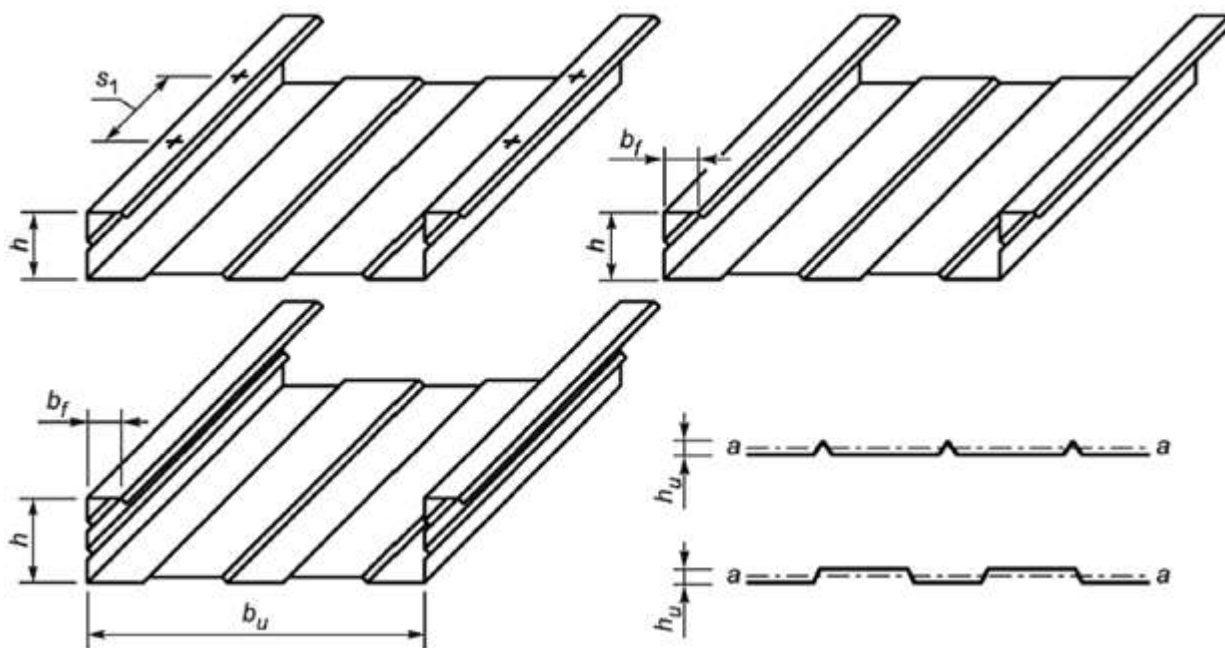
Рисунок 9.1 - Типовая геометрия кассетных профилей
