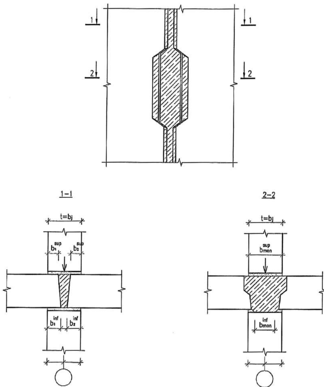
Рисунок 4.5 - Платформенно-монолитный стык сборных стен
