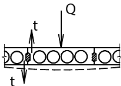
Рисунок Г.1 - Шпоночные соединения плит перекрытий
