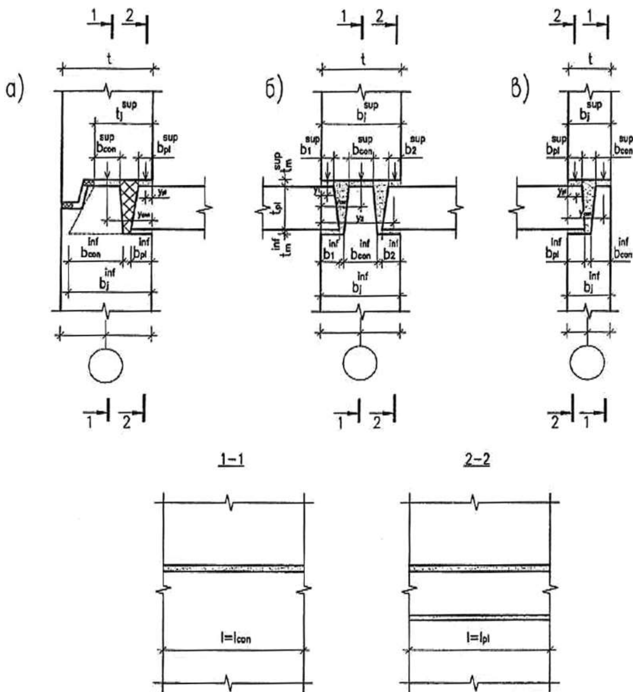
а - наружных панелей; б, в - внутренних стен
