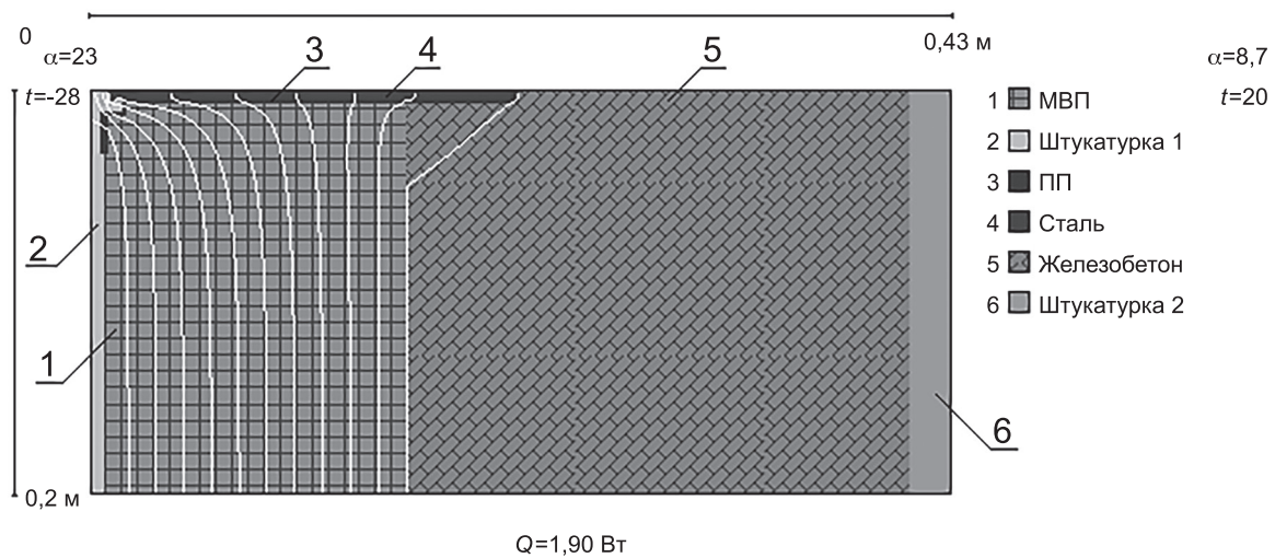
Рисунок И.4 — Температурное поле узла конструкции, содержащего точечный элемент 1
