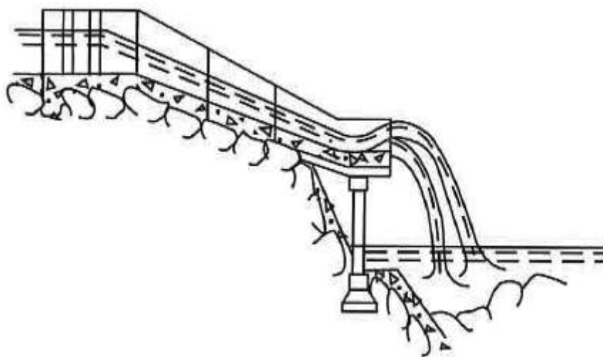
Рисунок 39 - Схема консольного сброса с концевой частью лотка в виде сплошной плиты с расщепителями, расположенной на опорах
