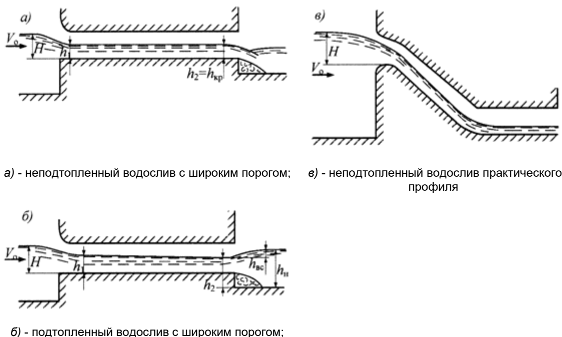
Рисунок 19 - Безнапорные закрытые водосбросы с фронтальным лобовым входом, пропускная способность которых определяется как для водослива
