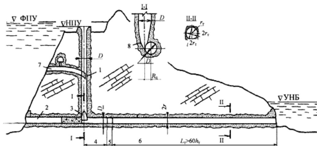
1 - шахта; 2 - строительный туннель; 3 - тангенциальный завихритель; 4 - туннель круглого сечения; 5 - переходной участок; 6 - отводящий туннель; 7 - глубинный водоприемник; 8 - цилиндрическая вставка завихрителя
