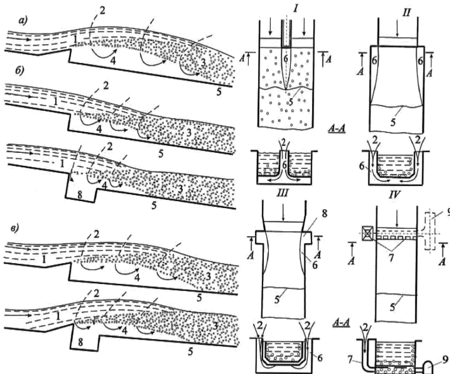
Продольные разрезы по оси аэраторов: а) - трамплинный; б) и в) - ступенчатый и комбинированный без воздухоподводящего (аэрационного) паза и с воздухоподводящим пазом на дне; Схемы подвода воздуха: I - полостная за бычком; II - полостная за ступенчатым или трамплинным отклонителем; III - с боковым воздухоподводящим пазом; IV - канальная; 1 - неаэрированный поток; 2 - подвод воздуха; 3 - водовоздушная смесь; 4 - подструйная полость; 5 - граница в конце подструйной полости; 6 - воздухоподводящая полость; 7 - воздуховод; 8 - воздухоподводящий паз; 9 - воздухоподводящая галерея
