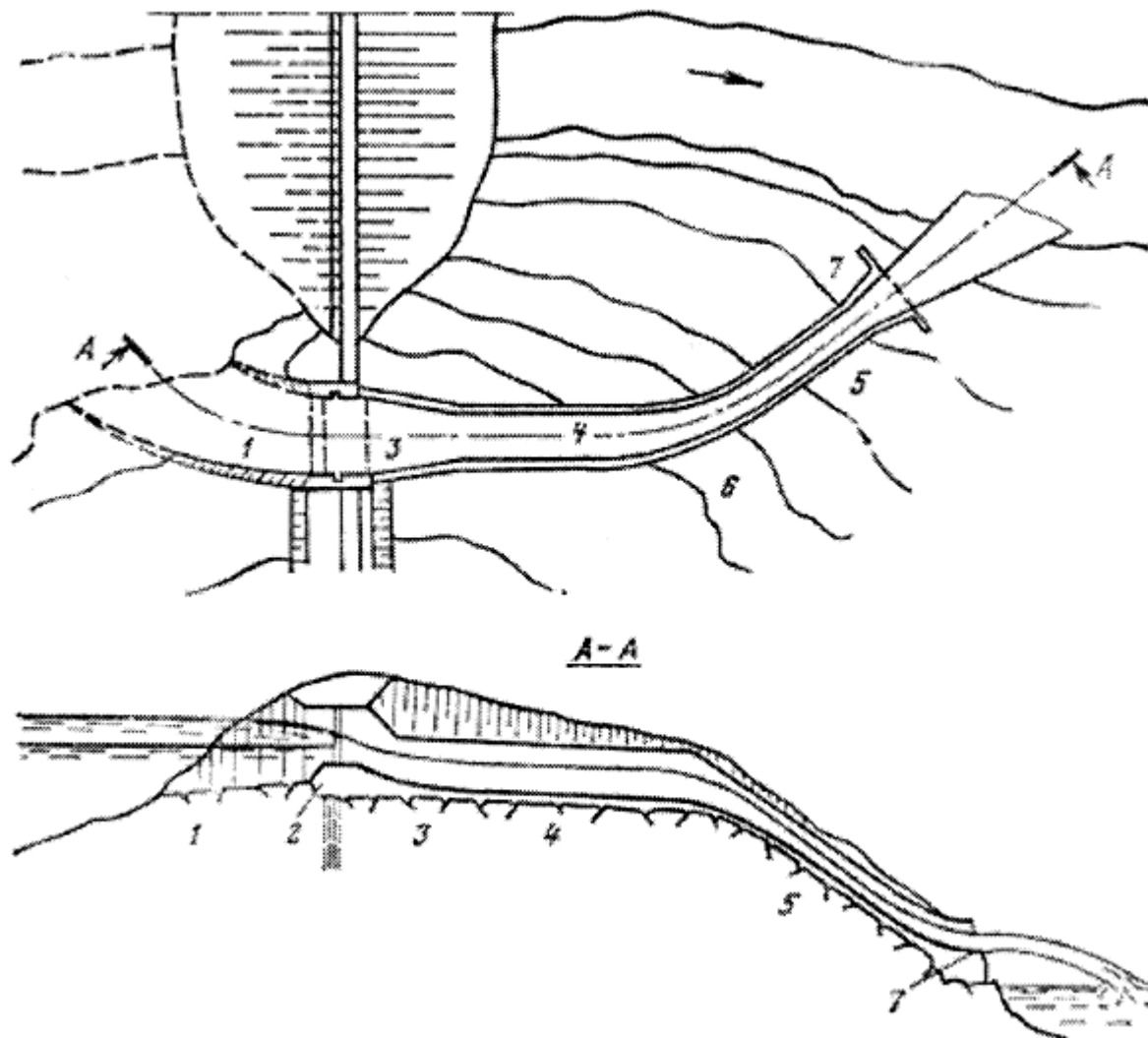
Рисунок 15 - Схема берегового поверхностного водосброса
