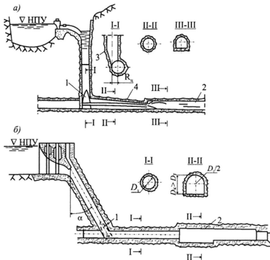
1 - тангенциальный завихритель; 2 - камера гашения; 3 - плоская вставка завихрителя; 4 - конфузорный участок
