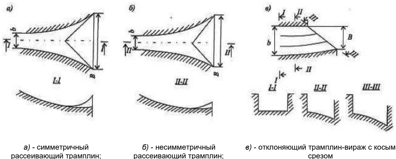
Рисунок 44 - Рассеивающие и отклоняющие трамплины с дном двойкой кривизны
