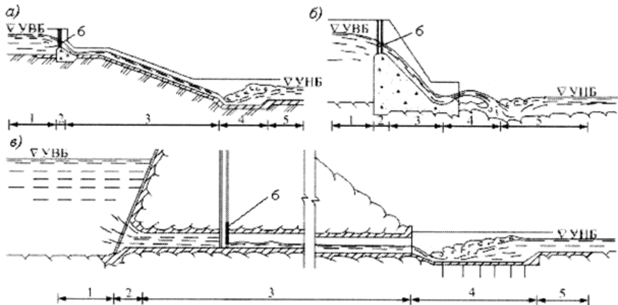
а) - открытый береговой водосброс; б) - открытый русловый водосброс в виде водосливной плотины с высоким порогом; в) - закрытый туннельный водосброс
