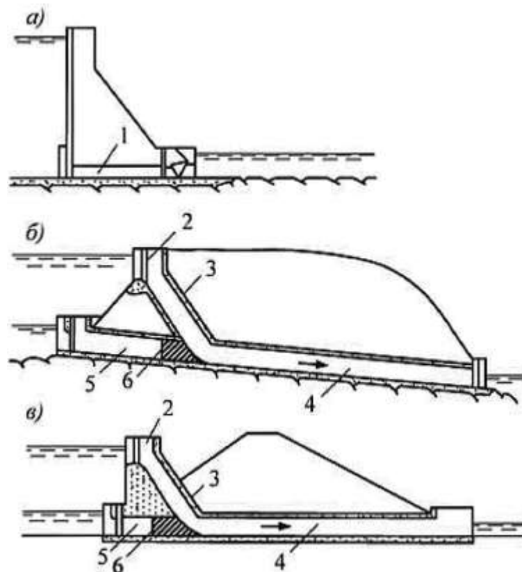
а) - донный водосброс в бетонной плотине; б) - туннельный водосброс; в) - трубчатый водосброс под грунтовой плотинной; 1 - строительно-эксплуатационный водосброс; 2 - входная часть эксплуатационного водосброса; 3 - сопрягающий участок эксплуатационного водосброса; 4 - отводящий участок; 5 - участок строительного водосброса; 6 - пробка
