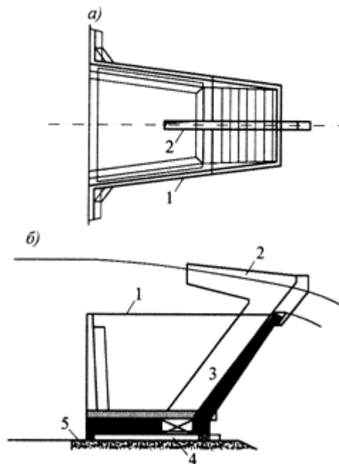
а) - план; б) - продольный разрез; 1 - гребень лабиринтного водослива; 2 - гребень водоприемника рабочей камеры; 3 - водовод рабочей камеры; 4 - рабочая камера; 5 - гребень плотины (порог затвора)
