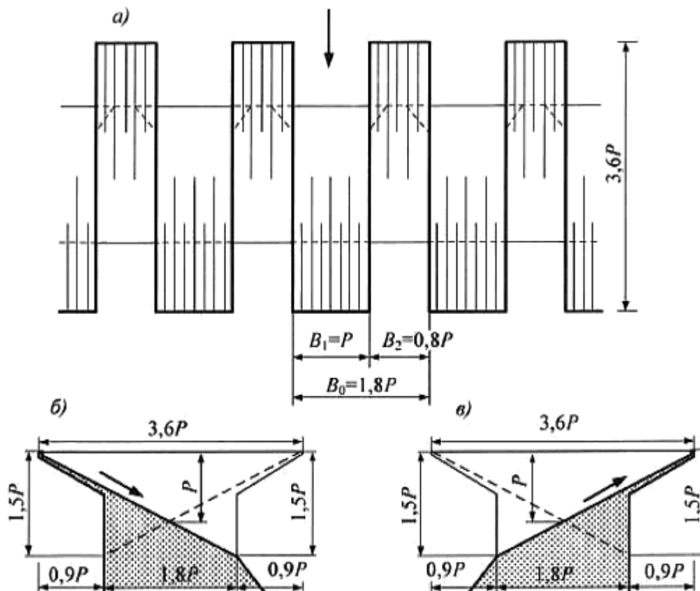
а) - план; б) - разрез по нисходящей части секции; в) - разрез по восходящей части секции
