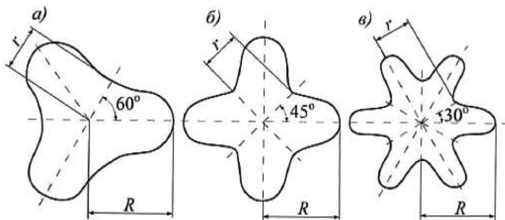
а)-в) - оголовки с тремя, четырьмя и шестью лепестками
