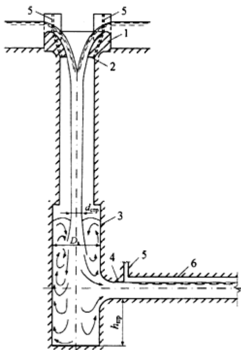
1 - кольцевая воронка; 2 - уступ для подвода воздуха; 3 - цилиндрический (шахтный) гаситель; 4 - забральная стена; 5 - воздуховоды; 6 - отводящий тракт
