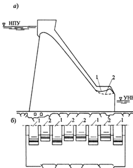
а) - разрез по плотине и б) - вид со стороны нижнего бьефа; 1 и 2 - носки-трамплины с меньшими и большими углами на сходе, обеспечивающими различную дальность отброса потока
