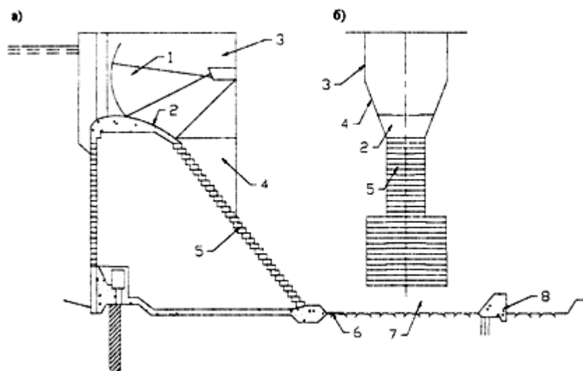
а) - продольный разрез; б) - вид на водосливной пролет с нижнего бьефа; 1 - сегментный затвор; 2 - водосливной оголовок безвакуумного профиля из вибрированного бетона; 3 - бык; 4 - сужение пролета; 5 - сборные элементы сливной грани; 6 - крепление; 7 - водобойный колодец; 8 - водобойная стенка
