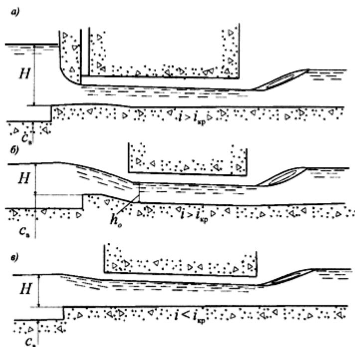
а) - с забральной стенкой; б) - с водосливным порогом; в) - в виде водослива без порога
