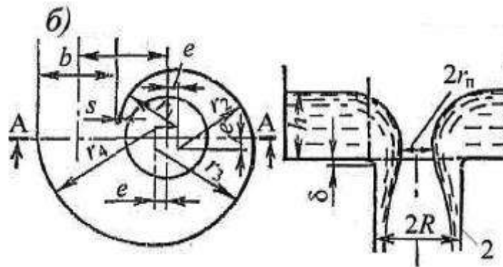
б) - завихритель в виде спиральной камеры;
