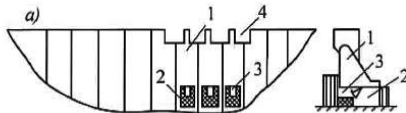
а) - плотина с эксплуатационными поверхностными водосбросами;
