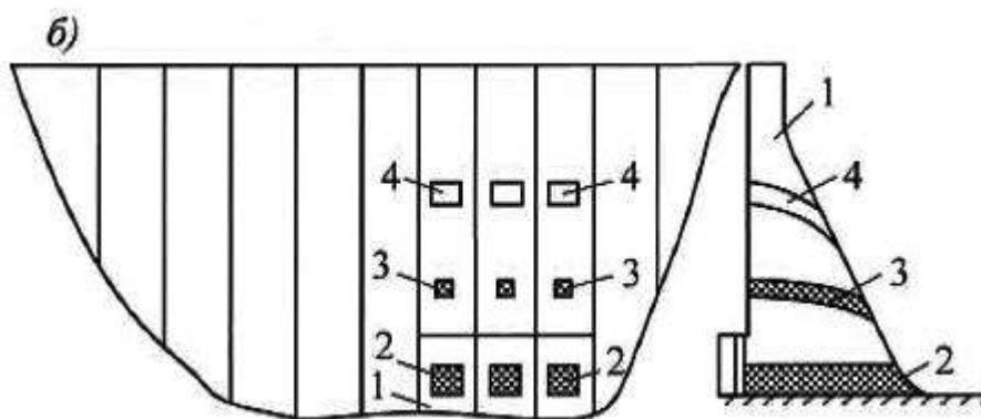
б) - плотина с эксплуатационными глубинными водосбросами;
