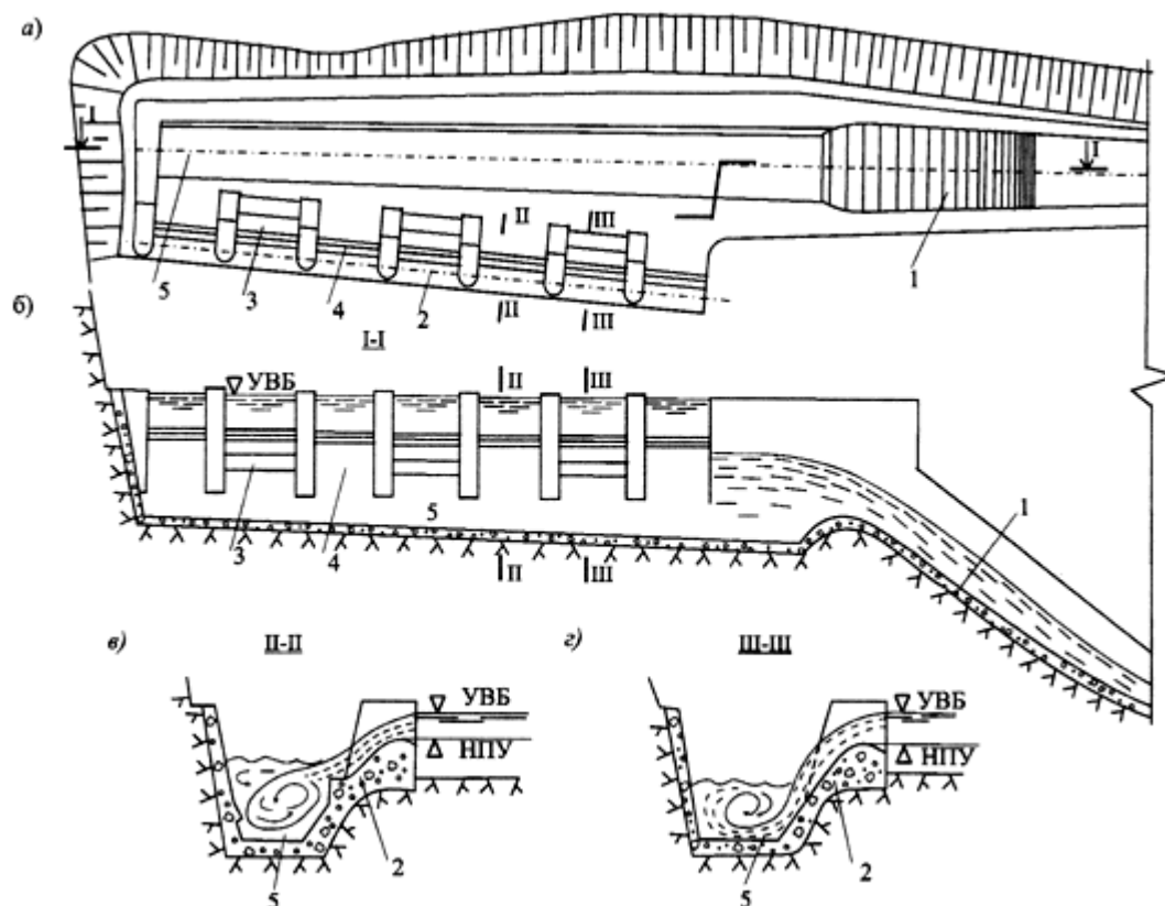
а) - план; б) - вид на боковой водослив со стороны водосбросной траншеи; в) и г) - поперечные разрезы по пролетам бокового водослива, соответственно, с носками и без носков на сливной грани; 1 - быстроток; 2 - боковой водослив; 3 - пролеты бокового водослива с носками на сливной грани; 4 - пролеты без носков; 5 - водосбросная траншея
