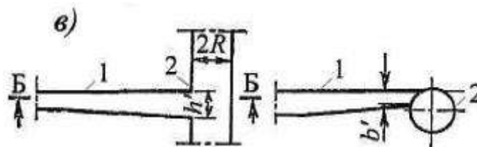
в) - завихритель с тангенциальным подводом к шахте;
