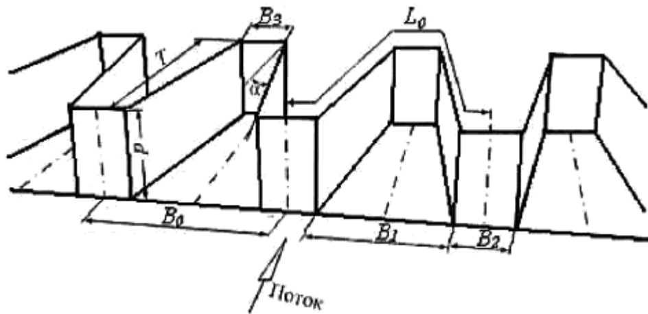
Рисунок 13 - Схема лабиринтного водослива
