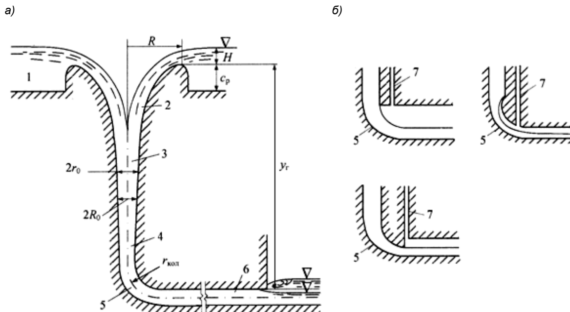
Рисунок 20 - Схема шахтного водосброса с кольцевой водосливной воронкой (а) и ряд схем конструкции, сопрягающей его шахту с отводящим трактом (б)
