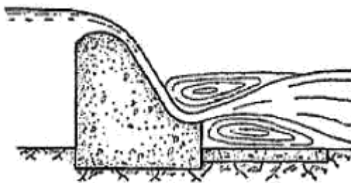
Рисунок 6 - Водосливная плотина с уступом
