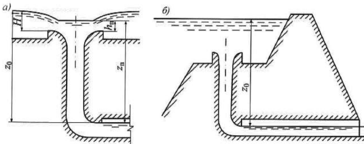
а) - с подтопленной и б) - затопленной водосливной воронкой
