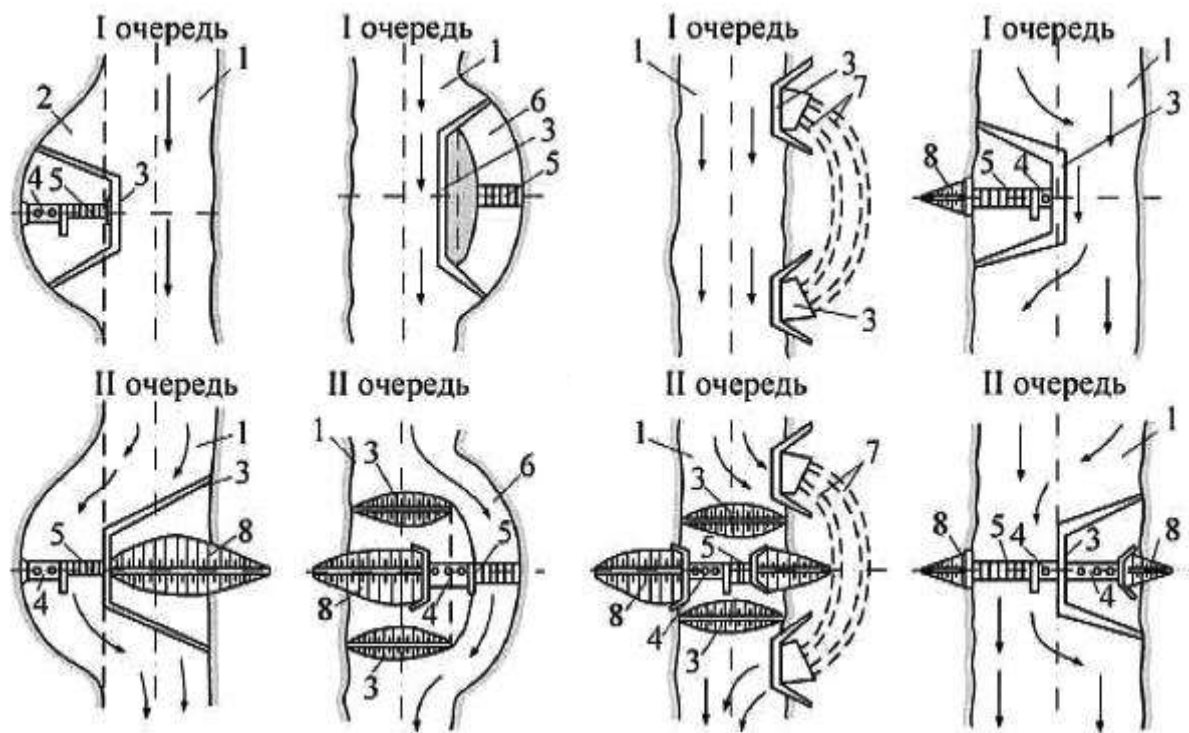
1 - русло реки; 2 - пойменная выемка; 3 - перемычки; 4 - здание ГЭС; 5 - водосброс; 6 - канал; 7 - туннели (или трубы); 8 - глухая плотина
