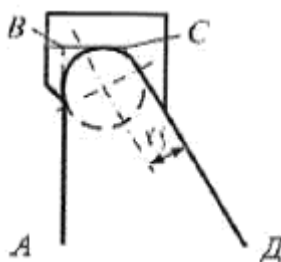
Рисунок 3 - Схема вакуумного водосливного оголовка
