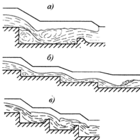
Рисунок 17 - Схемы перепадов
