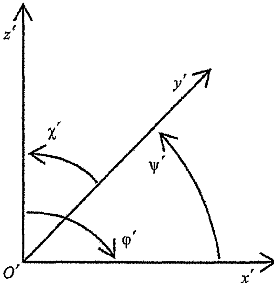
Рисунок Б.1 – Степени свободы фундамента
