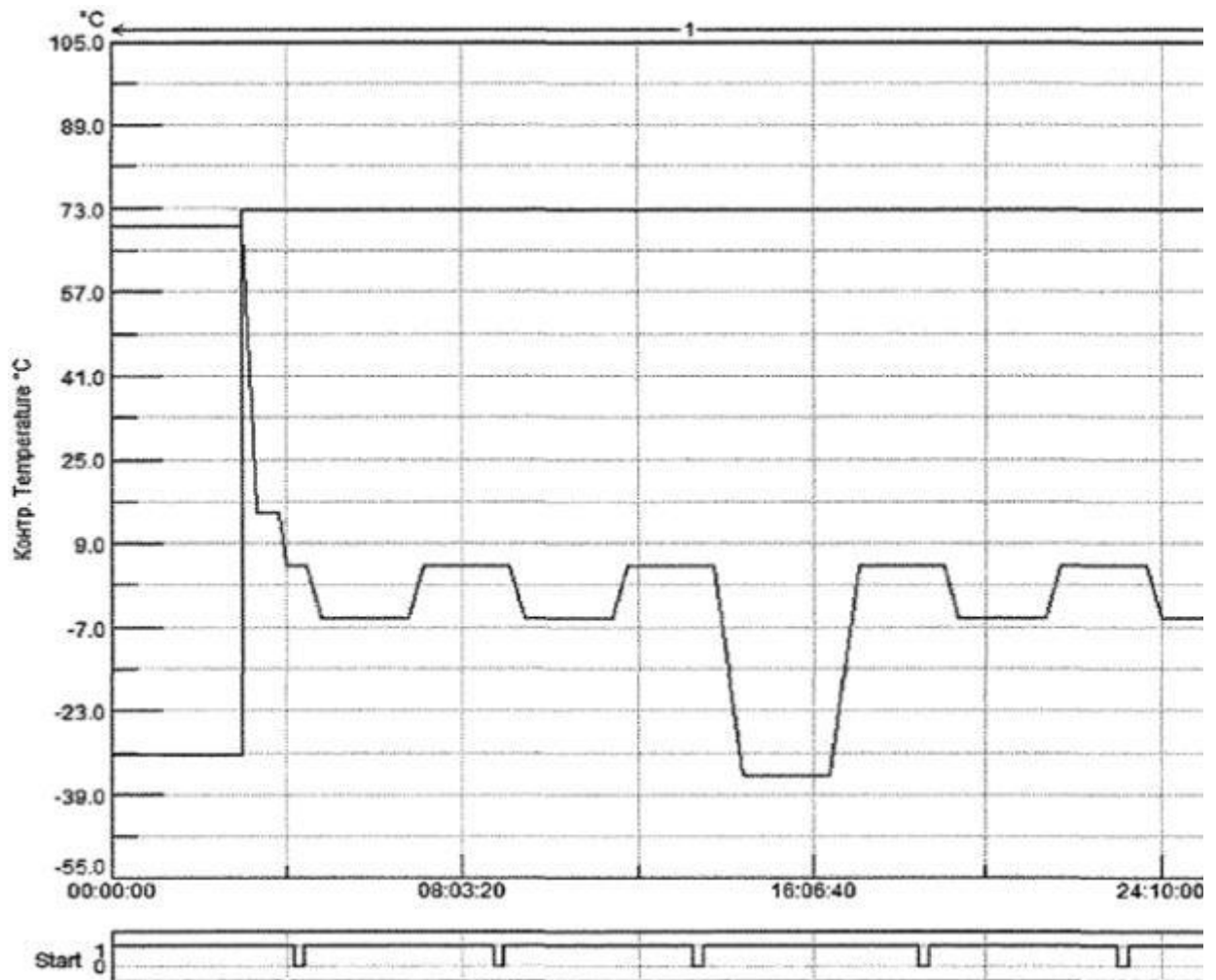
Рисунок А.1 - Графическая модель одного цикла климатических испытаний
