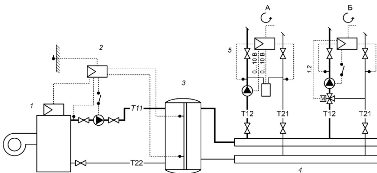
1 - котельная установка; 2 - контроллер управления источника 1; 3 - буферная емкость теплоносителя; 4 - распределительный коллектор; 5 - контур теплоснабжения: А - жилых помещений, Б - мест общего пользования
