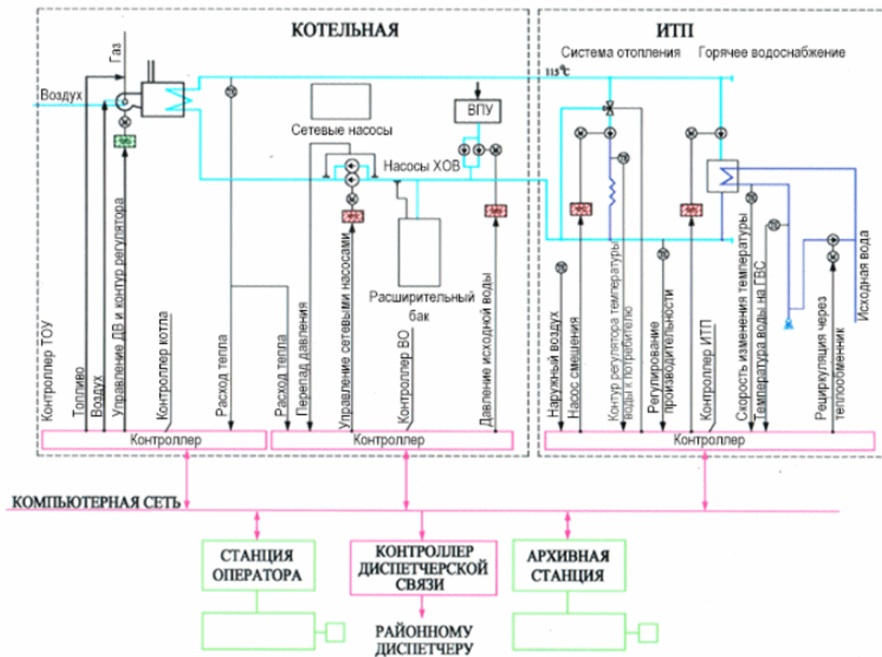
Рисунок 5.1 - Комплексная автоматизированная система управления теплоснабжения жилого района при количественно-качественном регулировании
