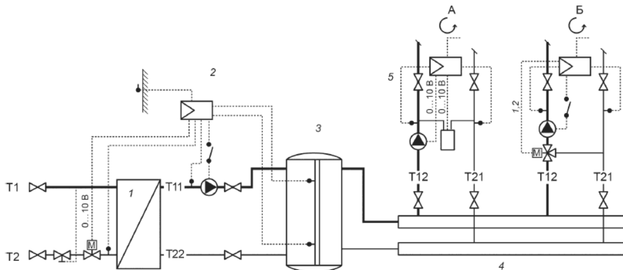
1 - сетевой теплообменник; 2 - контроллер управления источника 1; 3 - буферная емкость теплоносителя; 4 - распределительный коллектор; 5 - контур теплоснабжения: А - жилых помещений, Б - мест общего пользования
