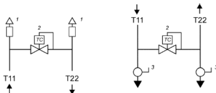
а) - верхний мост циркуляции б) - нижний мост циркуляции
