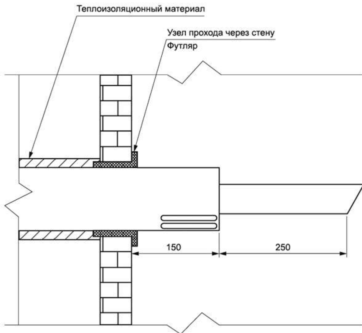
Рисунок А.1 - Конструкция оголовка индивидуальной коаксиальной системы дымоудаления Таблица А.1 - Расчет температур продуктов сгорания для температуры уходящих газов 80°C для теплогенераторов с немодулируемыми вентиляторами
