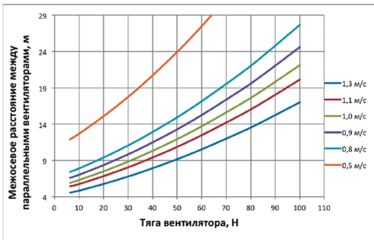
Рисунок И.2 - График зависимости межосевого расстояния b от расчетной реактивной тяги
