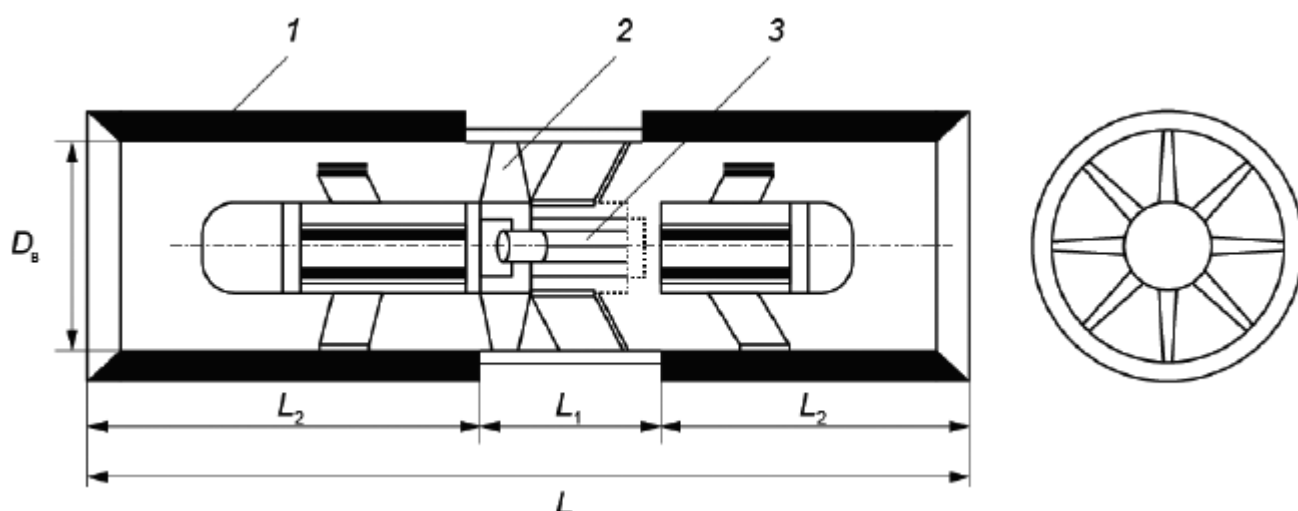
L - общая длина струйного вентилятора; L_1 - длина осевого реверсивного вентилятора с двигателем; L_2 - длина глушителя; 1 - шумоглушитель; 2 - лопадки; 3 - двигатель
