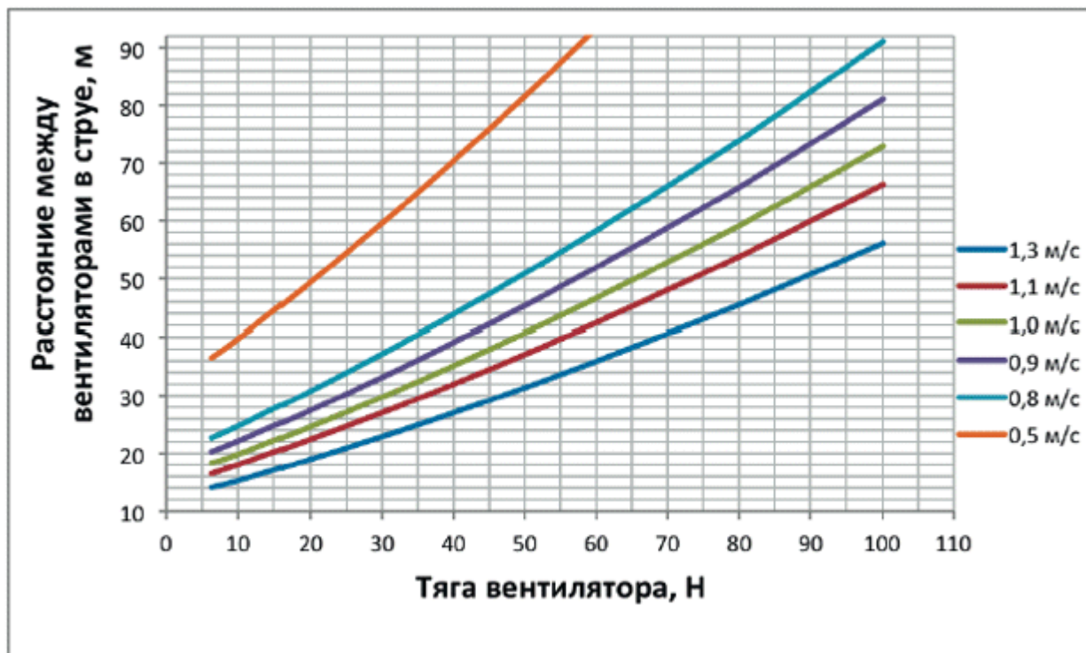
Рисунок И.1 - График зависимости расстояния L_{\text{ш}} (в струе) от расчетной реактивной тяги F_p вентилятора при различных значениях v_{x \min}
