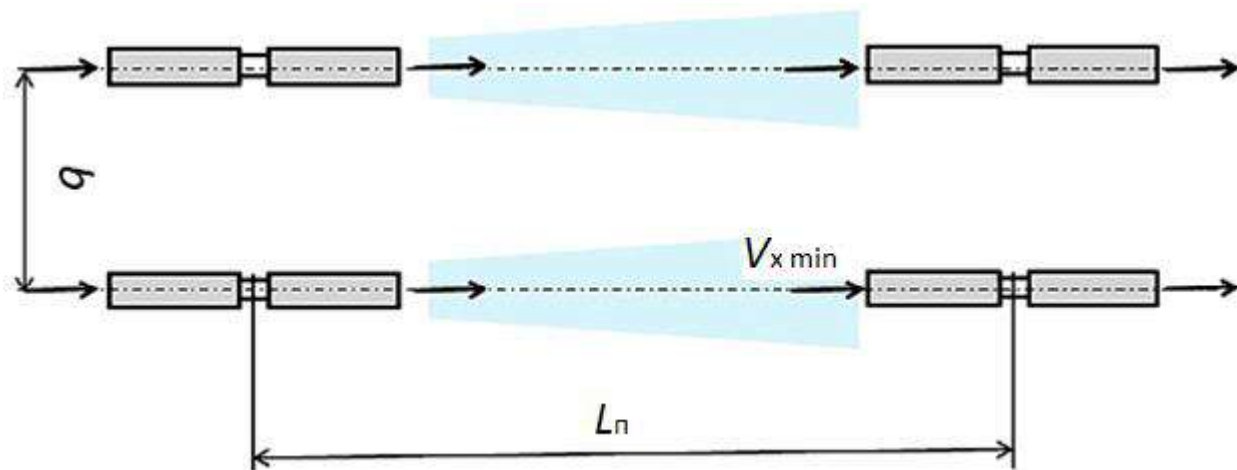
а) Соосная установка струйных вентиляторов
