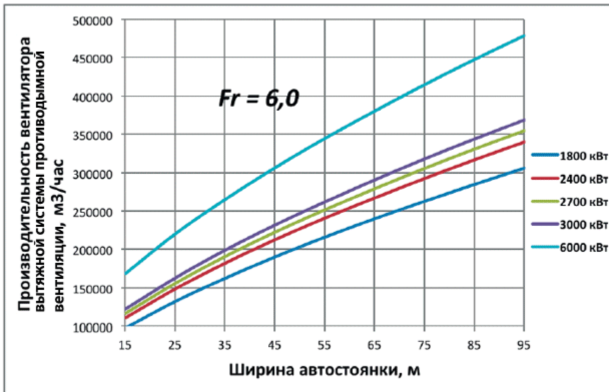
Рисунок Е.3* - График зависимости производительности вентиляторов вытяжной системы противодымной вентиляции
