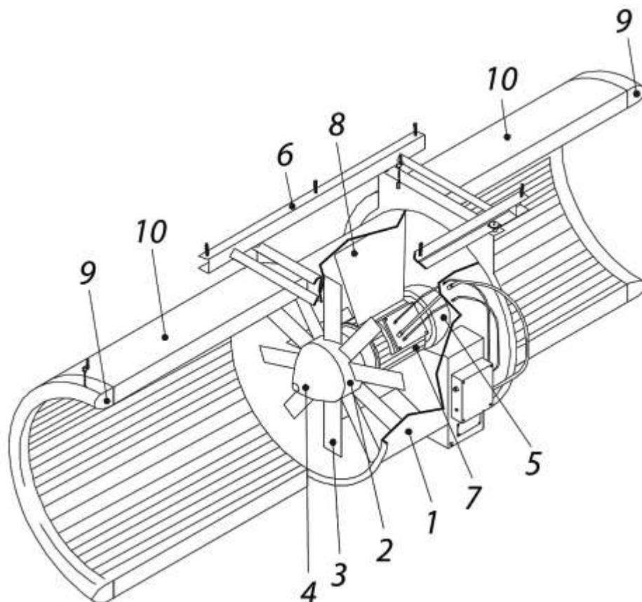
1 - корпус вентилятора; 2 - крыльчатка; 3 - лопасть крыльчатки; 4 - носовой обтекатель; 5 - хвостовой обтекатель; 6 - монтажная рама; 7 - электродвигатель; 8 - опора двигателя; 9 - наконечник; 10 - шумоглушитель
