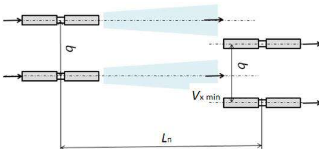
б) Параллельная установка струйных вентиляторов
