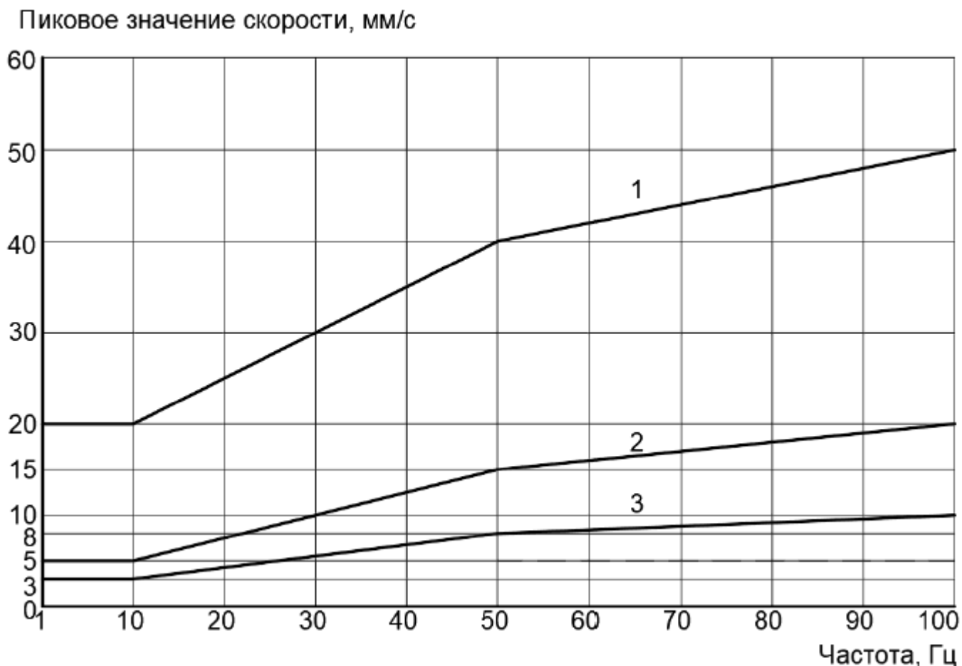
Рисунок 4.1 - Пиковые значения виброскорости колебаний
