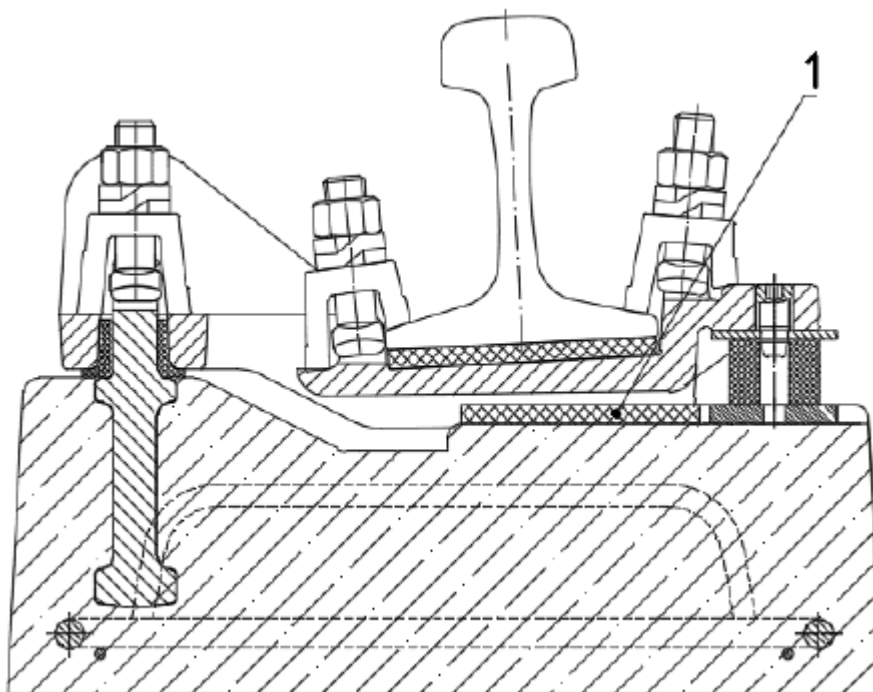
Рисунок В.4 - Специальное виброзащитное рельсовое скрепление типа ВГС5-65
