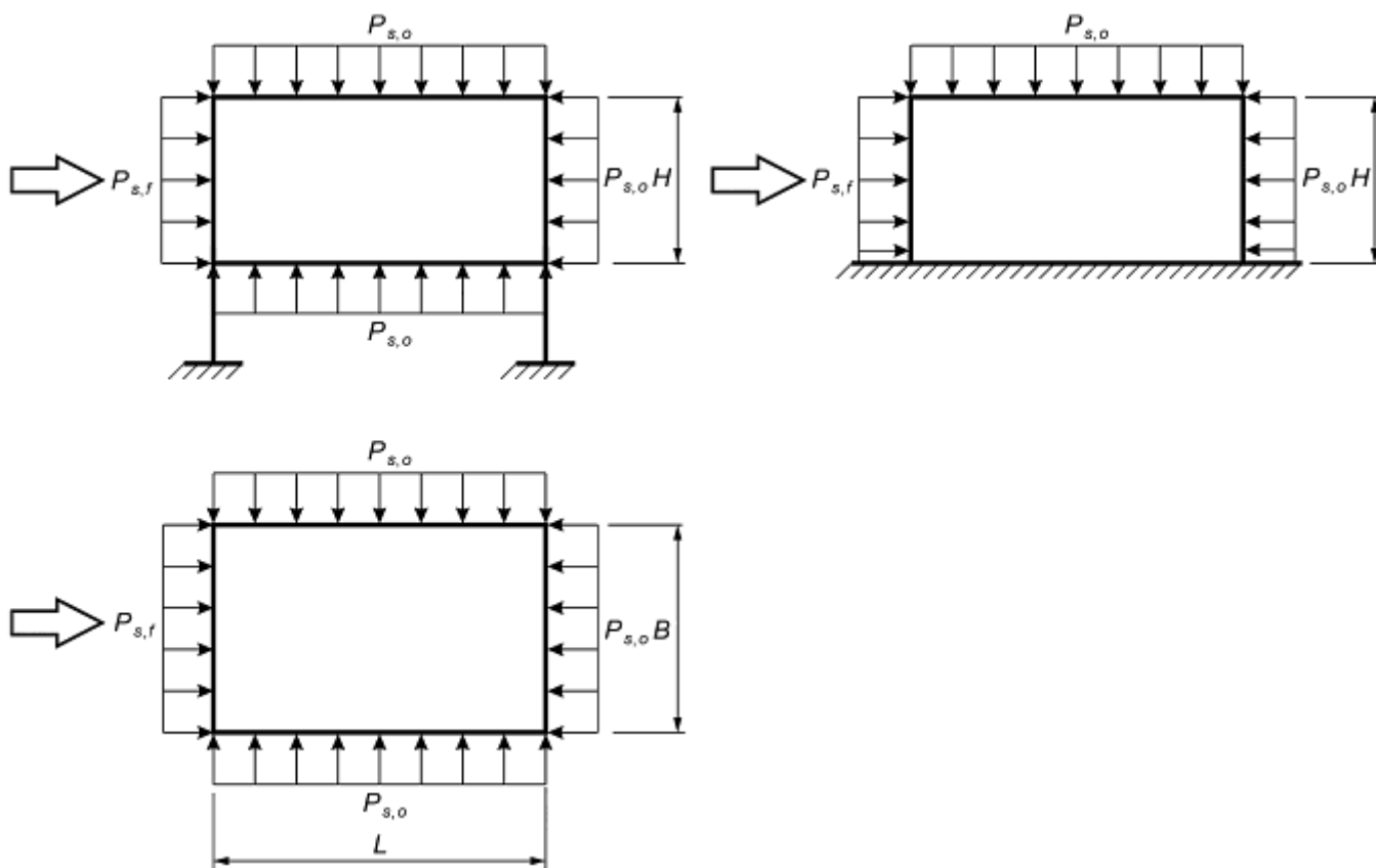
Рисунок 7.1 - Направления действия взрывных воздействий
