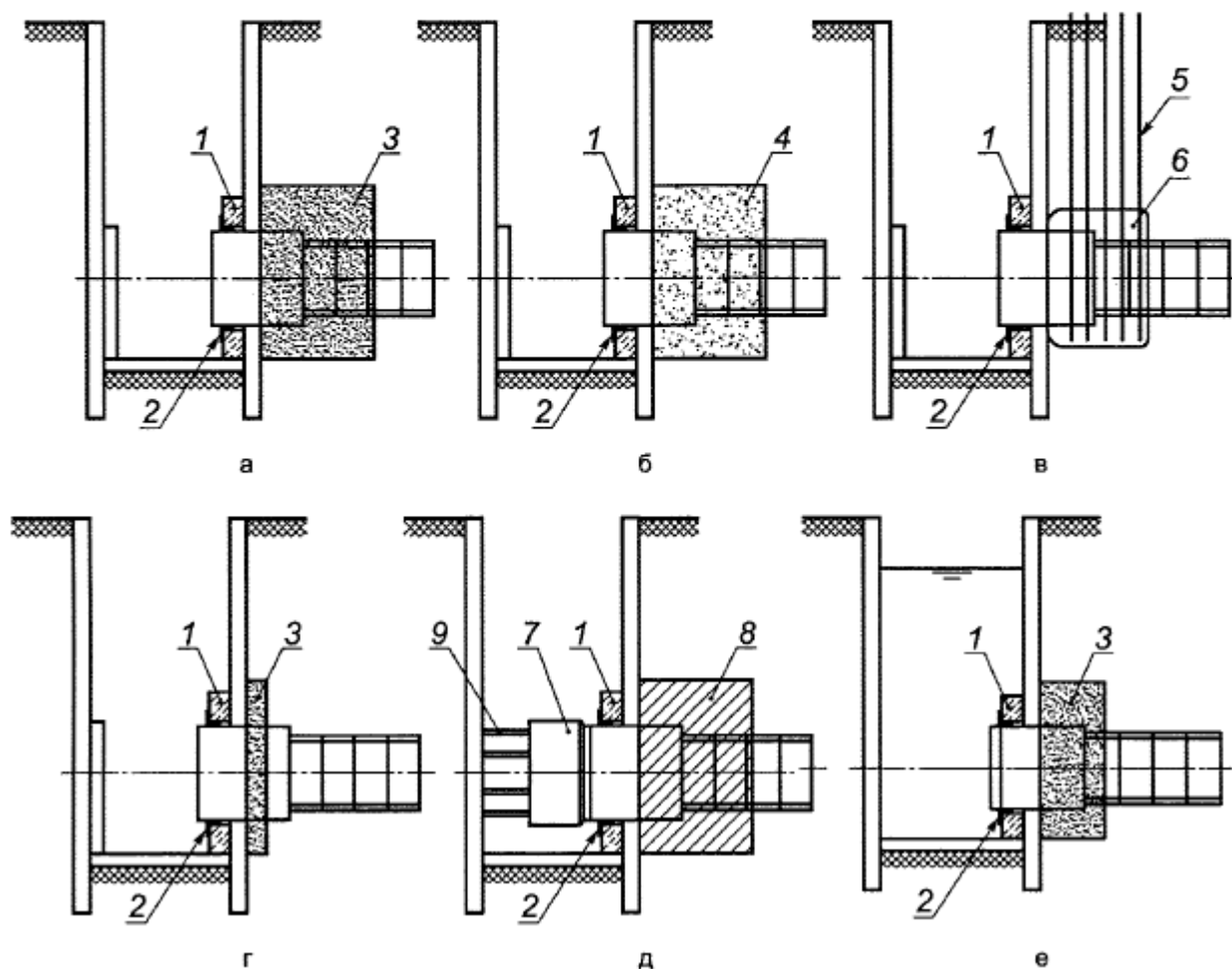
а - метод химического закрепления грунта; б - метод струйной цементации; в - метод замораживания грунтов; г - метод вырезания стенки; д - метод перемычки в шахте; е - плавающий метод; 1 - бетонное обрамление выхода; 2 - выходное уплотнение; 3 - закрепленная зона; 4 - зона замещенного грунта; 5 - замораживающие трубы; 6 - зона замороженного грунта; 7 - входная рама; 8 - глинистая паста; 9 - опора
