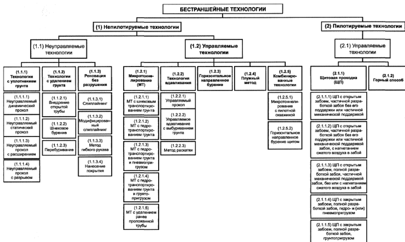
Рисунок Г.1 - Схема классификации бестраншейных технологий
