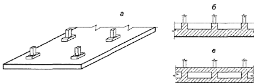
а - плитный безбалочный; б - плитно-балочный; в - коробчатый
