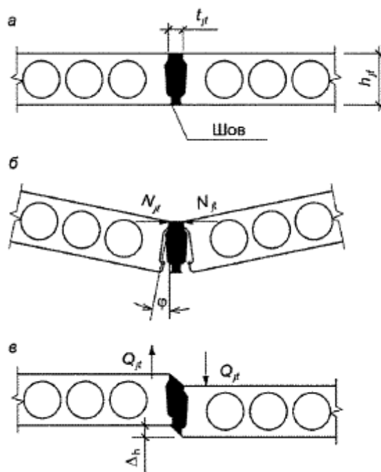
а - схема межплитного шва; б - поворот вдоль продольной оси; в - сдвиг плит
