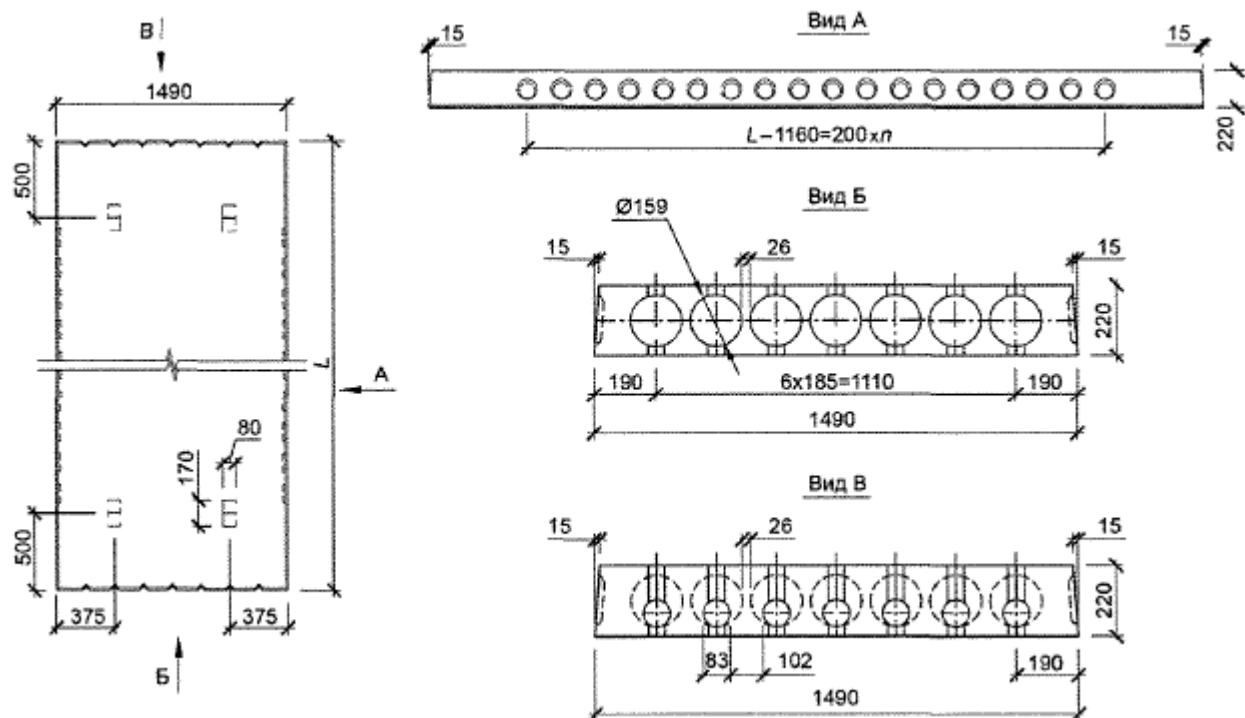
Рисунок 7.27 - Опалубочный чертеж рядовой многопустотной плиты размерами 5,65x1,49 м
