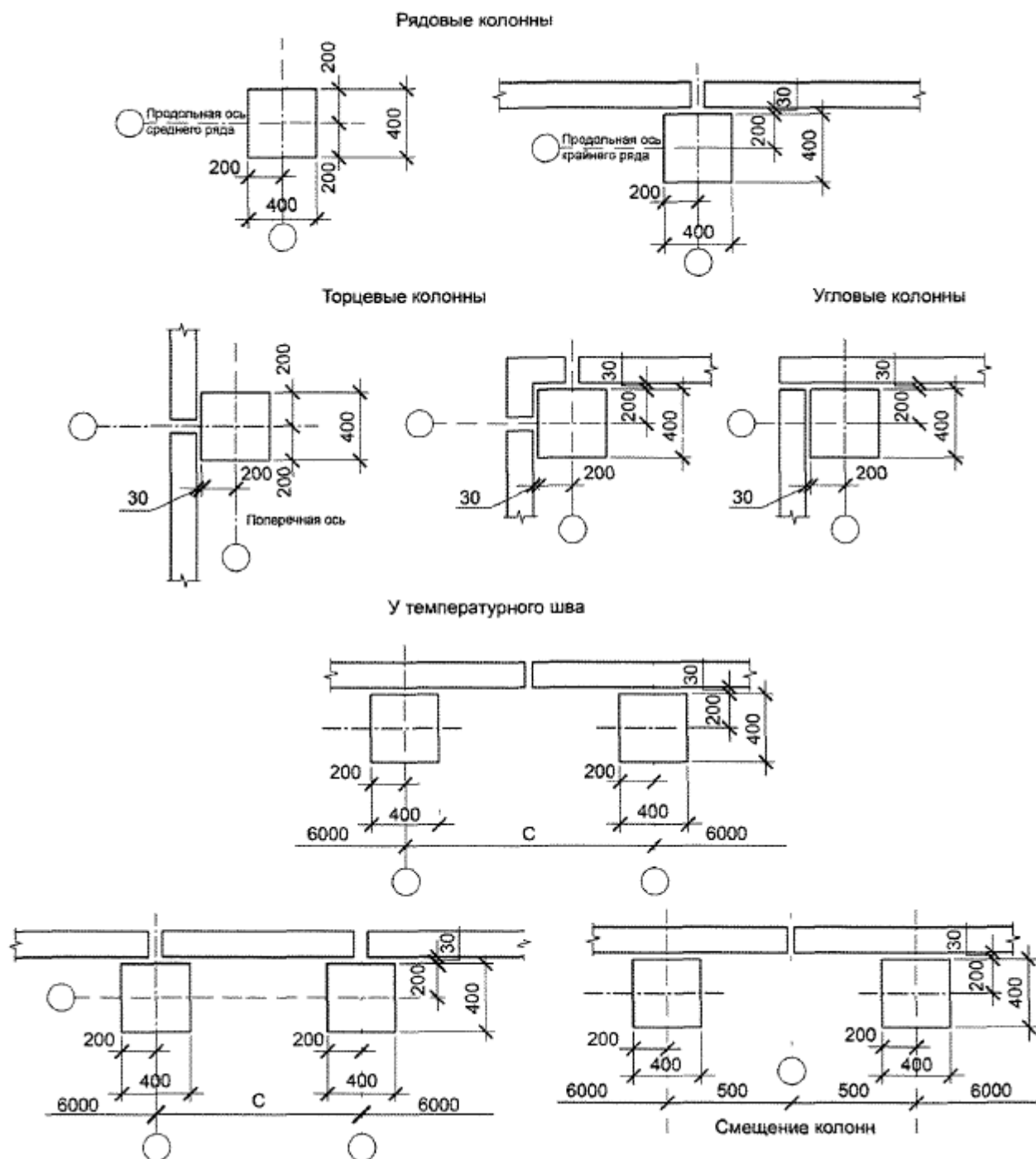
Рисунок 5.1 - Привязка конструкций к координационным осям здания
