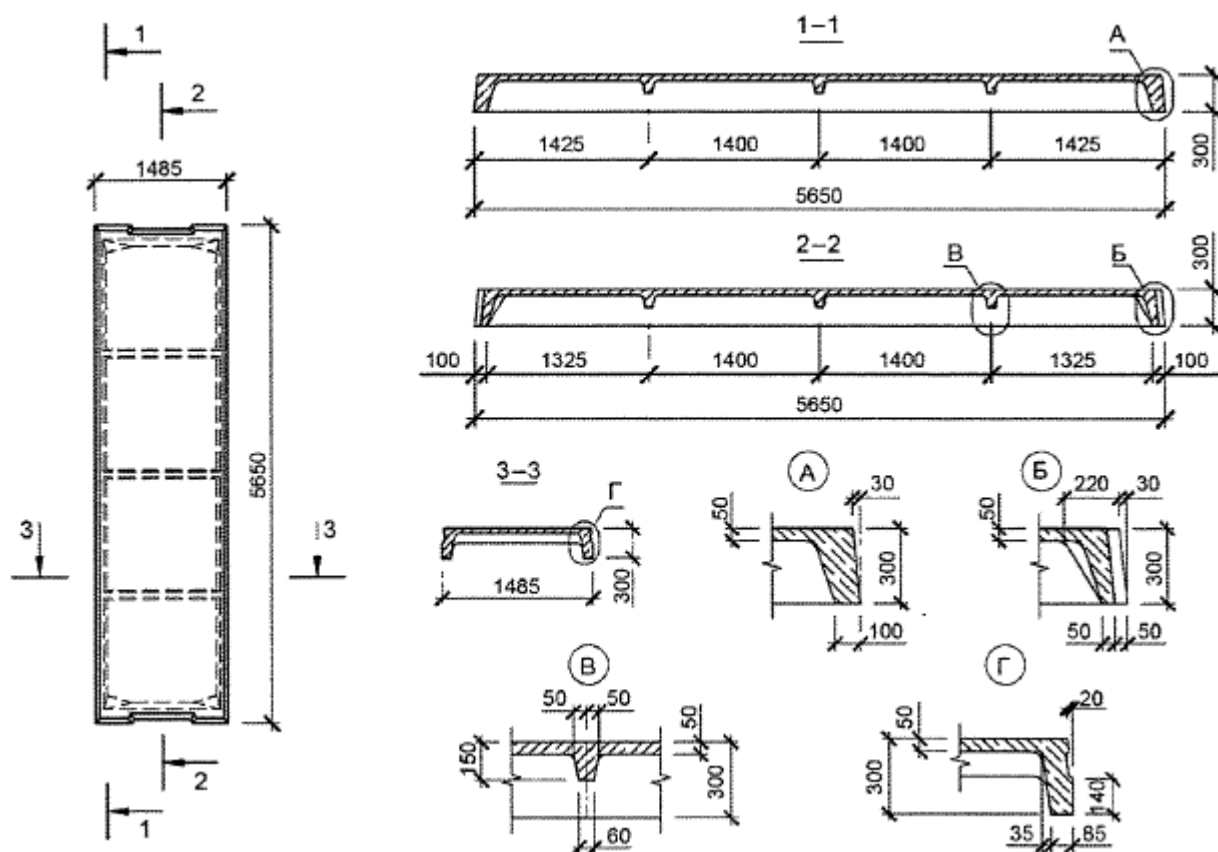
Рисунок 7.25 - Опалубочный чертеж ребристой плиты размерами 5,65x1,485 м
