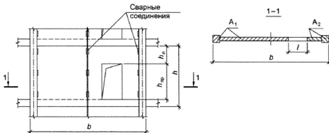
Рисунок 6.4 - Сборная железобетонная диафрагма жесткости
