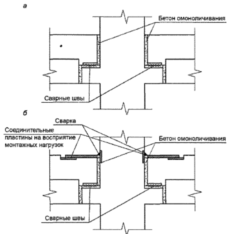
а - сопряжение ригеля с колонной со скрытой прямоугольной консолью; б - сопряжение ригеля с колонной со скрытой консолью и верхней монтажной соединительной пластиной
