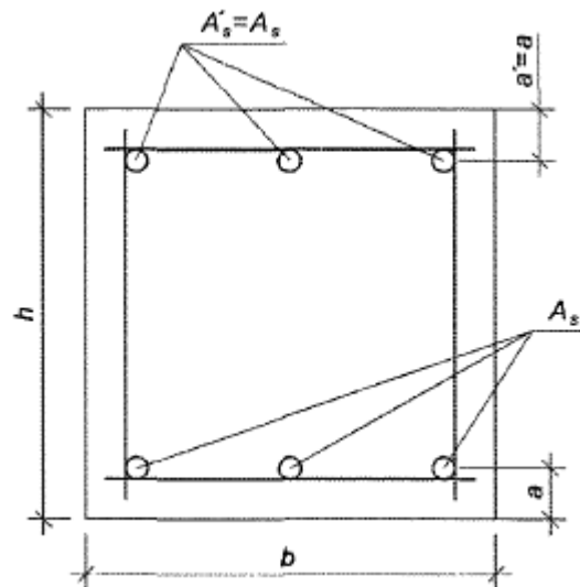
Рисунок 7.10 - Сечение с сосредоточенной симметричной арматурой
