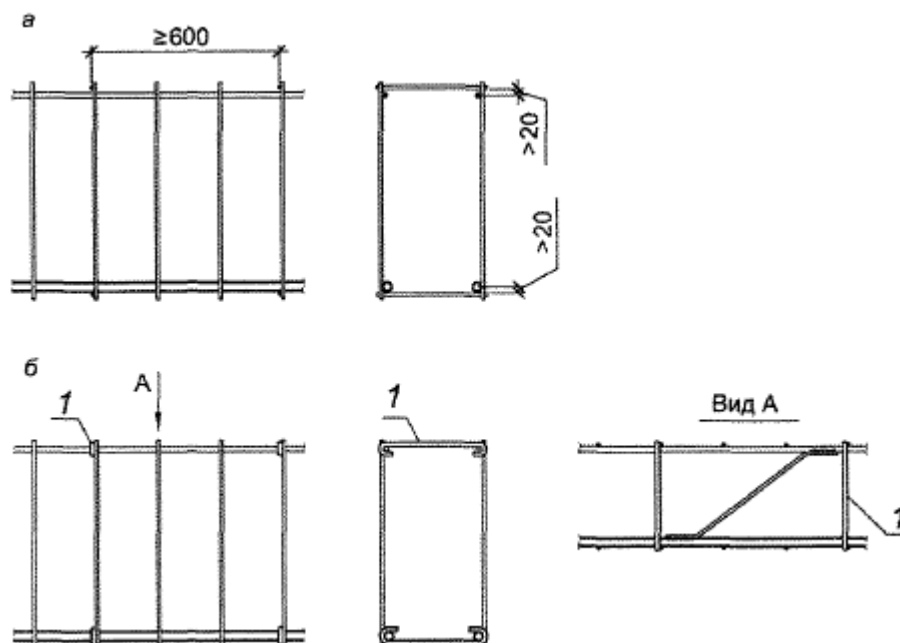
а - пространственный арматурный каркас при соединительных стержнях, привариваемых к вертикальным стержням; б - пространственный арматурный каркас при шпильках, привязываемых к продольным стержням; 1 - шпилька (соединительный стержень)
