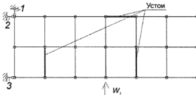
1 - опора, препятствующая поступательному смещению перекрытия; 2, 3 - опоры, препятствующие повороту перекрытия
