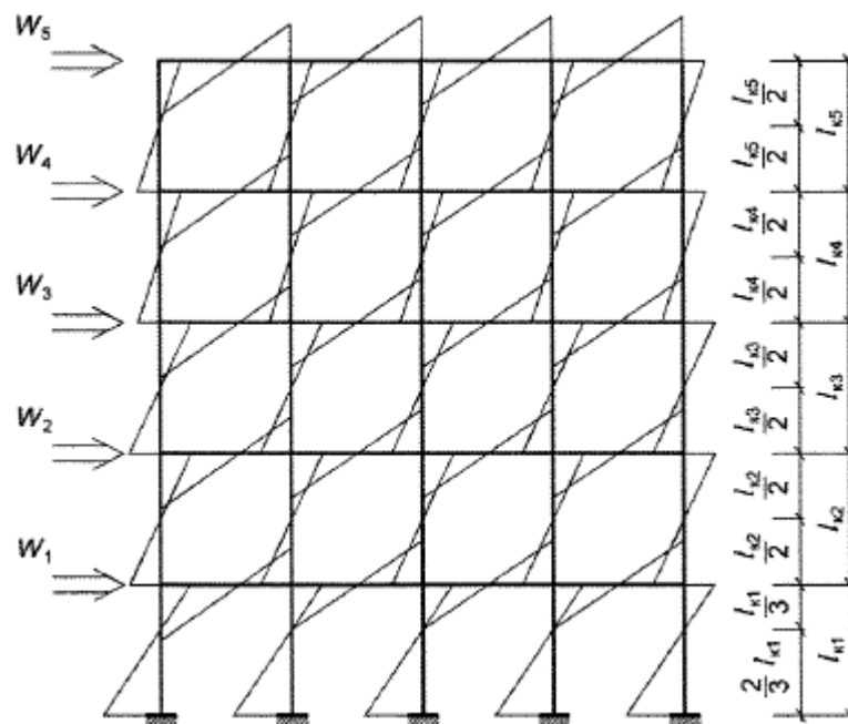
Рисунок А.2 - К упрощенному способу определения усилий
