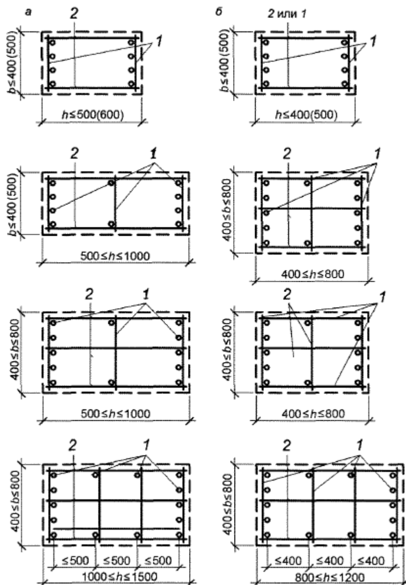
а - колонны, внецентренно сжатых в одной плоскости; б - колонны, внецентренно сжатые в обеих плоскостях; 1 - плоский каркас; 2 - соединительный стержень (поперечный привариваемый стержень или шпилька)
