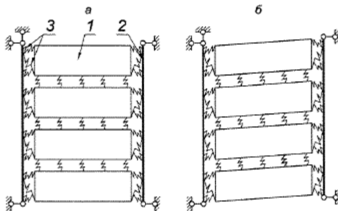
а - расчетная модель ячейки перекрытия; б - схемы деформирования при наличии связей
