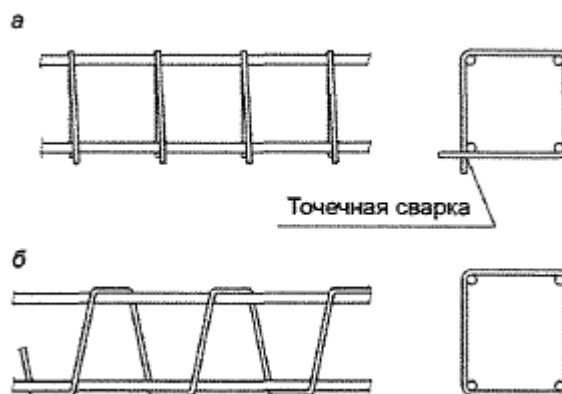
а - из ранее согнутых и сваренных хомутов; б - со спиральной арматурой
