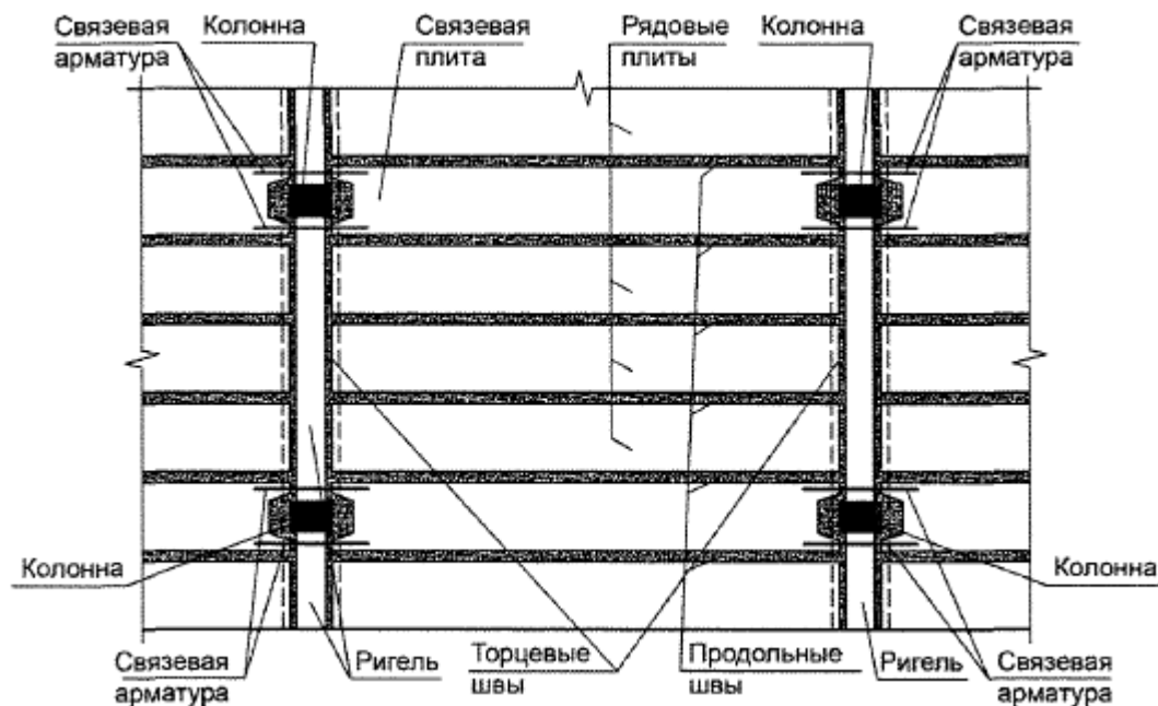
Рисунок 6.5 - Фрагмент сборного перекрытия из многопустотных плит
