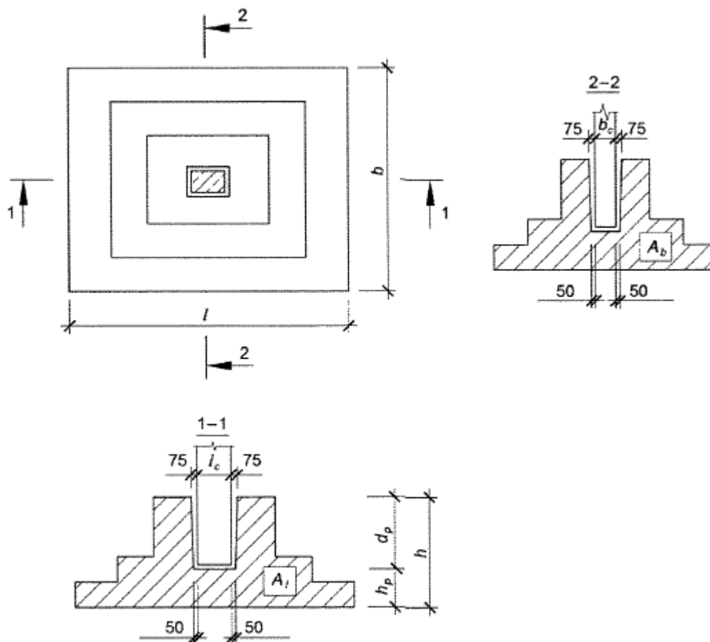
Рисунок 7.4 - К расчету фундамента стаканного типа на раскалывание
