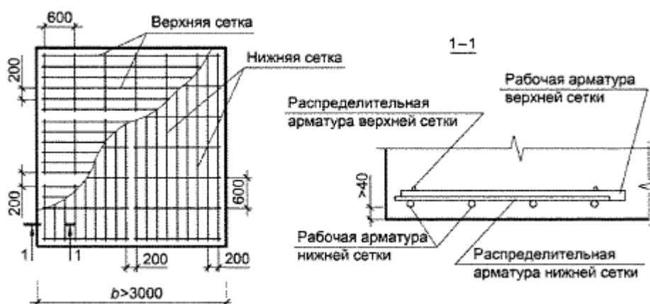
Рисунок 7.6 - Армирование подошвы фундамента сетками
