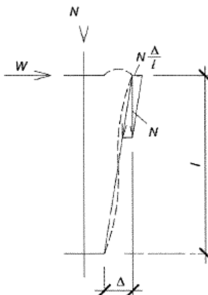
Рисунок А.8 - К учету деформированной схемы с помощью отклоняющих сил
