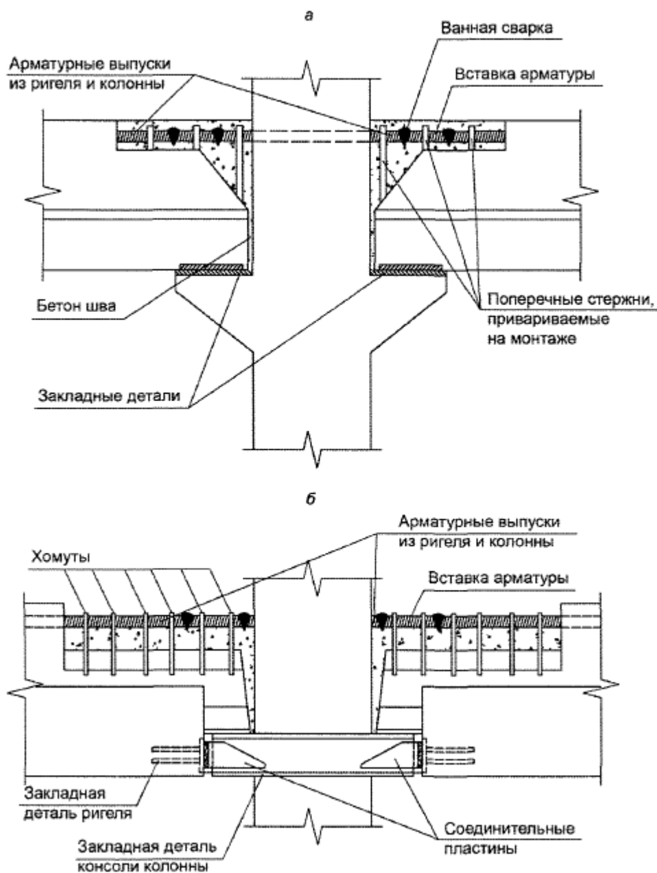
а - с опиранием на открытую консоль; б - с опиранием на скрытую консоль
