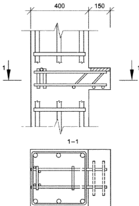
Рисунок 7.20 - Армирование консоли колонн при шарнирном опирании ригеля
