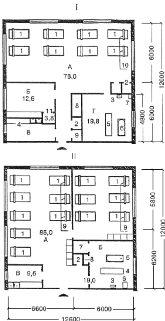
Рисунок Г.5 - Жилые ячейки для умственно отсталых детей
